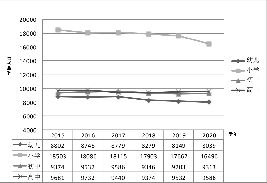
图 1 龙泉市幼儿适龄儿童和中小学学龄人口的预测
