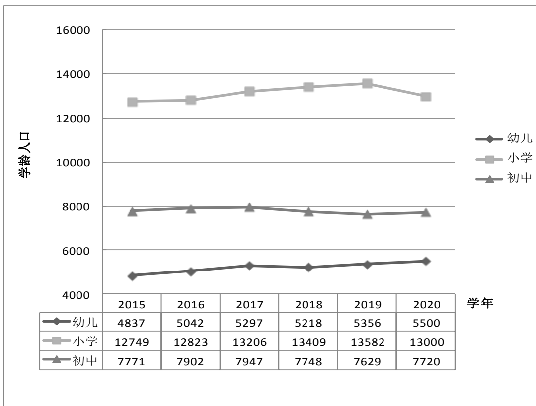
图 2 龙泉市城区幼儿和学龄人口的预测
