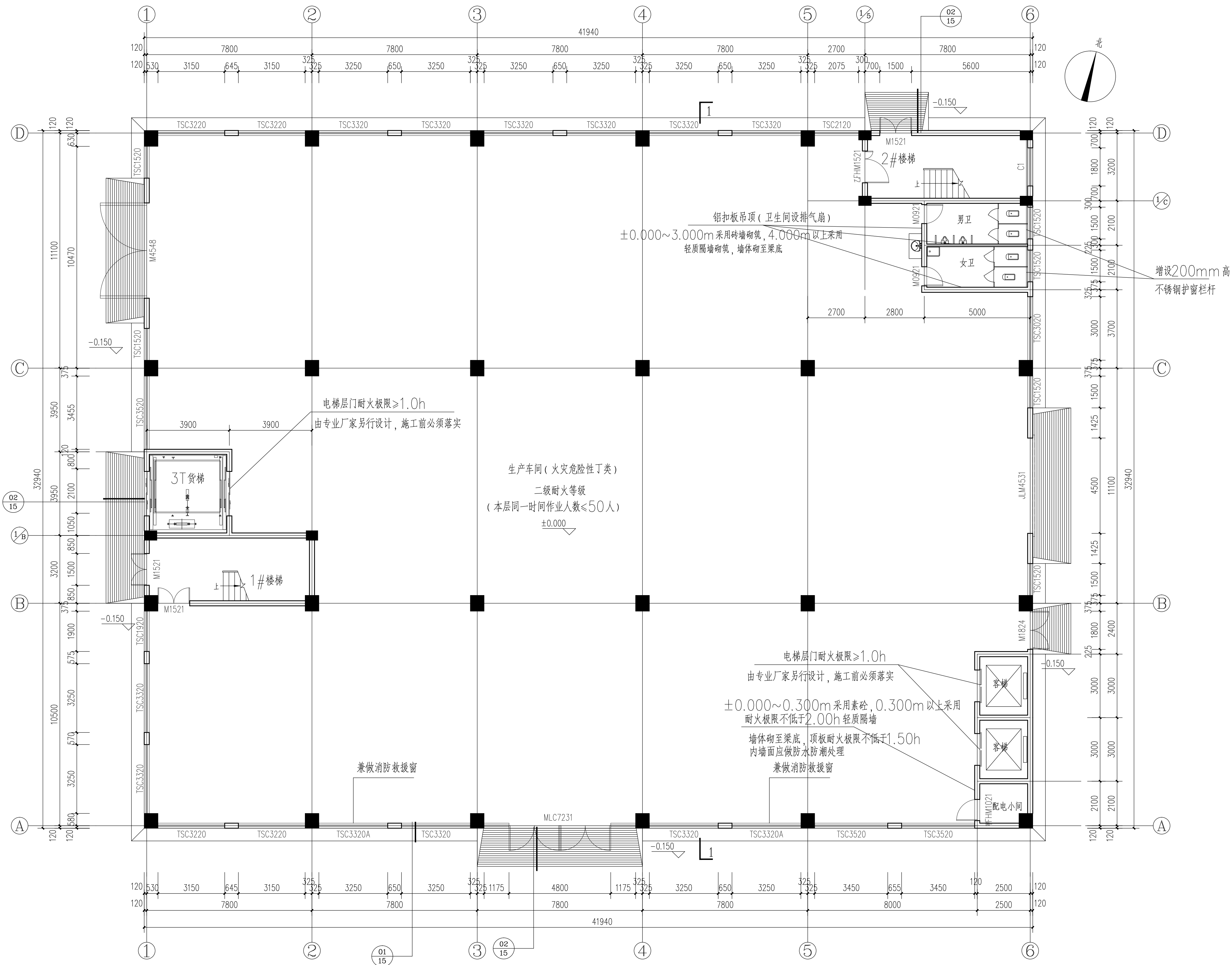
一层平面图 1:100
