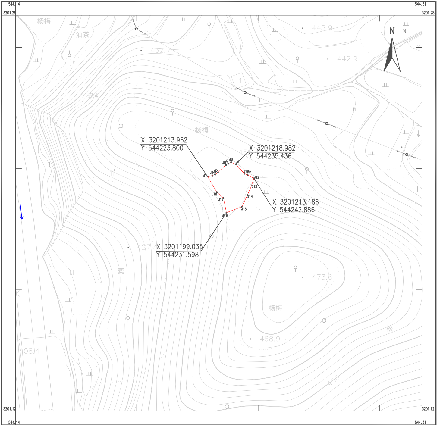
磐安移动节点机房建设双峰乡1号地块选址位置图
