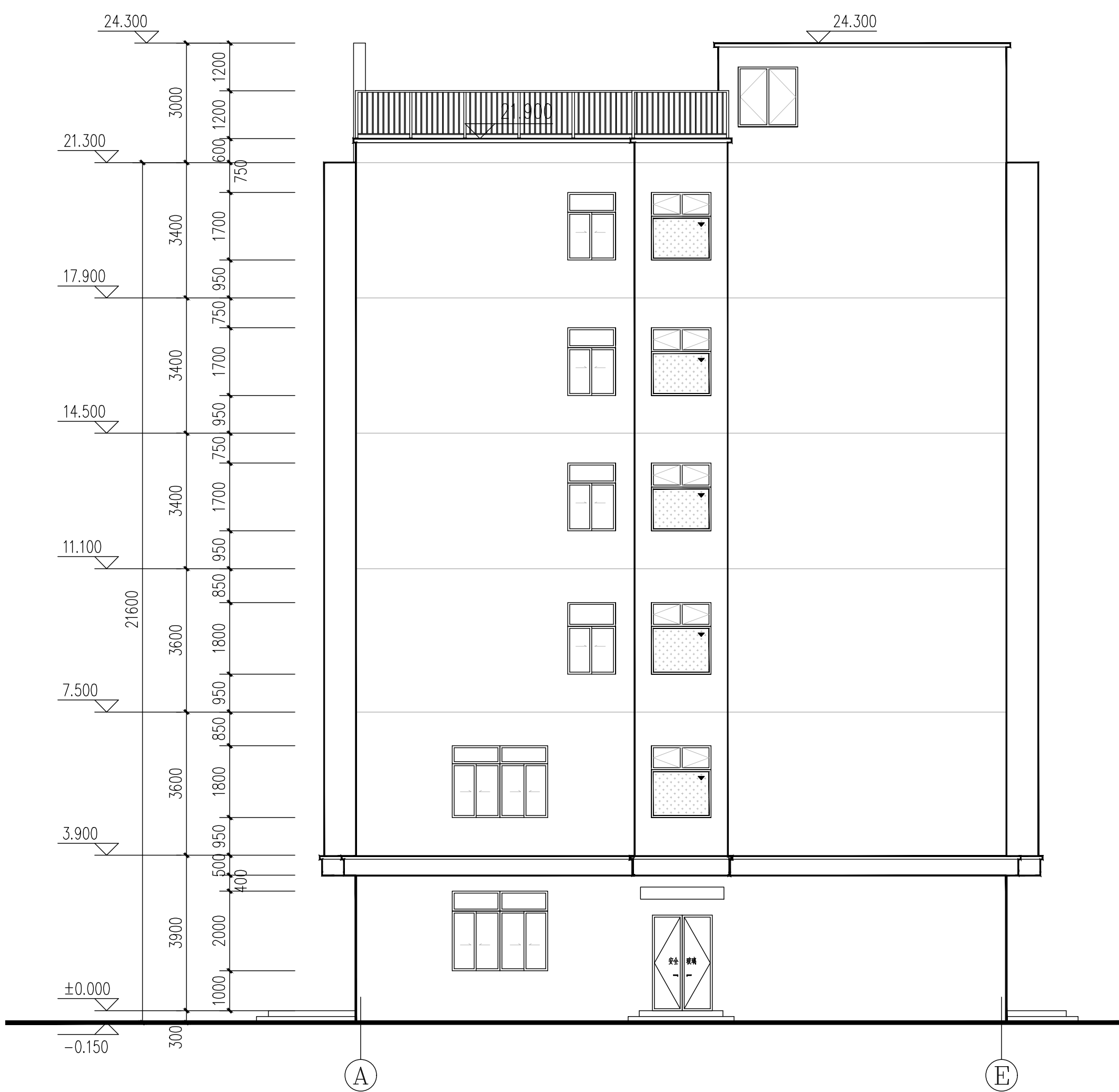
①~⑤立面图 1:100
