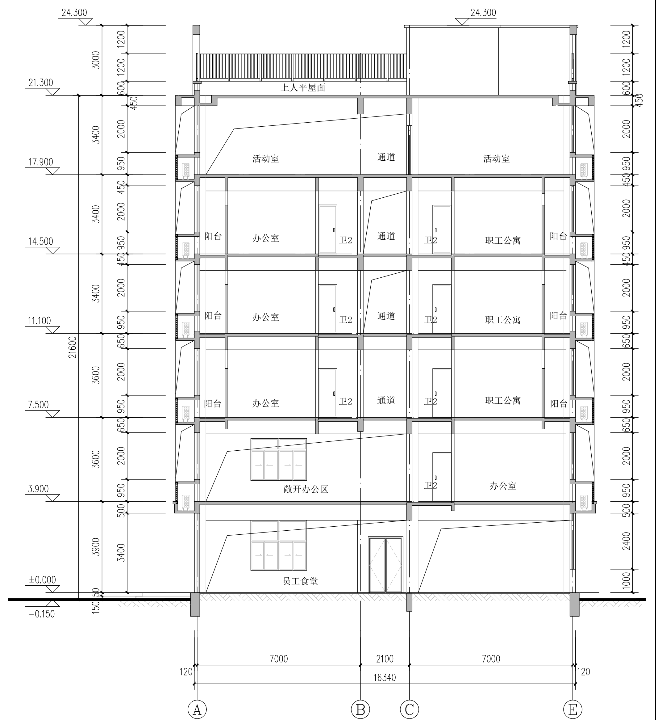
1-1剖面图 1:100
