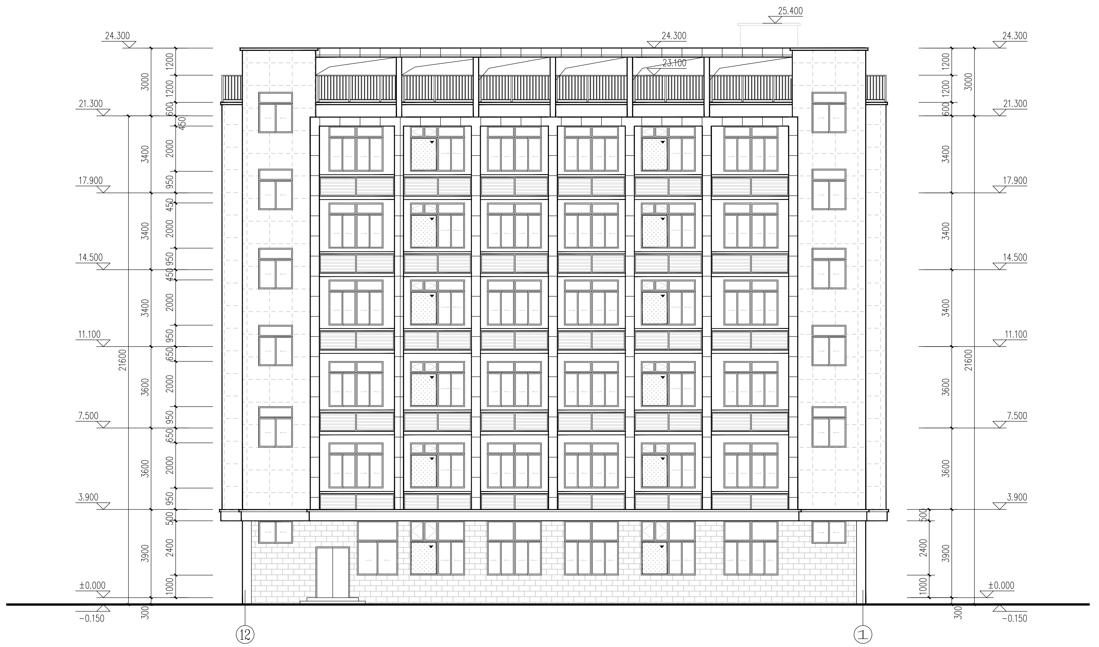
⑫~①立面图 1:100
