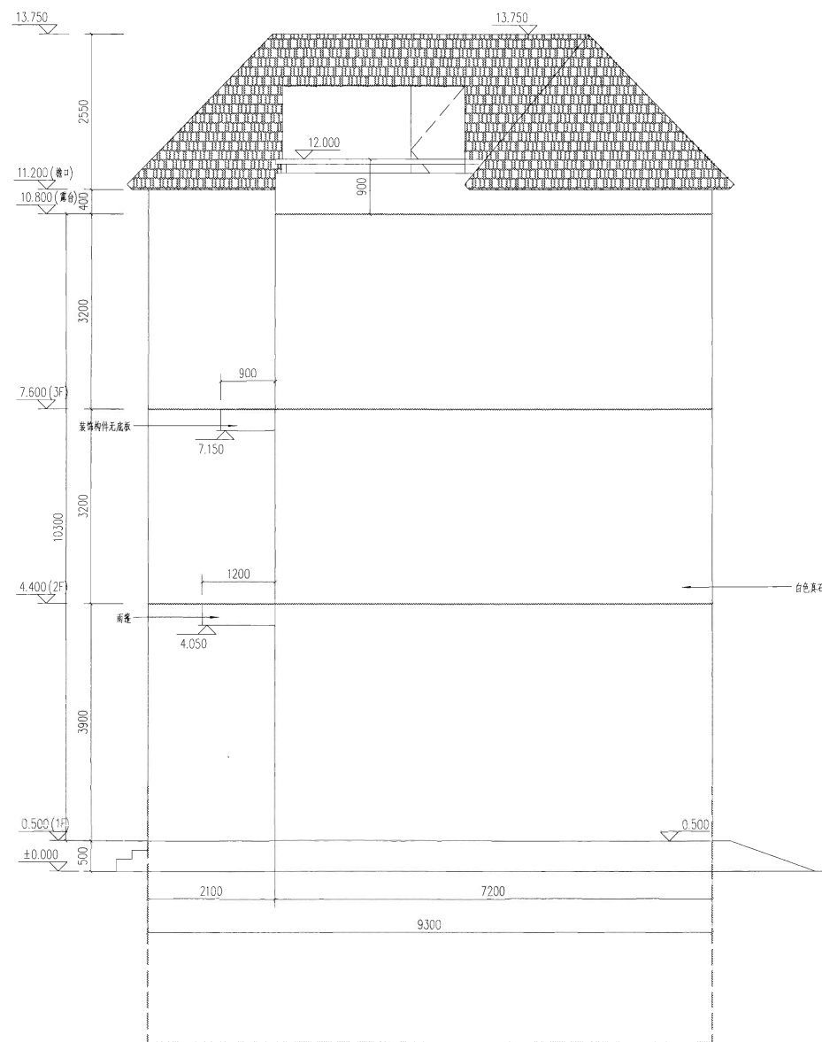
东立面 1:100
