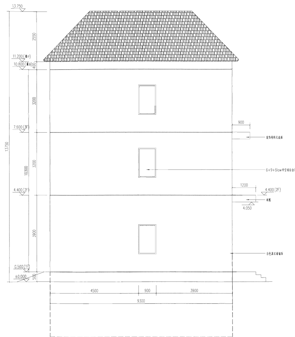
西立面 1:100
