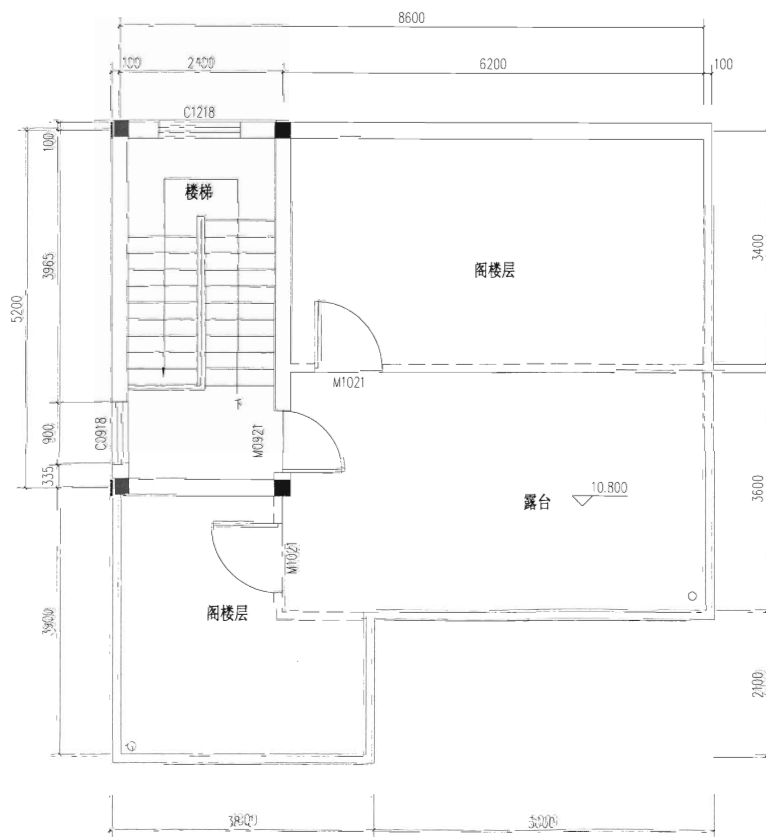
屋顶层
