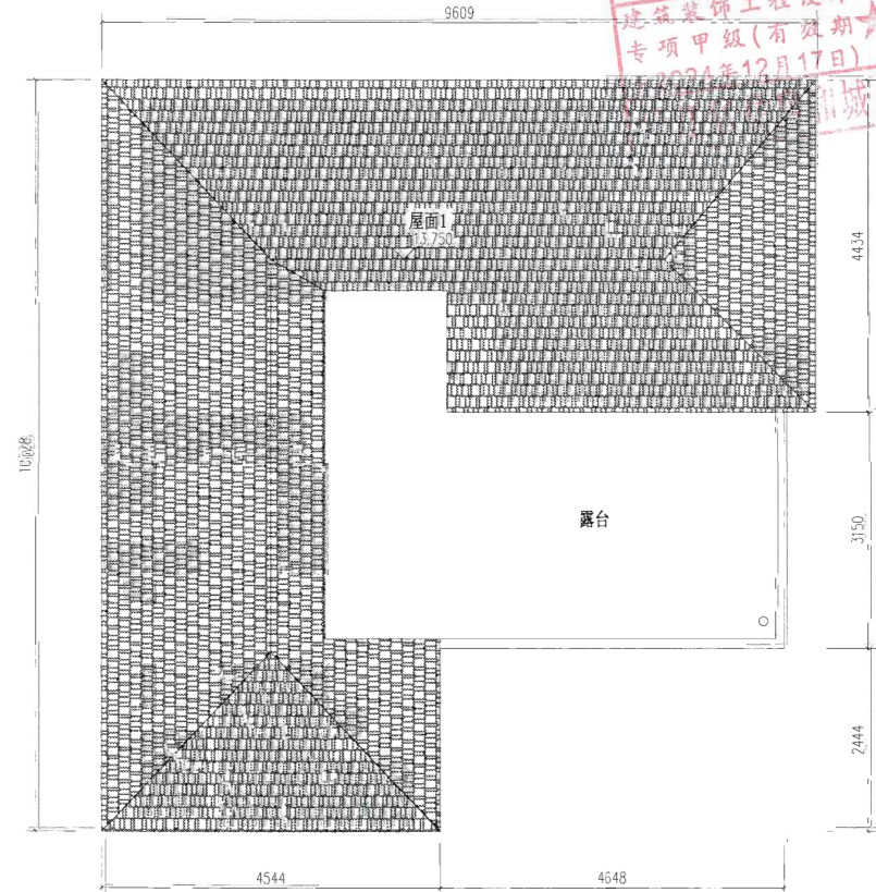
屋顶层
