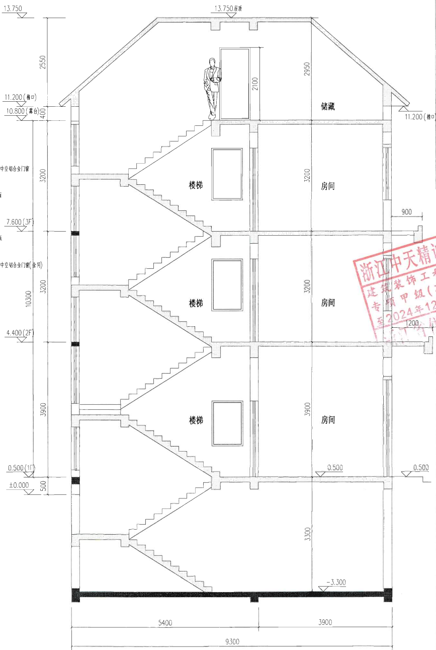
1-1剖面图100
