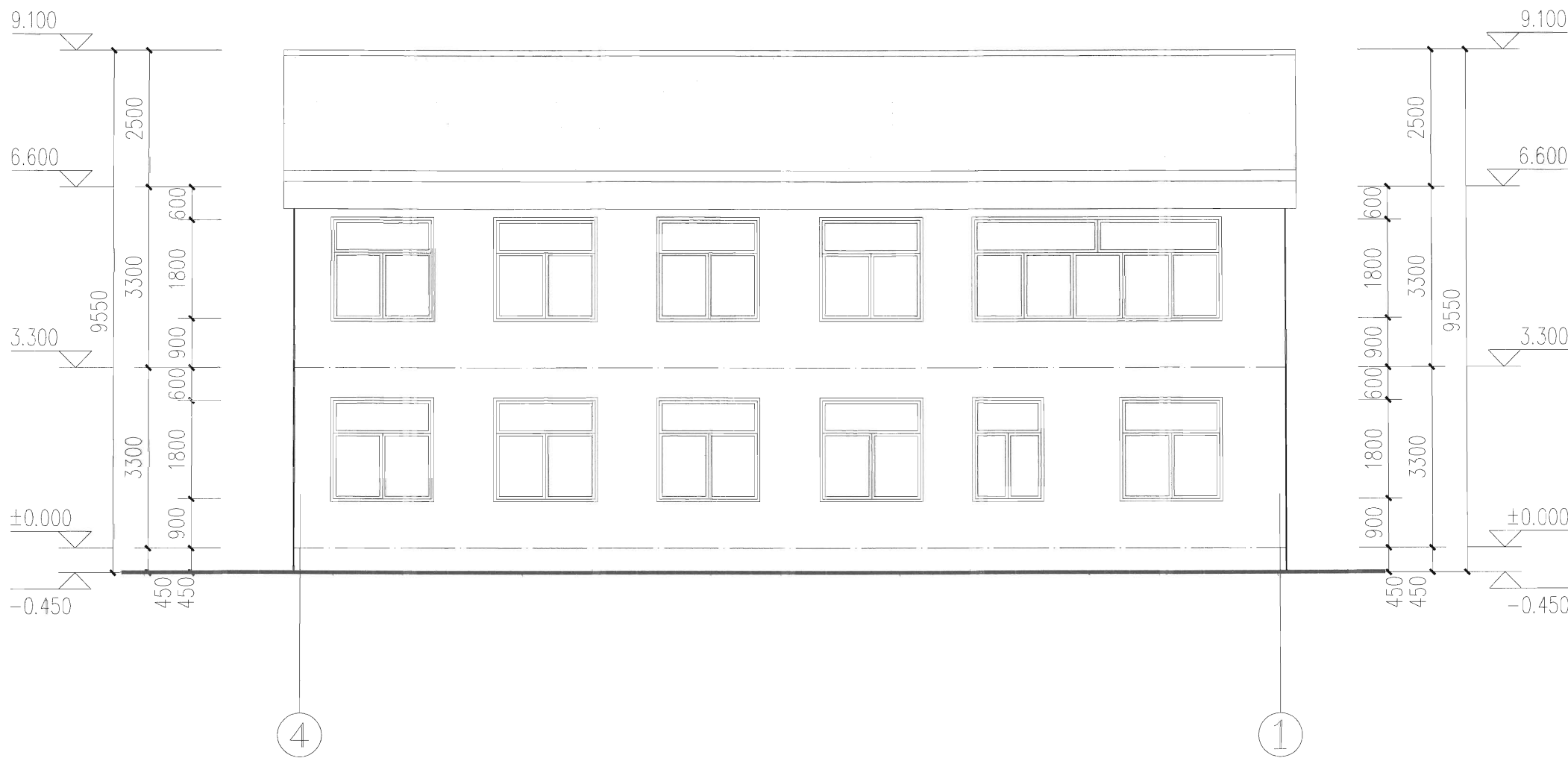
4-1轴立面图 1:100
