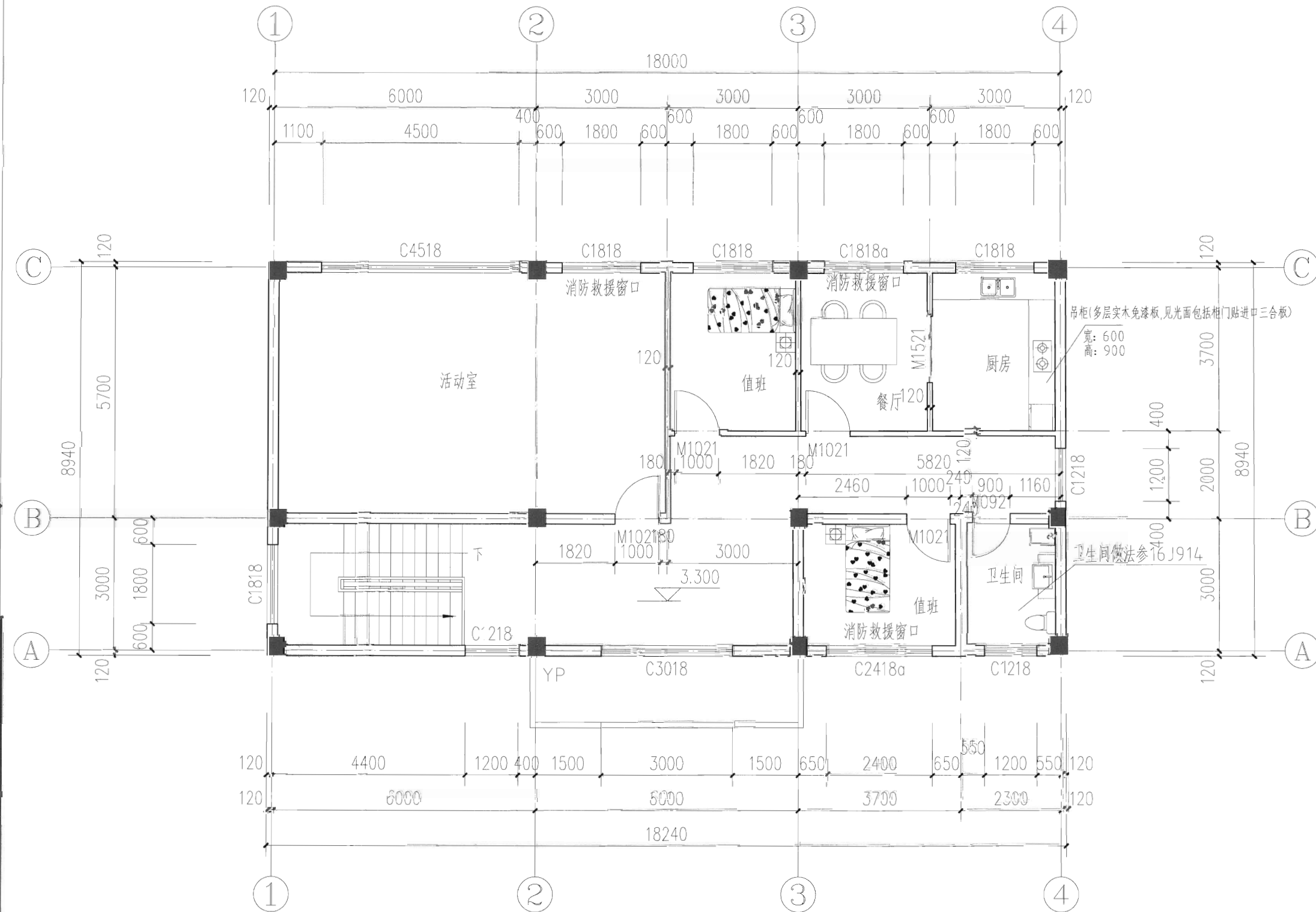
二层平面图 1:100
