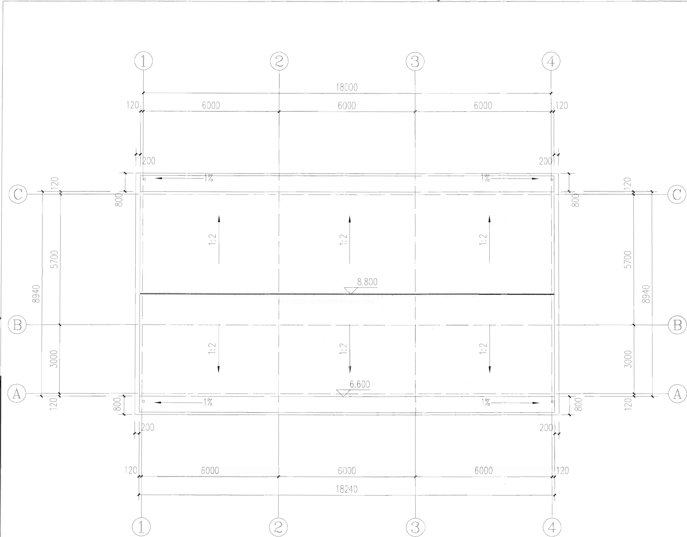
屋面层平面图 1:100
