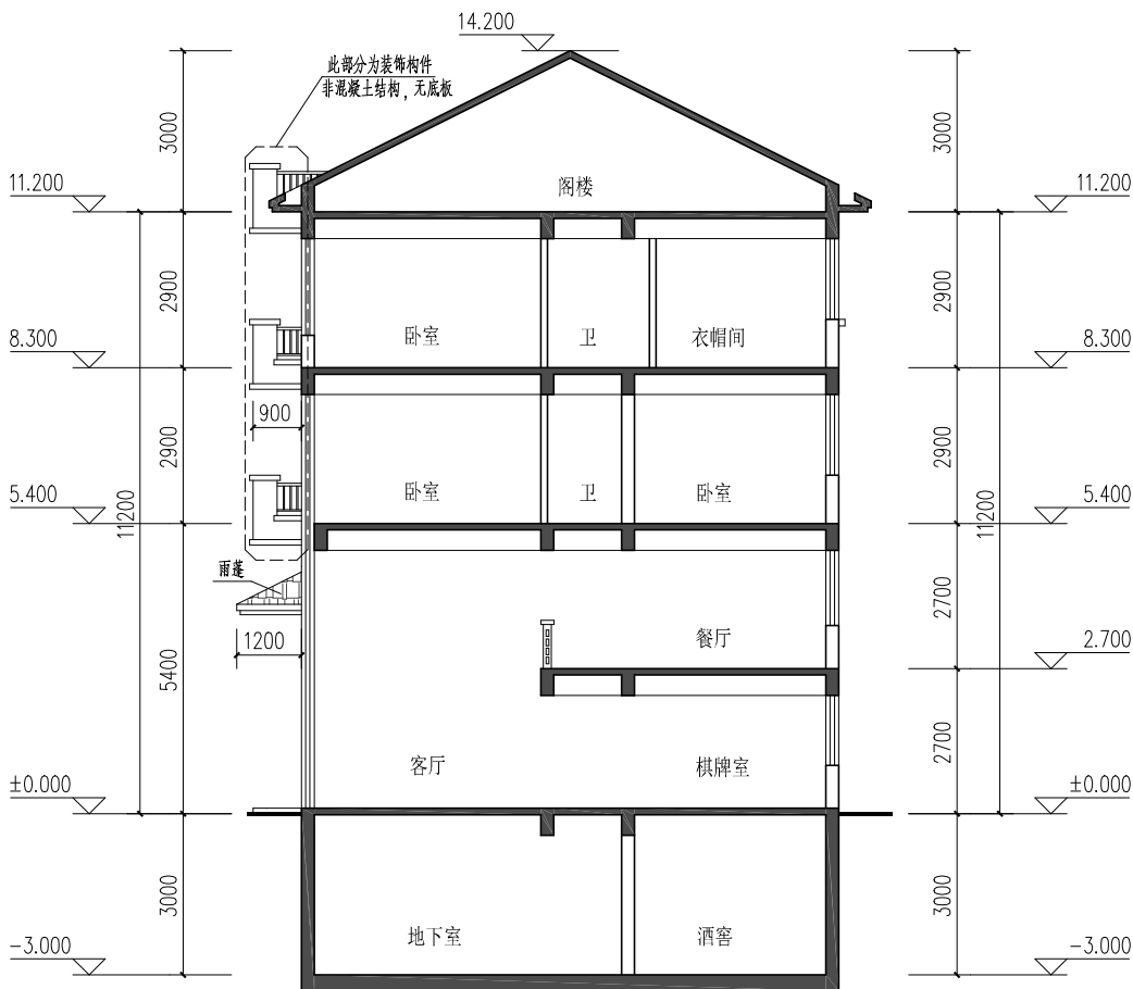
1-1剖面图
