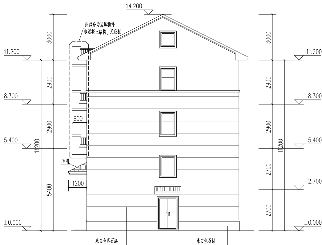
右立面图
