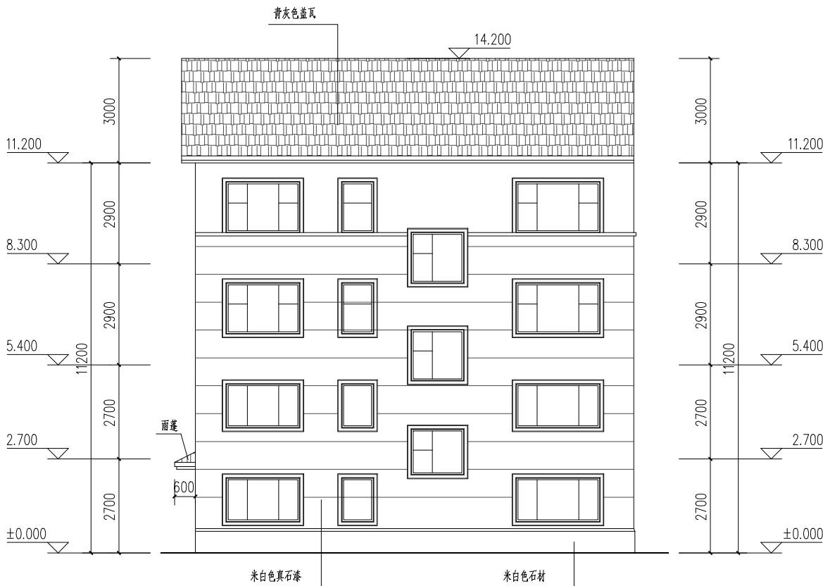
背立面图
