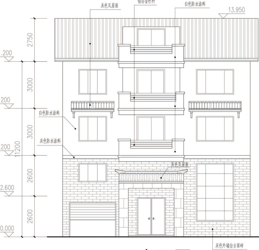
正立面图
