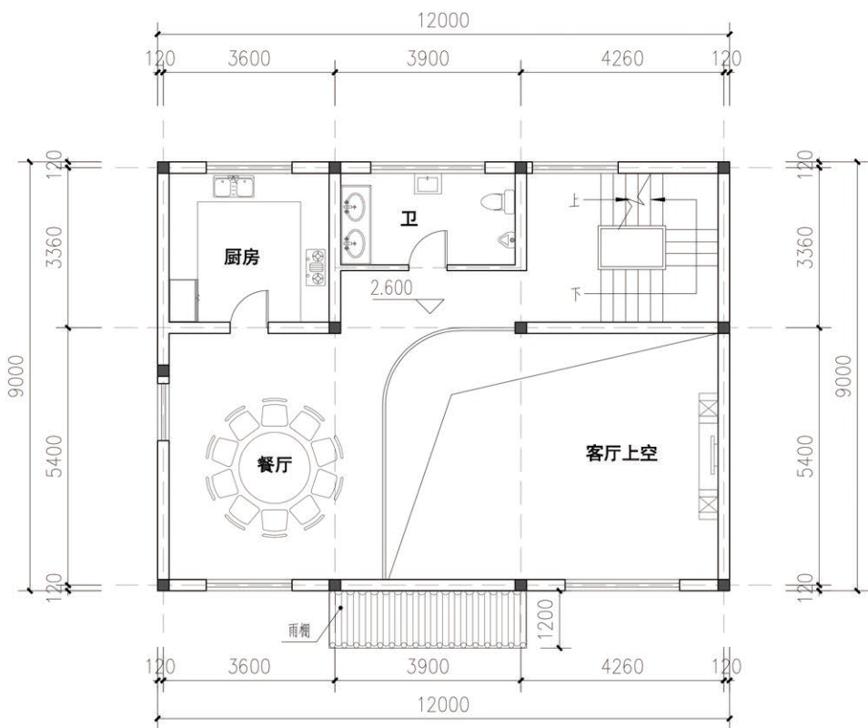
夹层平面图
