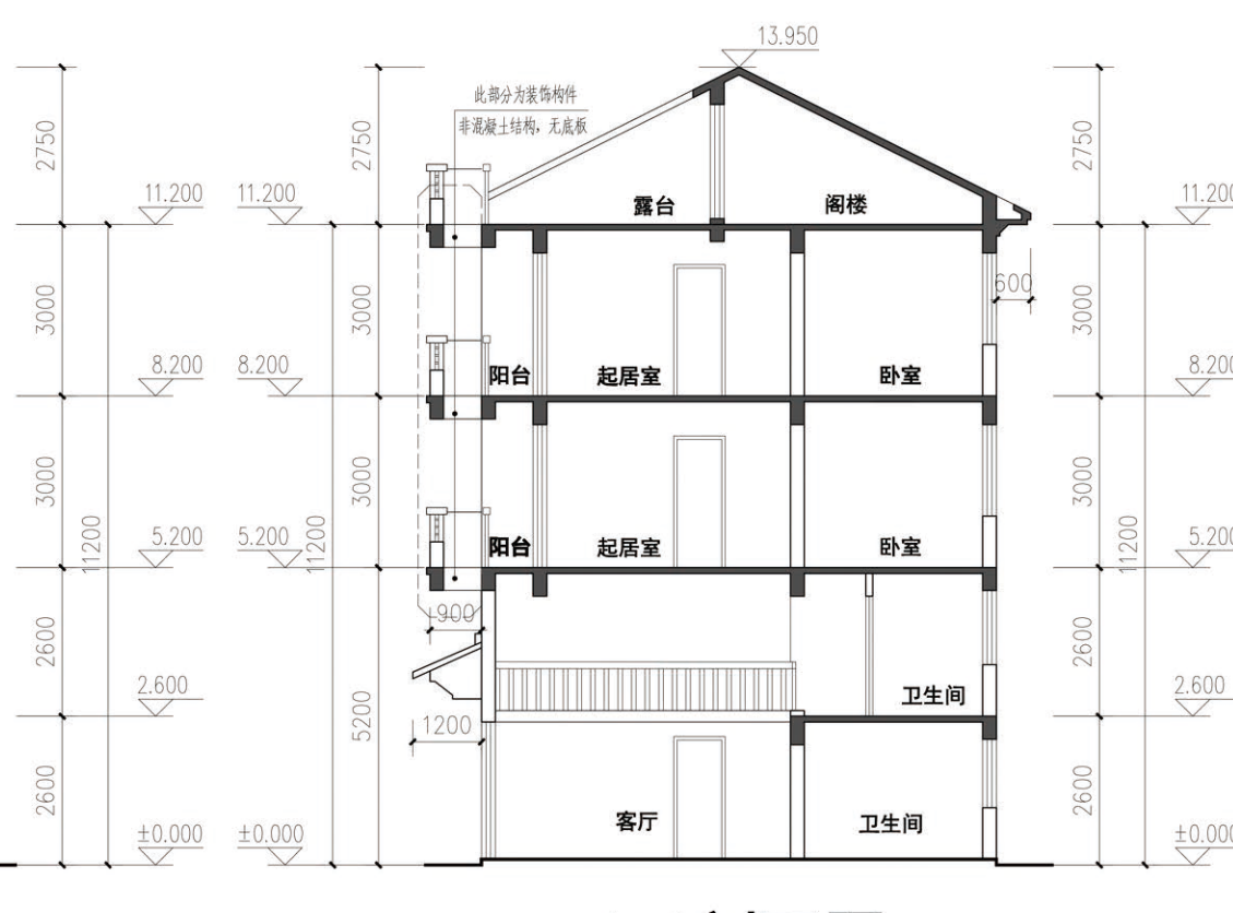
1-1剖面图
