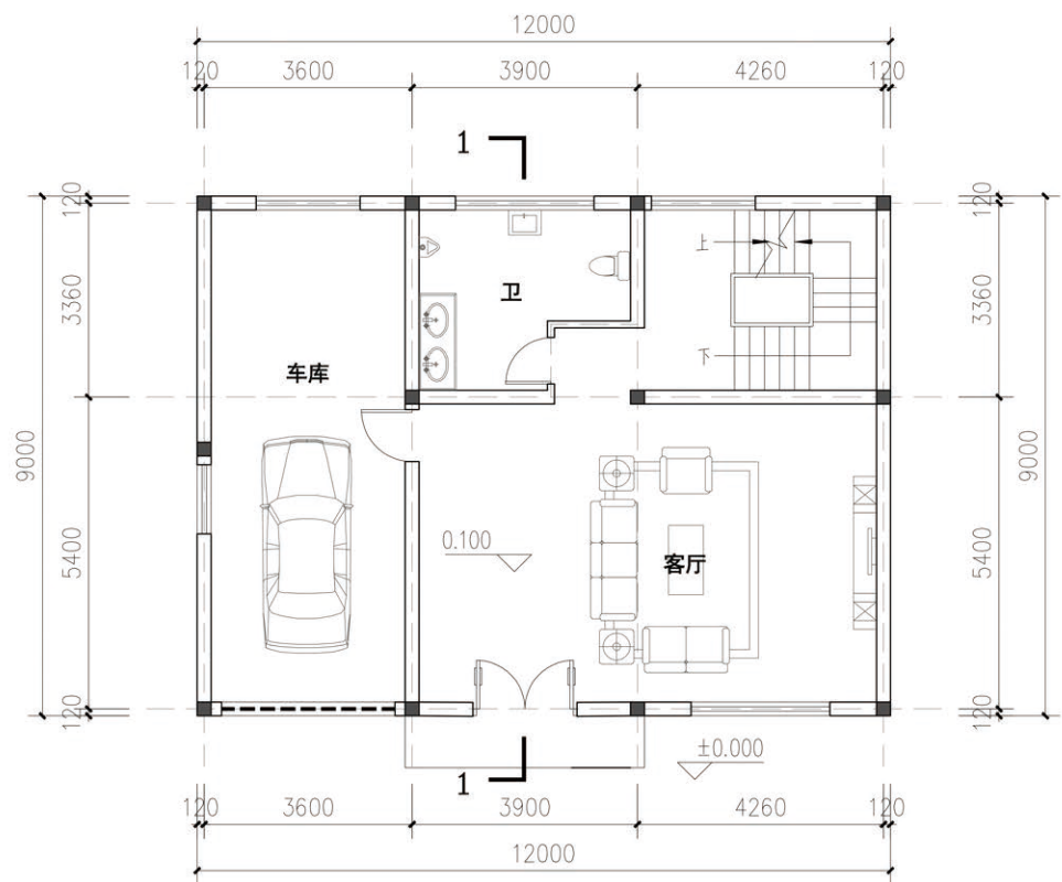
一层平面图
