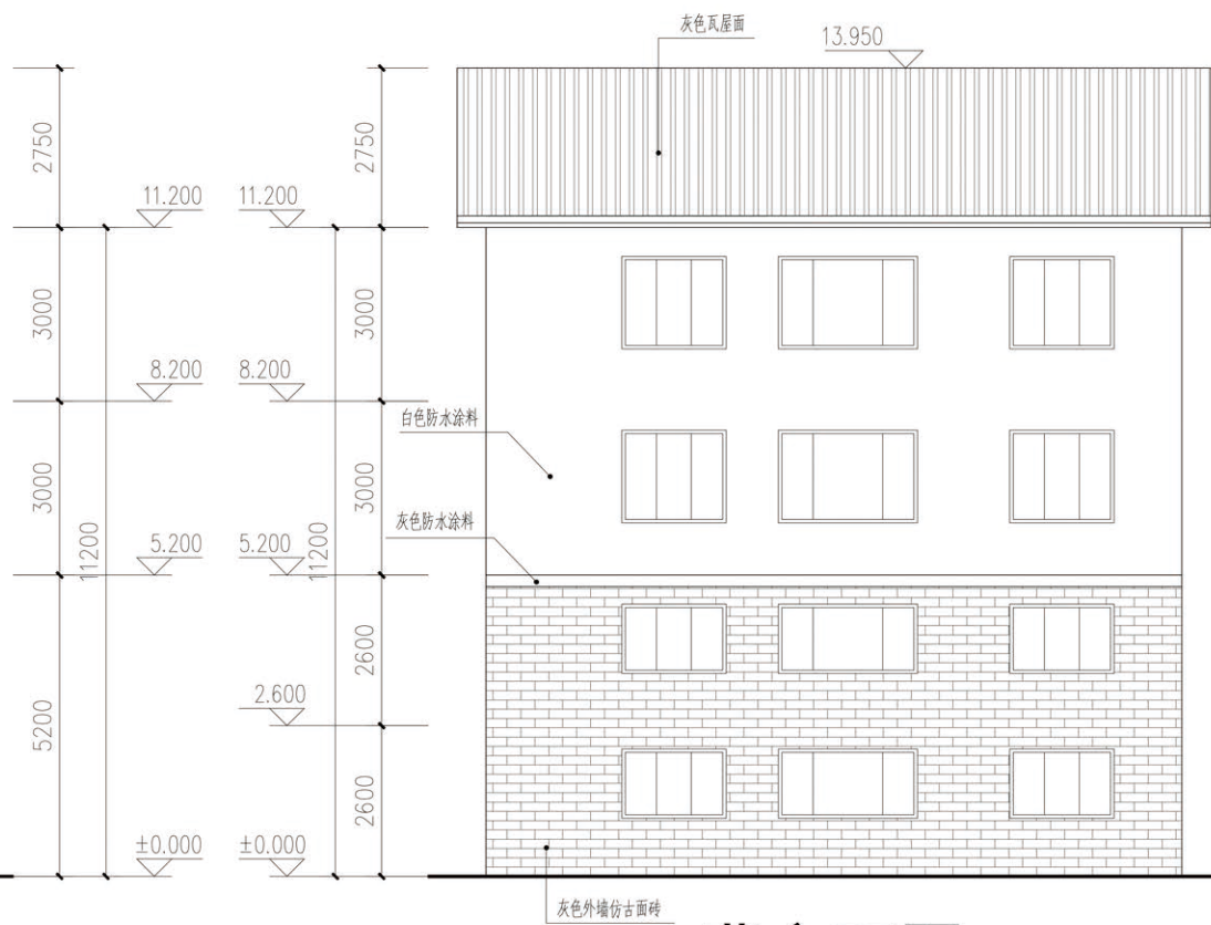
背立面图
