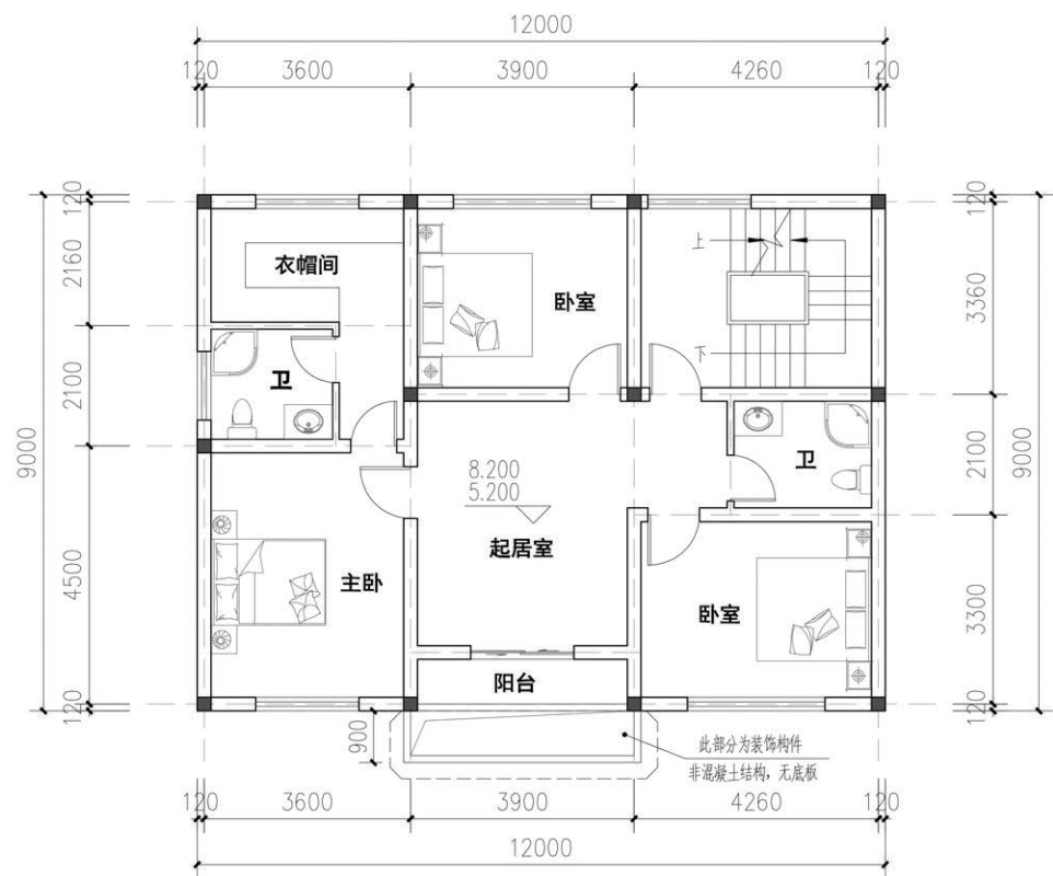
二、三层平面图
