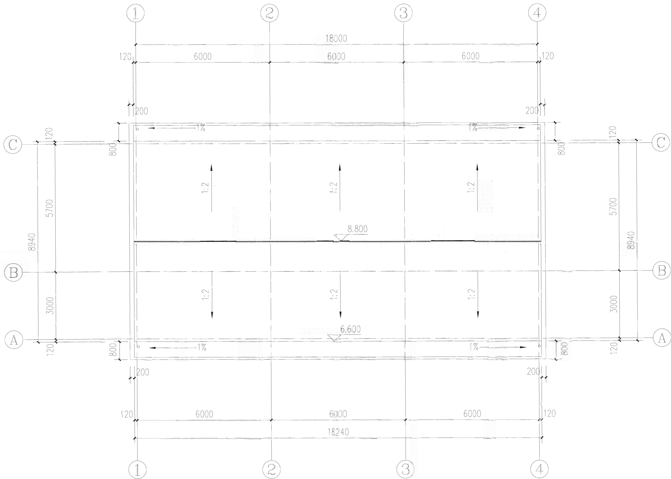
屋面层平面图 1:100
