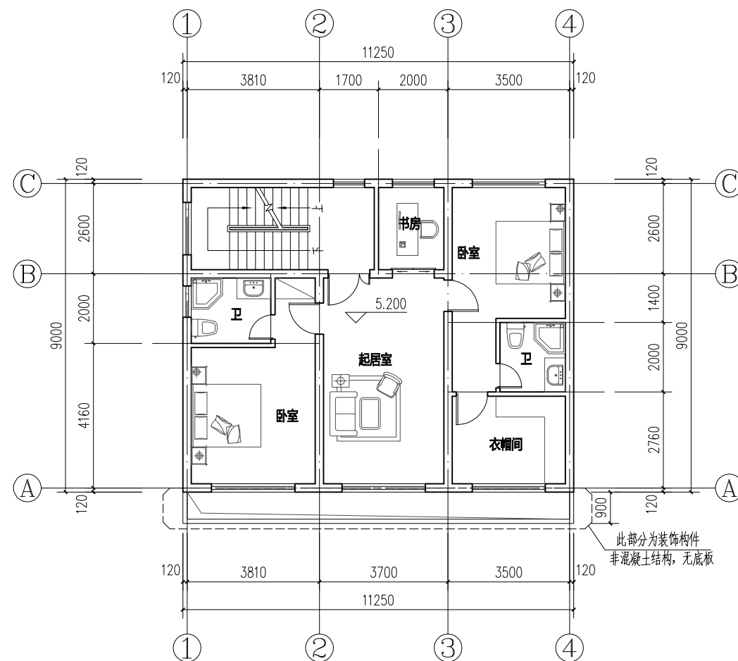
二层平面图
