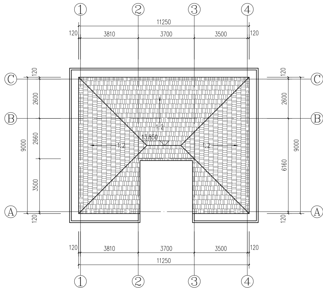
屋顶平面图
