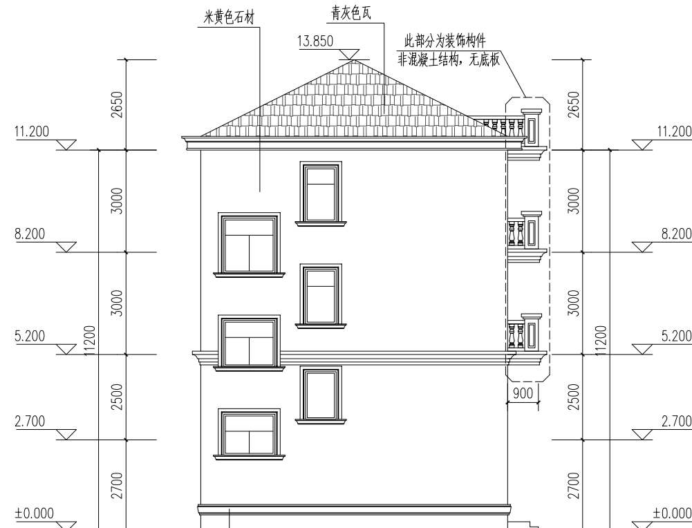
左立面图
