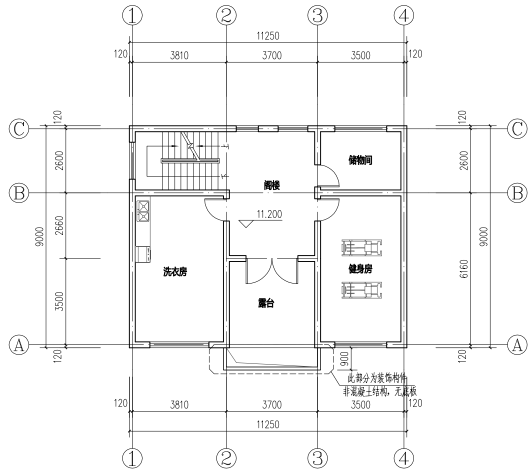
阁楼层平面图
