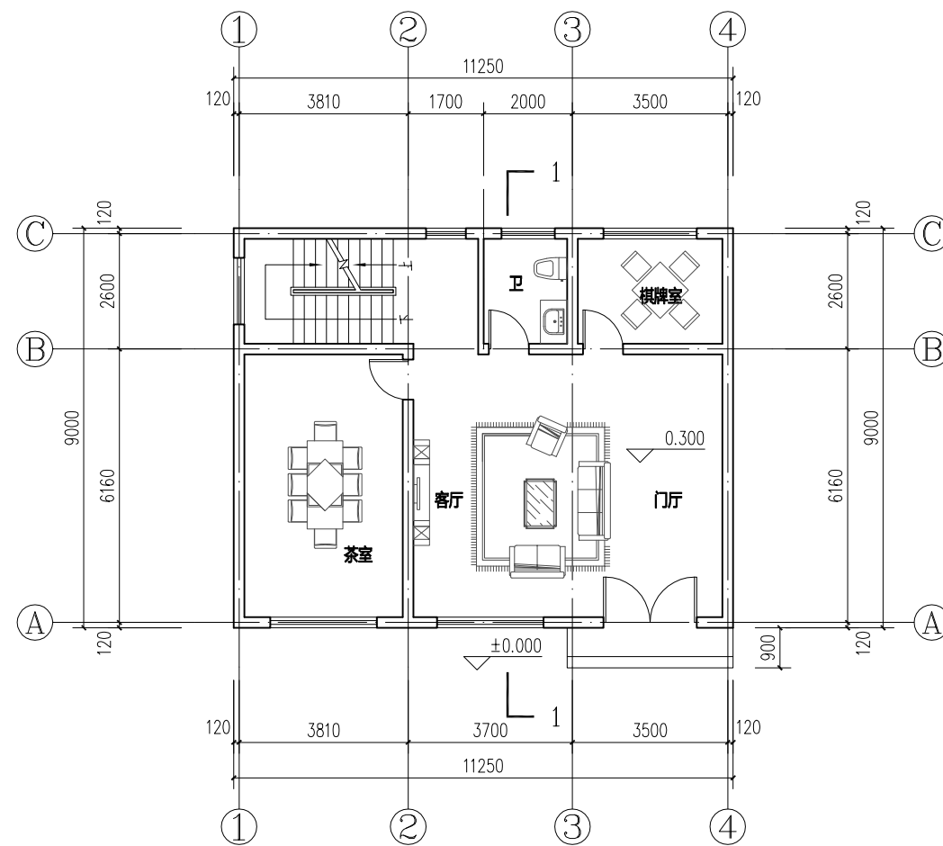
一层平面图
