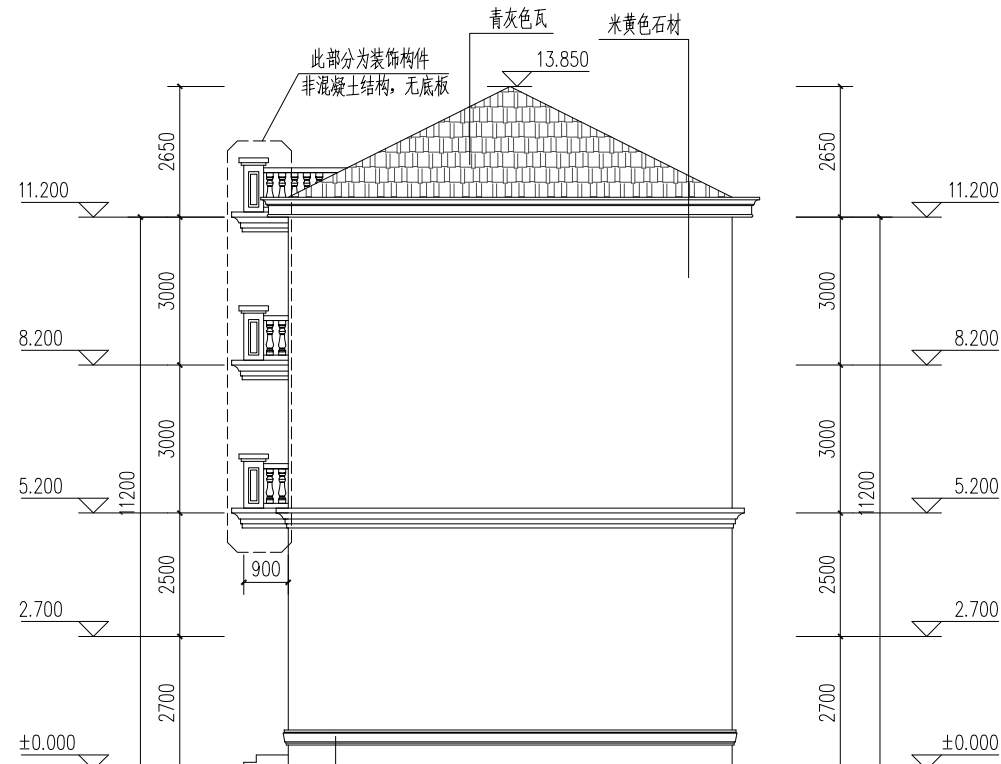
右立面图
