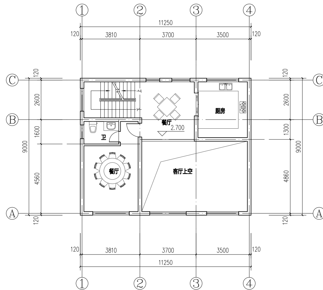
夹层平面图
