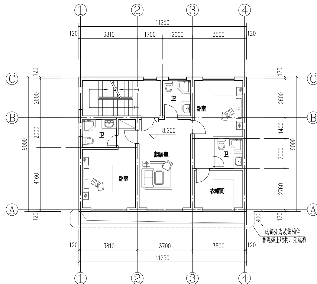
三层平面图
