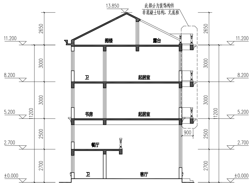
1-1剖面图
