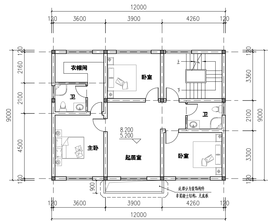
二、三层平面图
