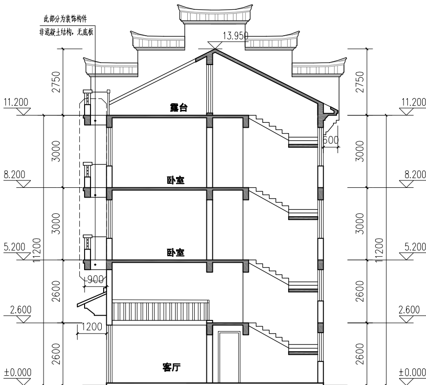
1-1剖面图
