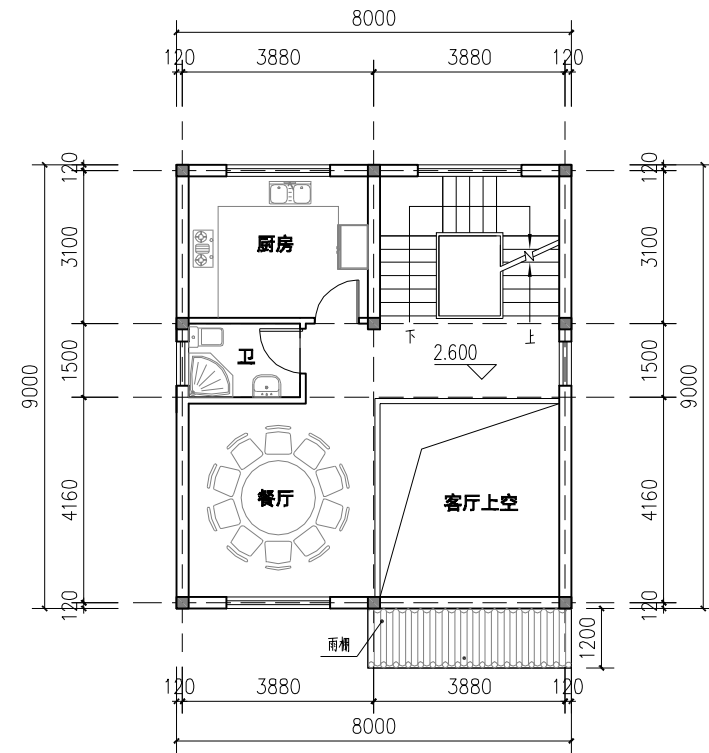
夹层平面图
