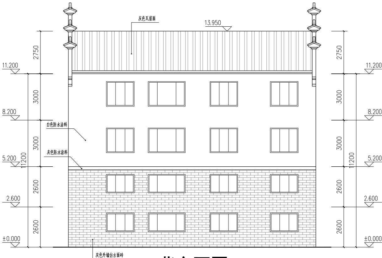
背立面图
