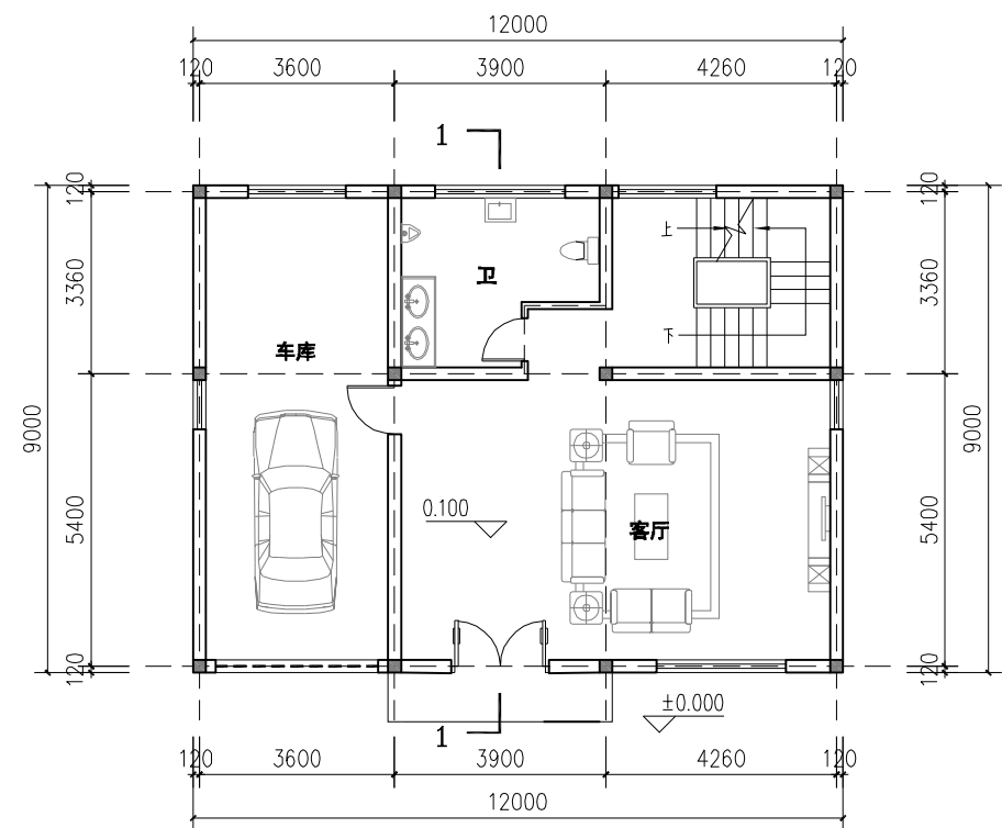
一层平面图
