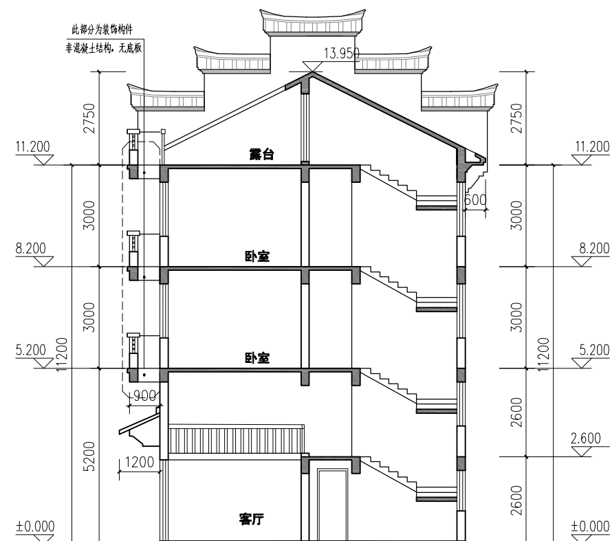
1-1剖面图
