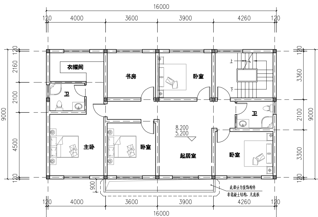
二、三层平面图
