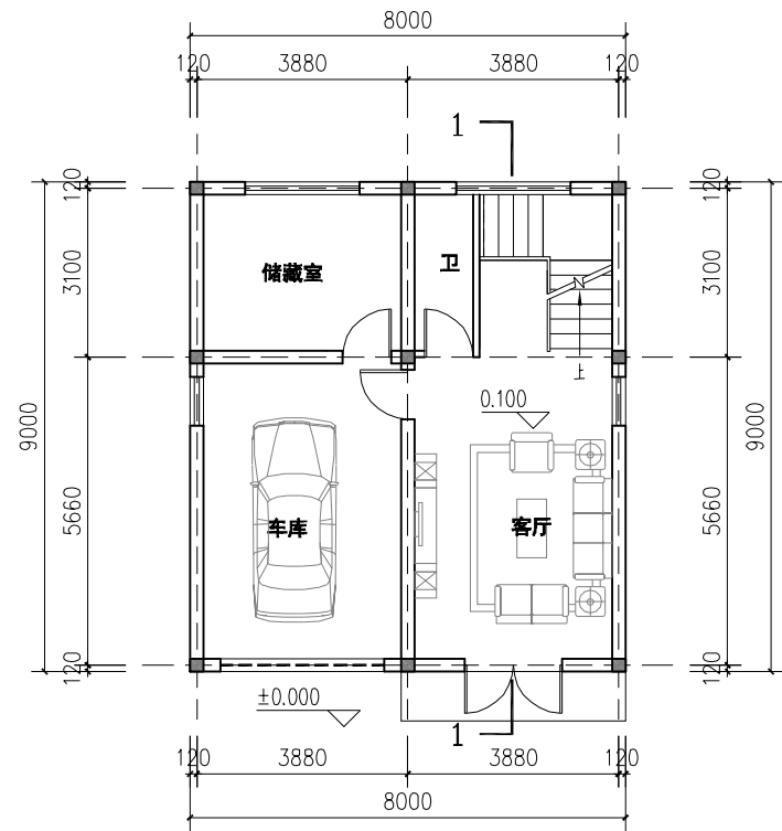
一层平面图
