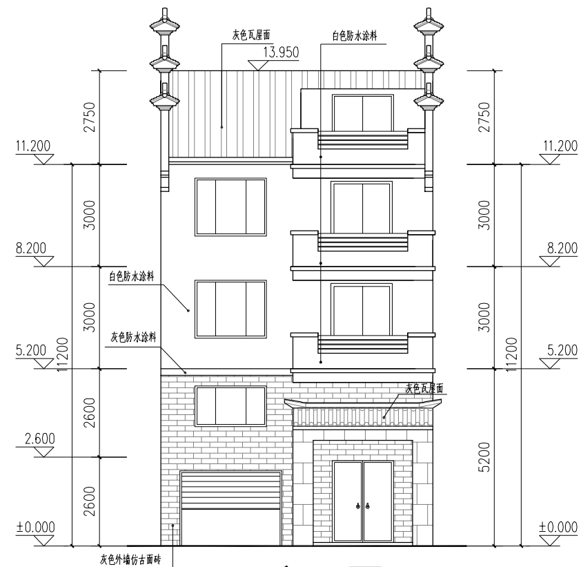
正立面图
