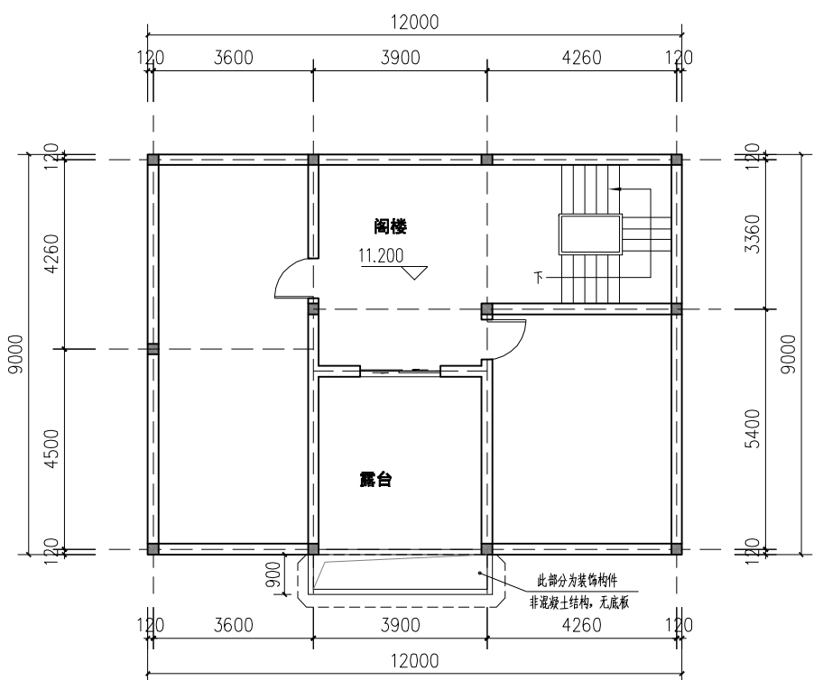
阁楼层平面图
