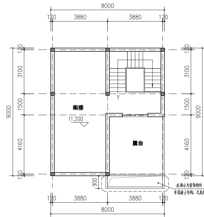
阁楼层平面图
