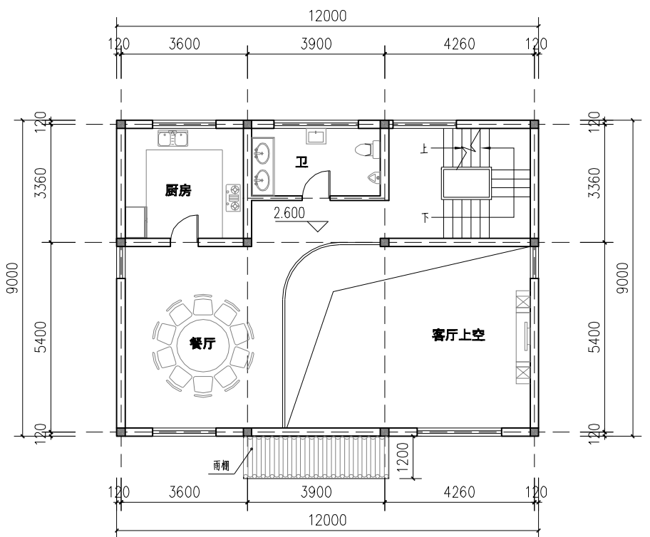
夹层平面图
