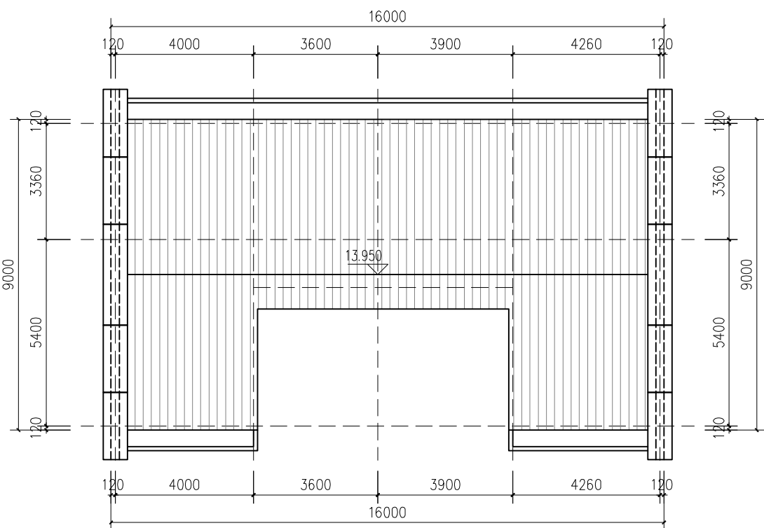
屋顶层平面图
