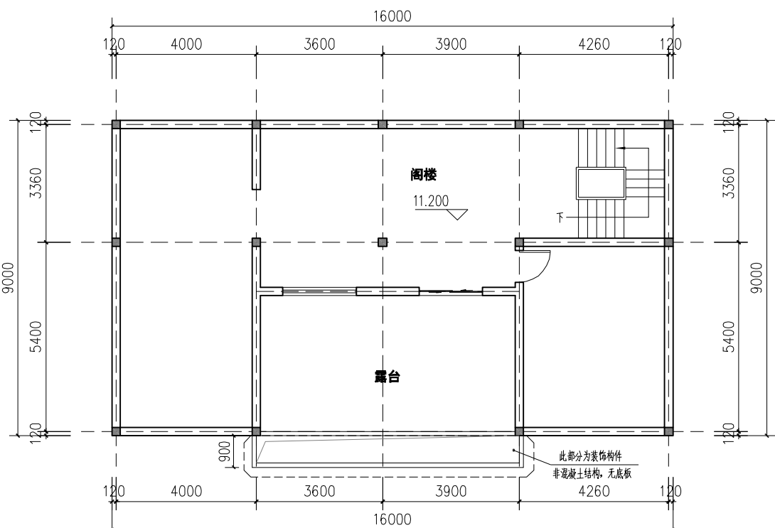
阁楼层平面图
