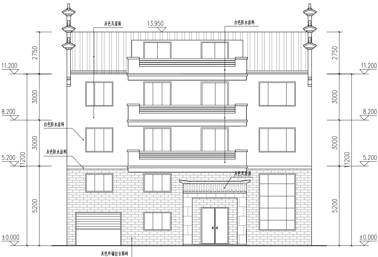
正立面图
