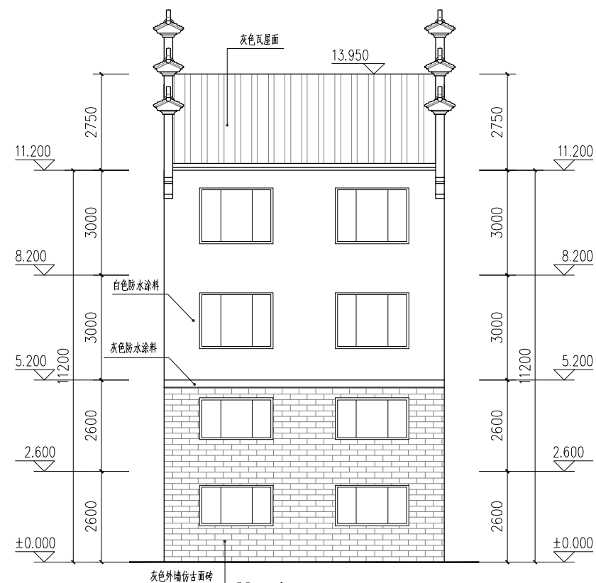
背立面图
