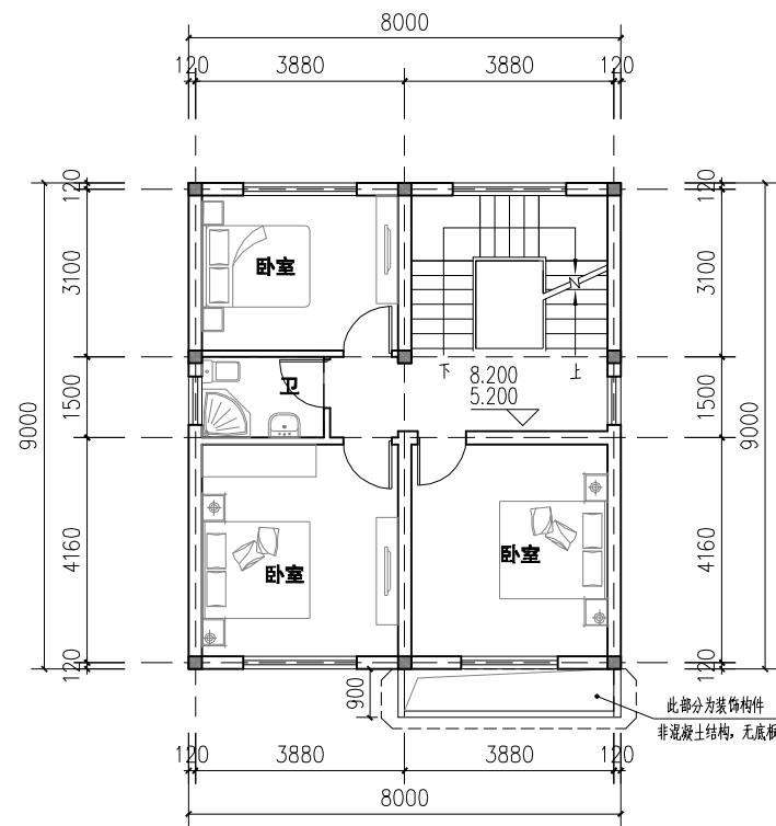
二、三层平面图
