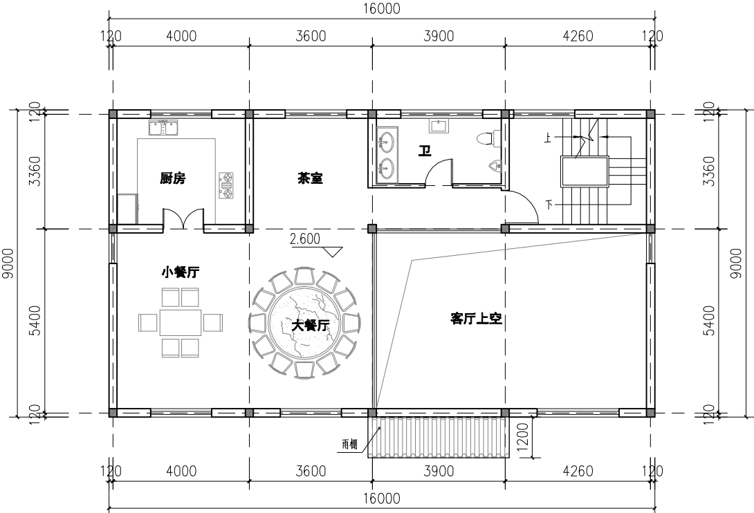
夹层平面图
