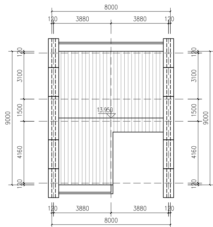
屋顶层平面图
