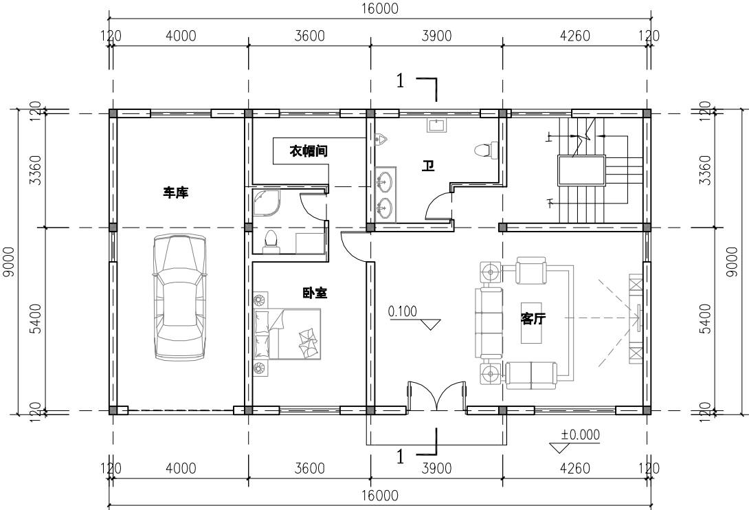
一层平面图
