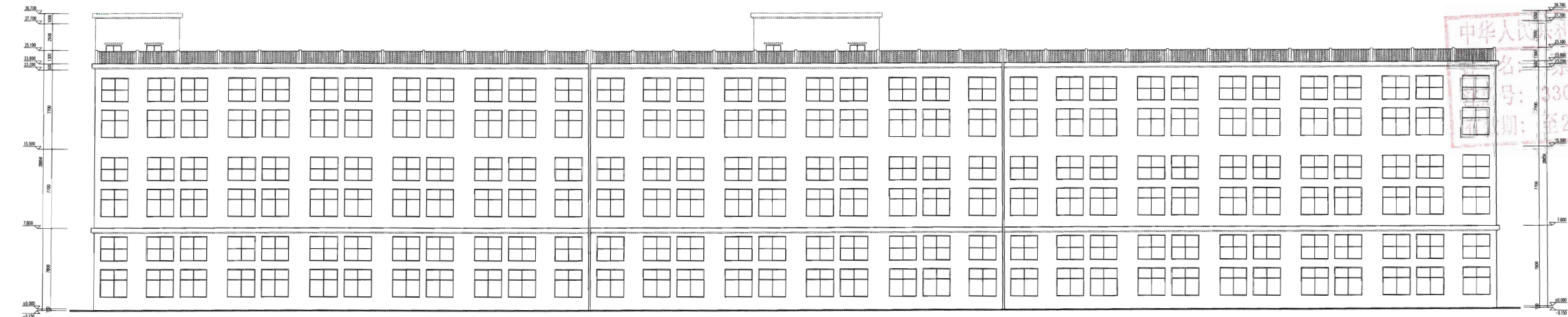
南立面图 1:100
