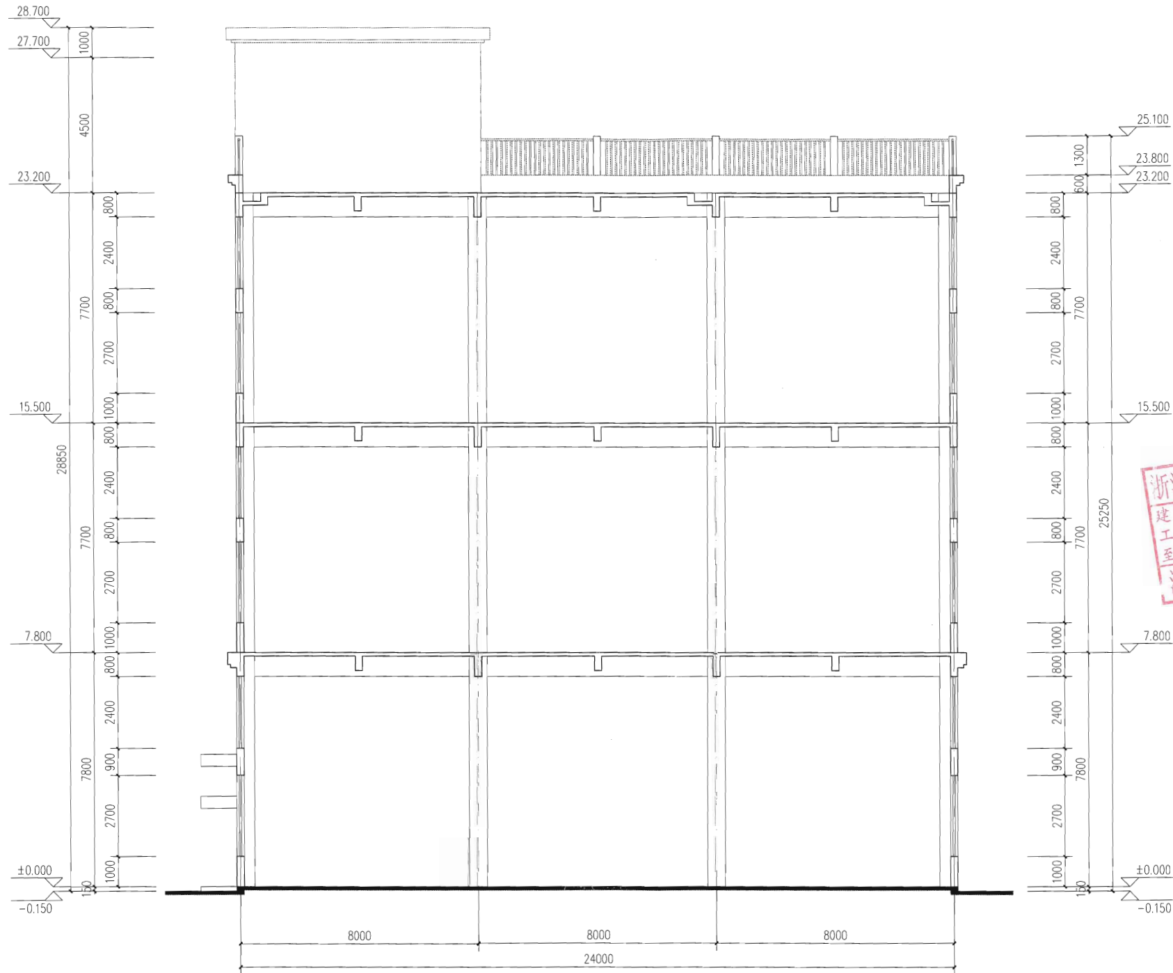
1-1剖面图 1:100
