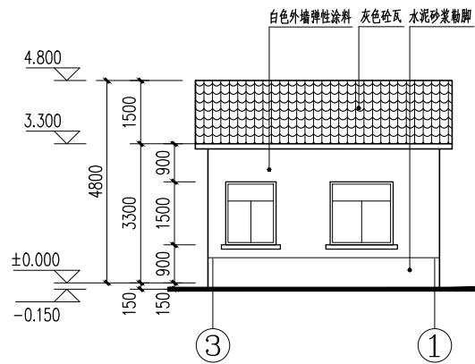
③—①立面图 1:100
