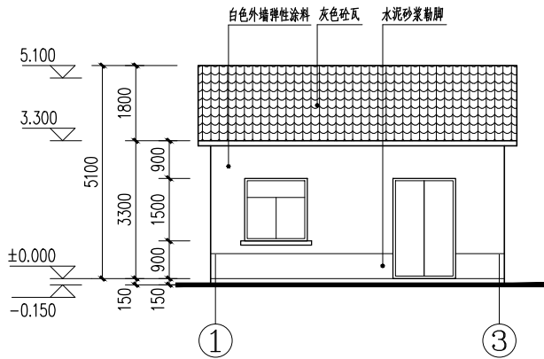
①—③立面图 1:100
