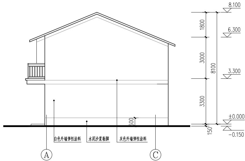
①—③立面图 1:100
