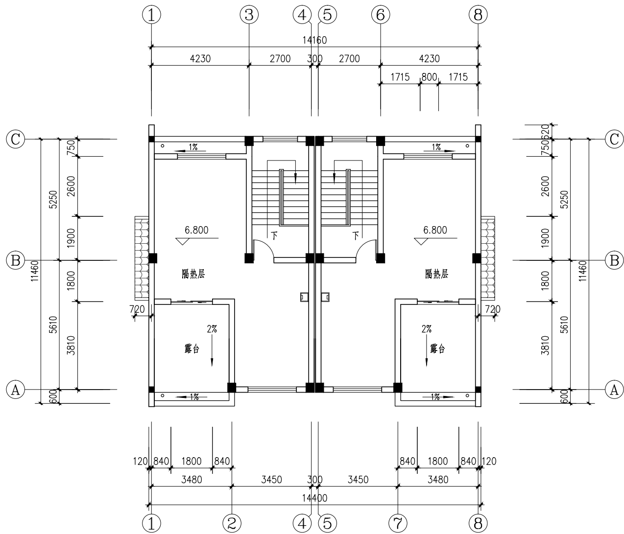
隔热层平面图 1:150
