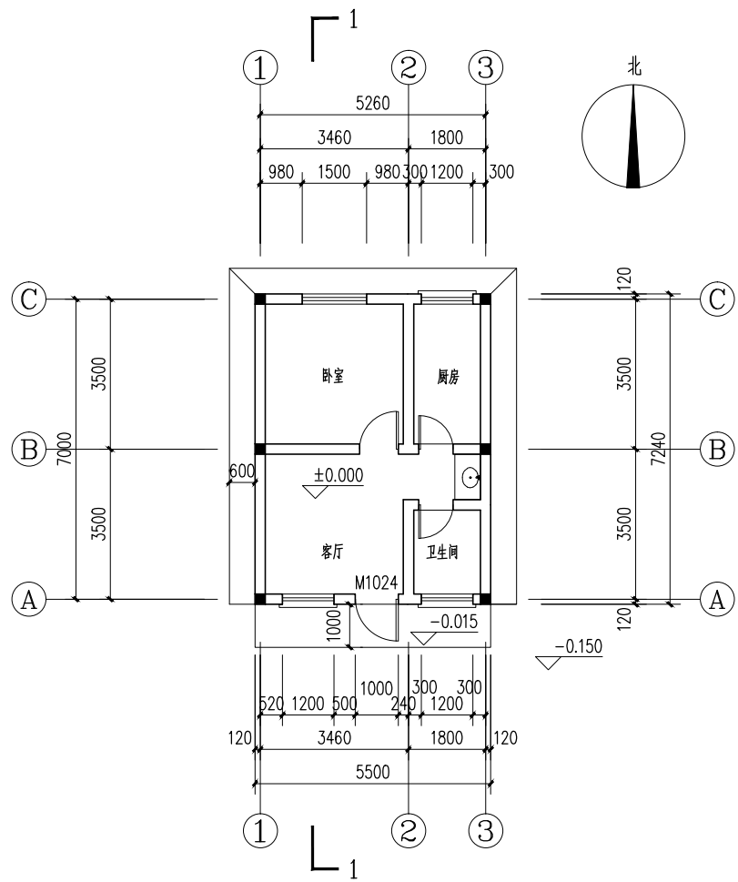
一层平面图 1:100
