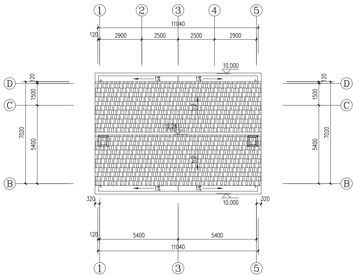
屋面层平面图 1:100
