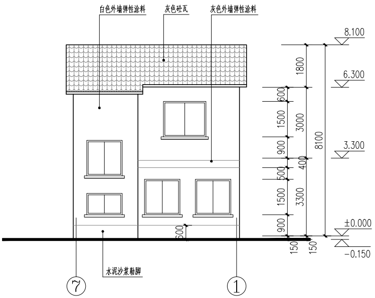
⑦—①立面图 1:100
