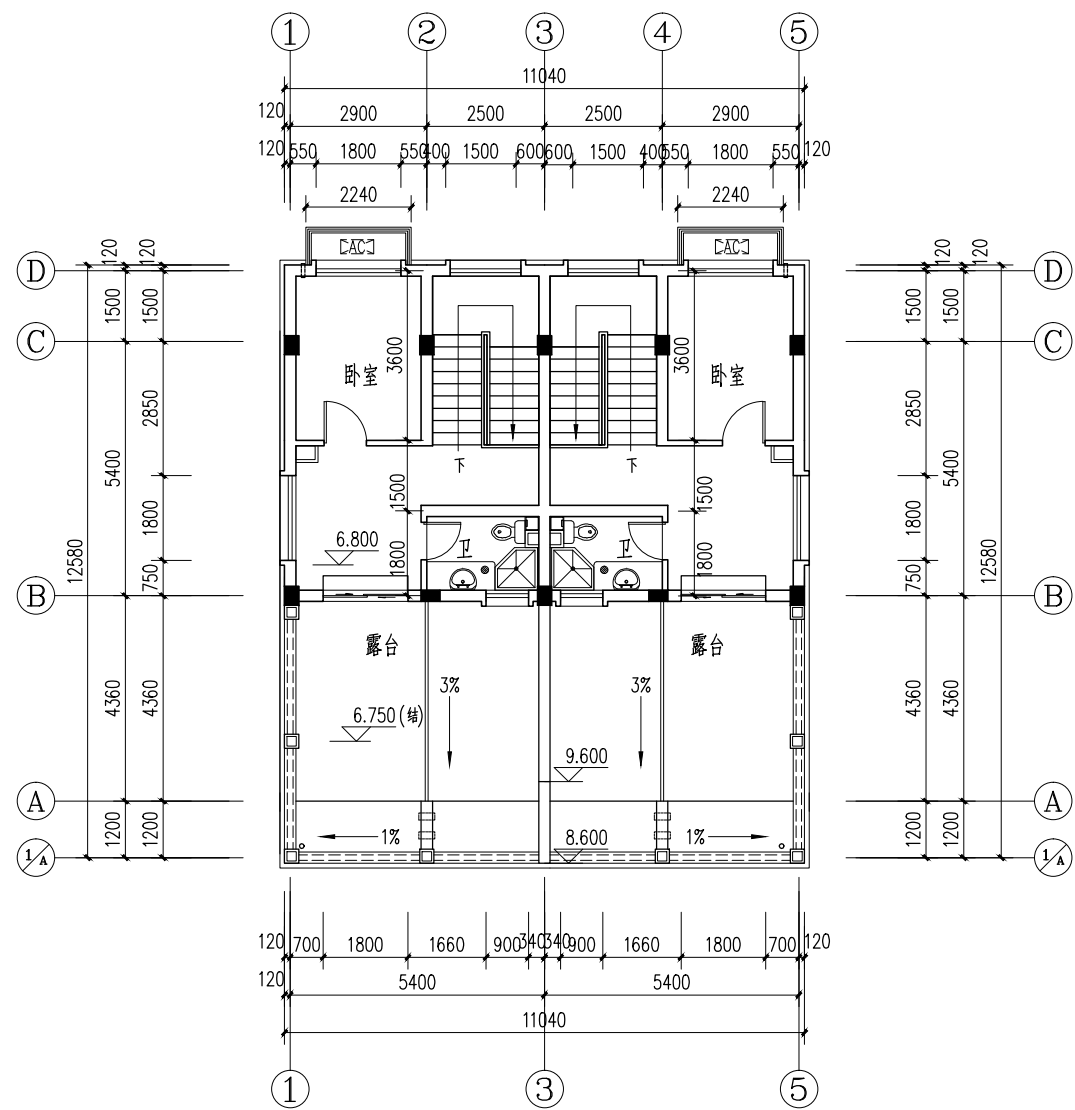
三层平面图 1:100
