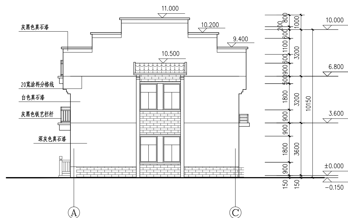
Ⓐ—Ⓒ 立面图 1:150
