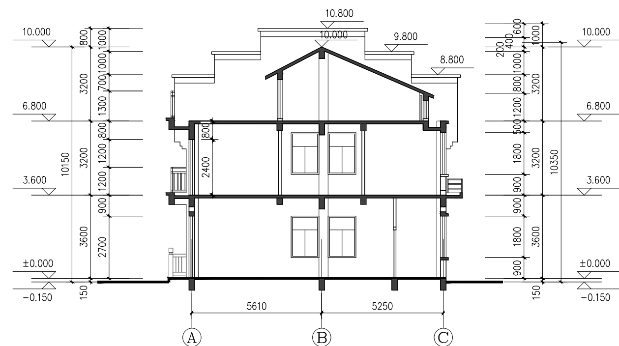
1-1 剖面图 1:150
