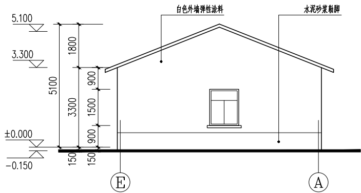
E—A立面图 1:100
