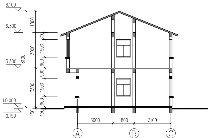
1—1剖面图 1:100
