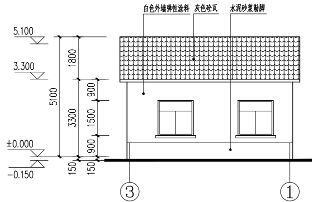
③—①立面图 1:100
