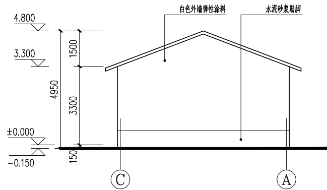
③—A立面图 1:100
