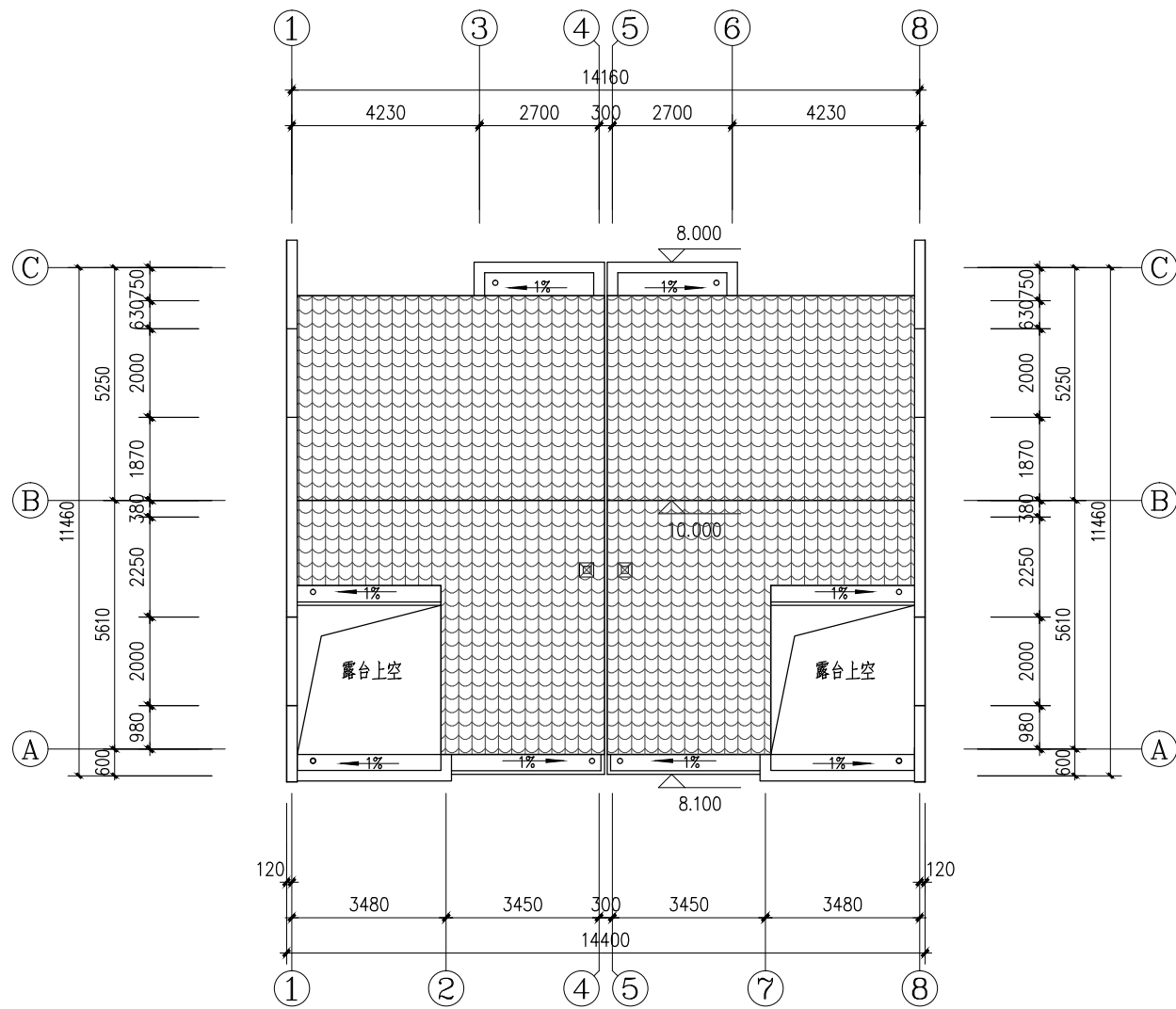
屋顶平面图 1:150
