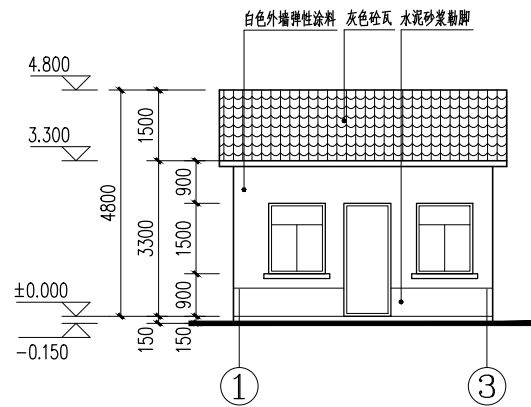
①—③立面图 1:100
