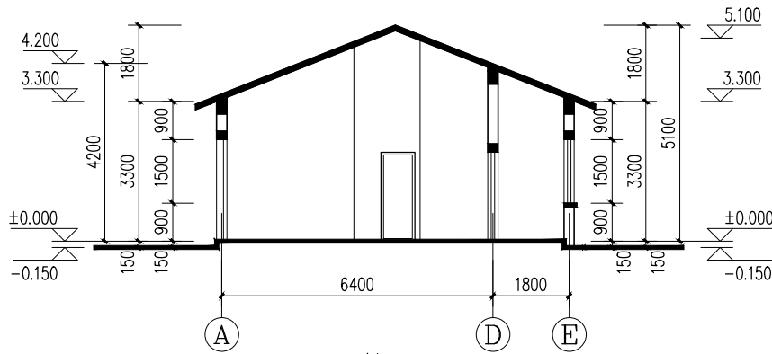
1—1剖面图 1:100
