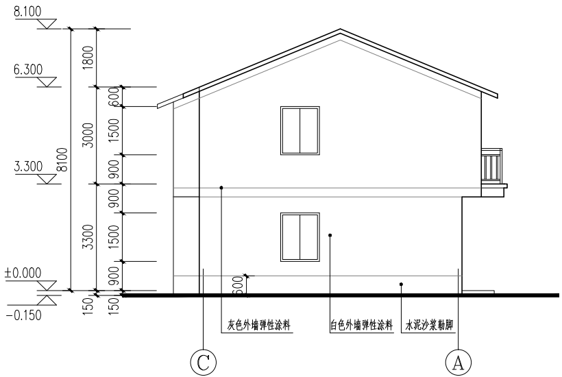
③—①立面图 1:100
