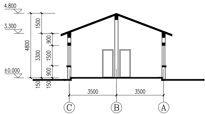
1—1剖面图 1:100
