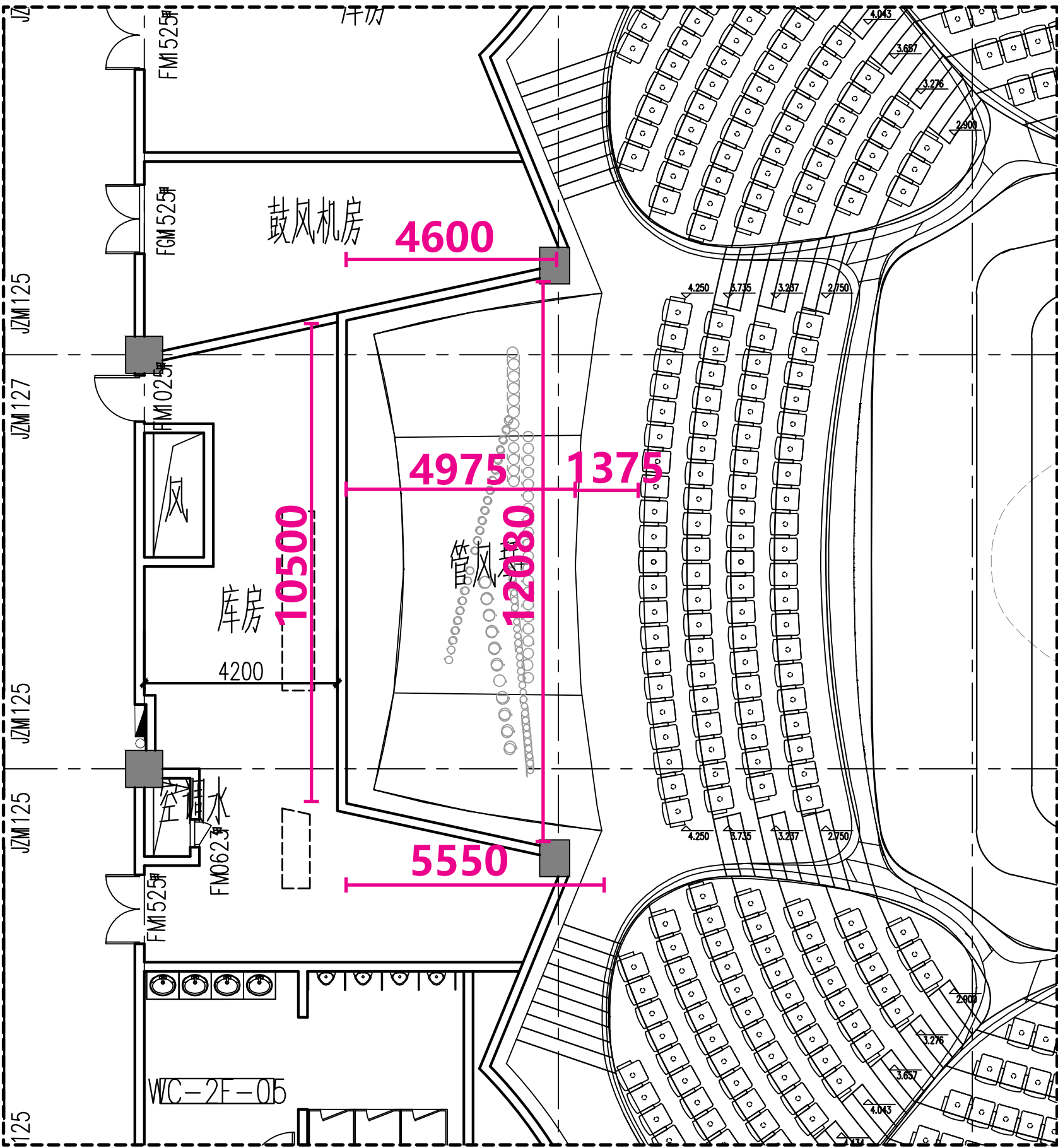
F2平面图
