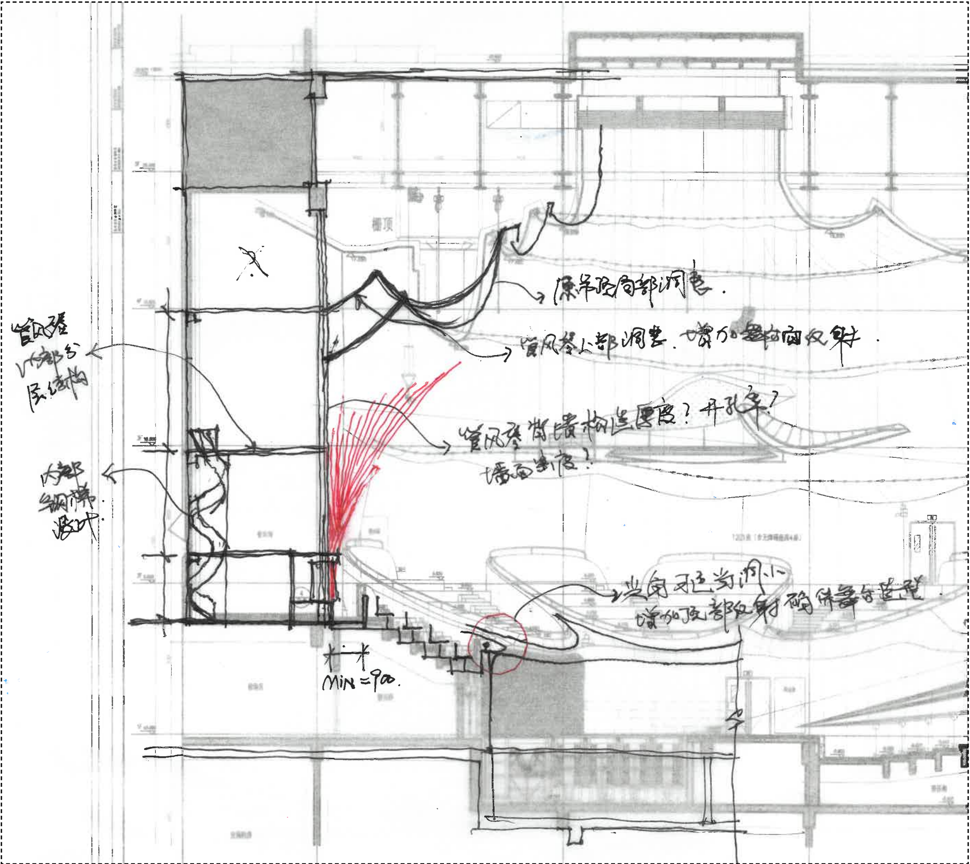
A-A剖立面图
