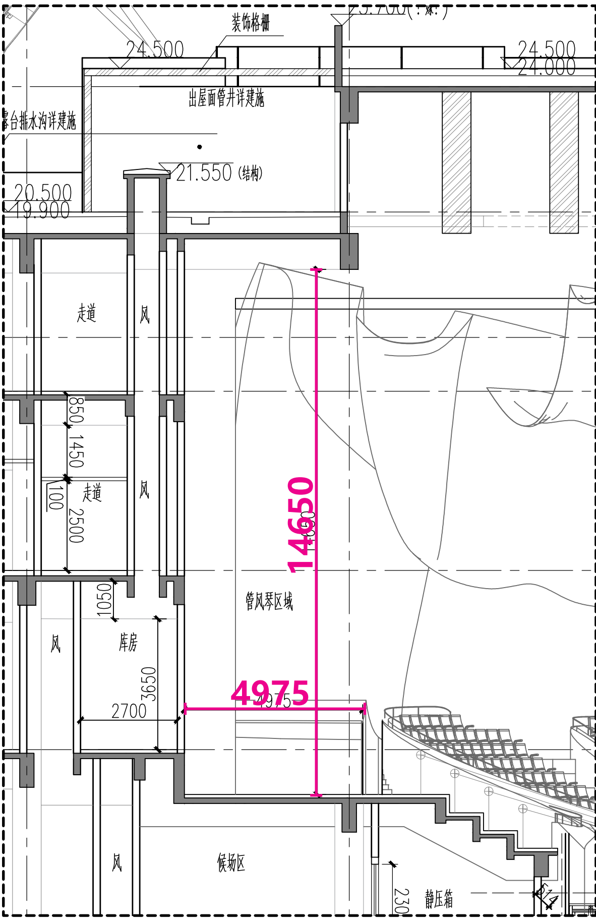
剖立面
