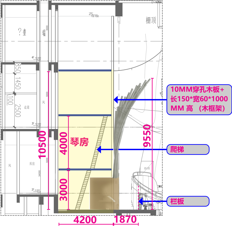
剖立面图
