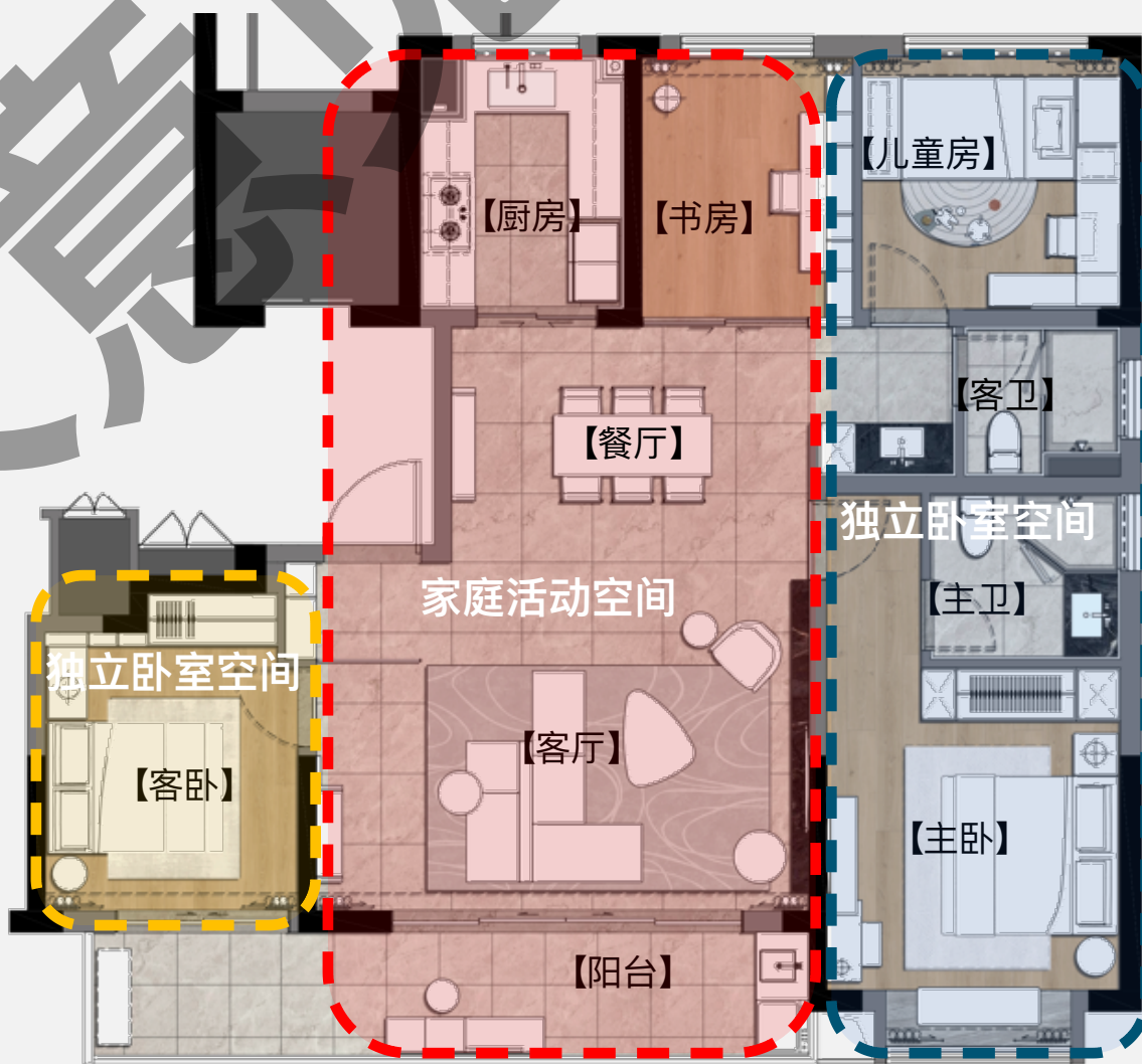
区域划分平面图
