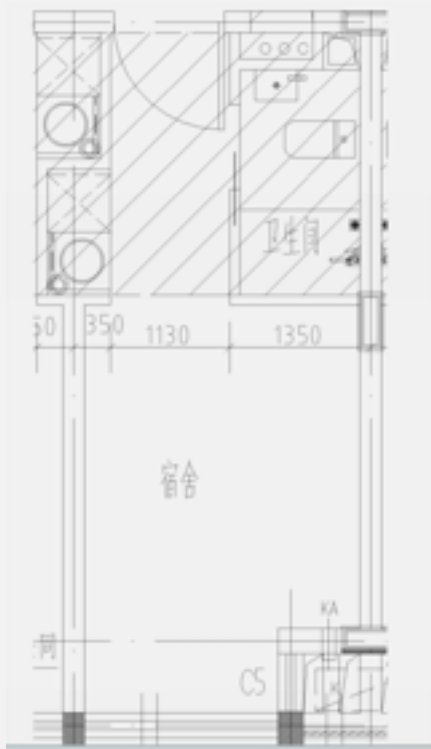
24m² 原始及改造平面图
