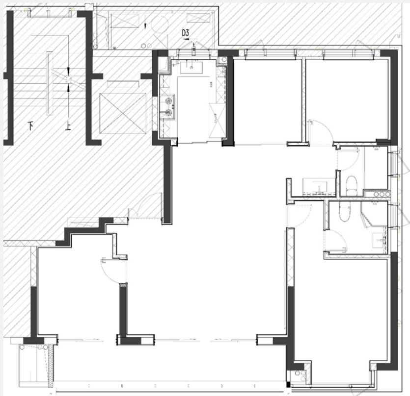
原始平面图
