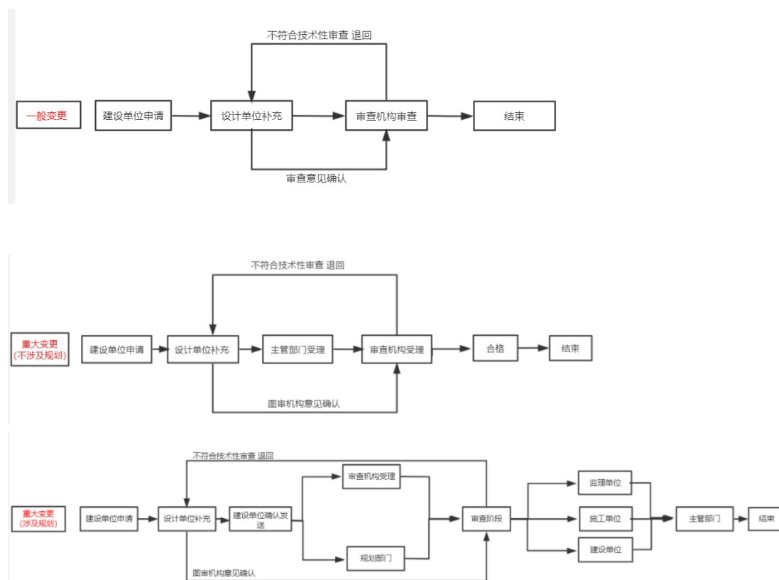
图：变更流程
