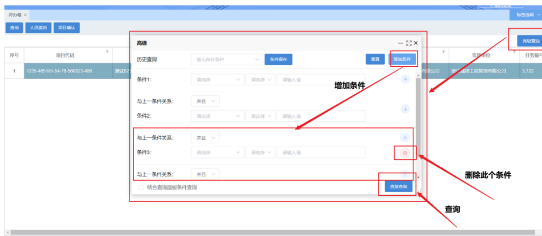
图：查询 2
