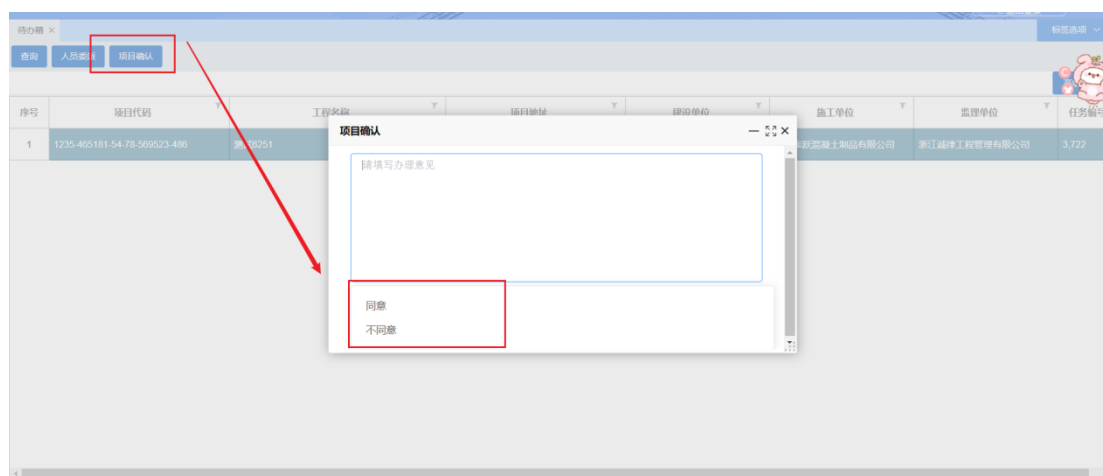
图：项目确认 1
