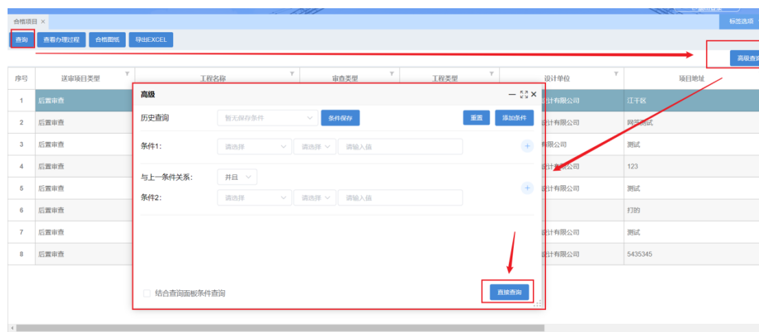
图：查询 1
