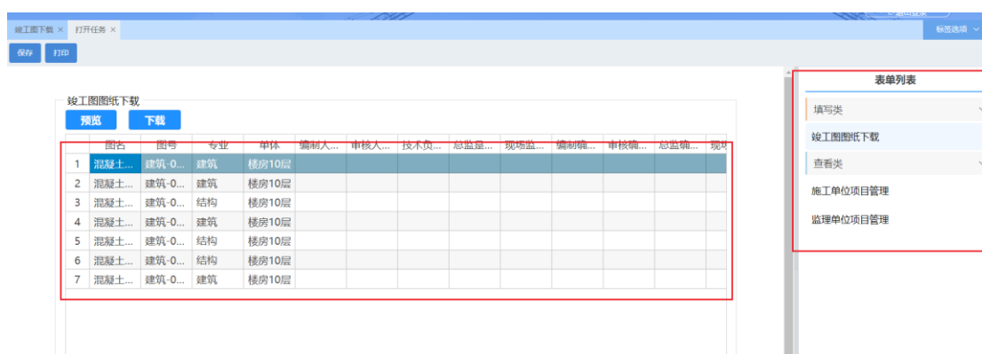
图：显示图纸
