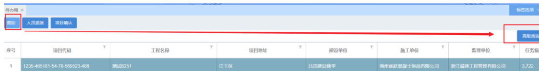
图：待办箱
