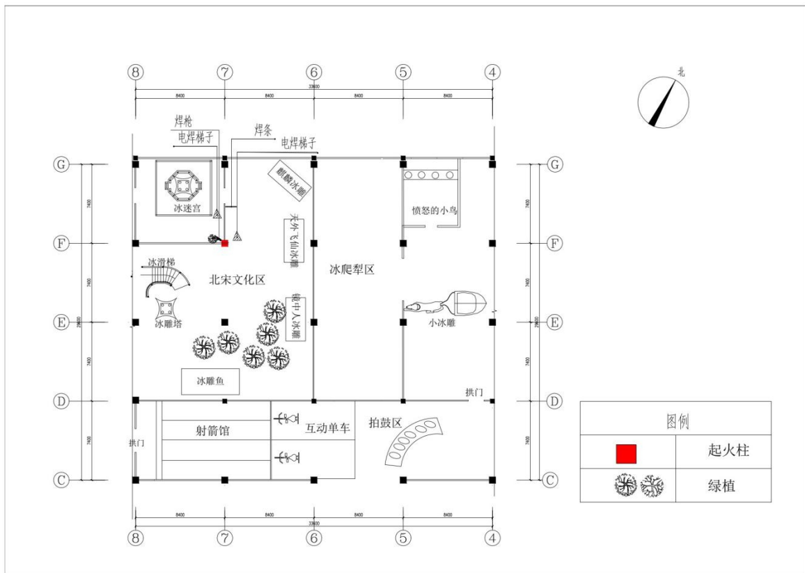
图 2：杭州冰雪大世界事故现场起火部位平面图
