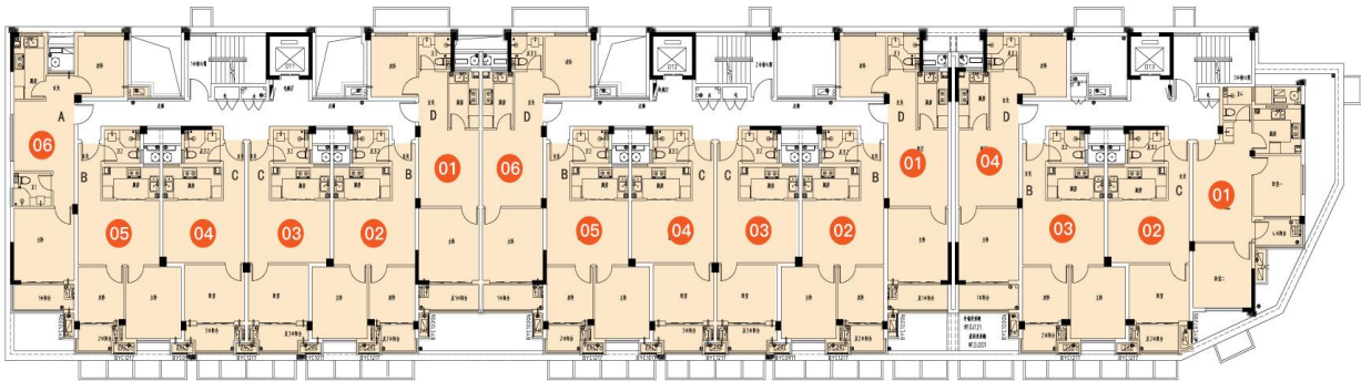
万塘云起公寓12幢2-8层平面图 ( 共8层 )
