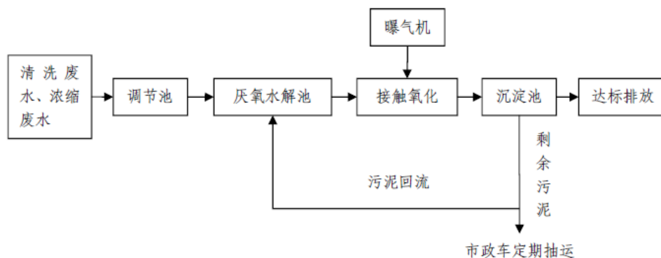
图 1.6-1 废水处理设施处理工艺流程图
