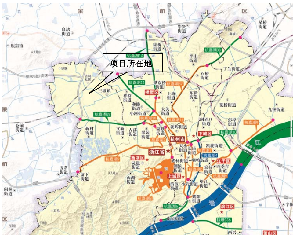
图 4-1 水环境功能区划图
