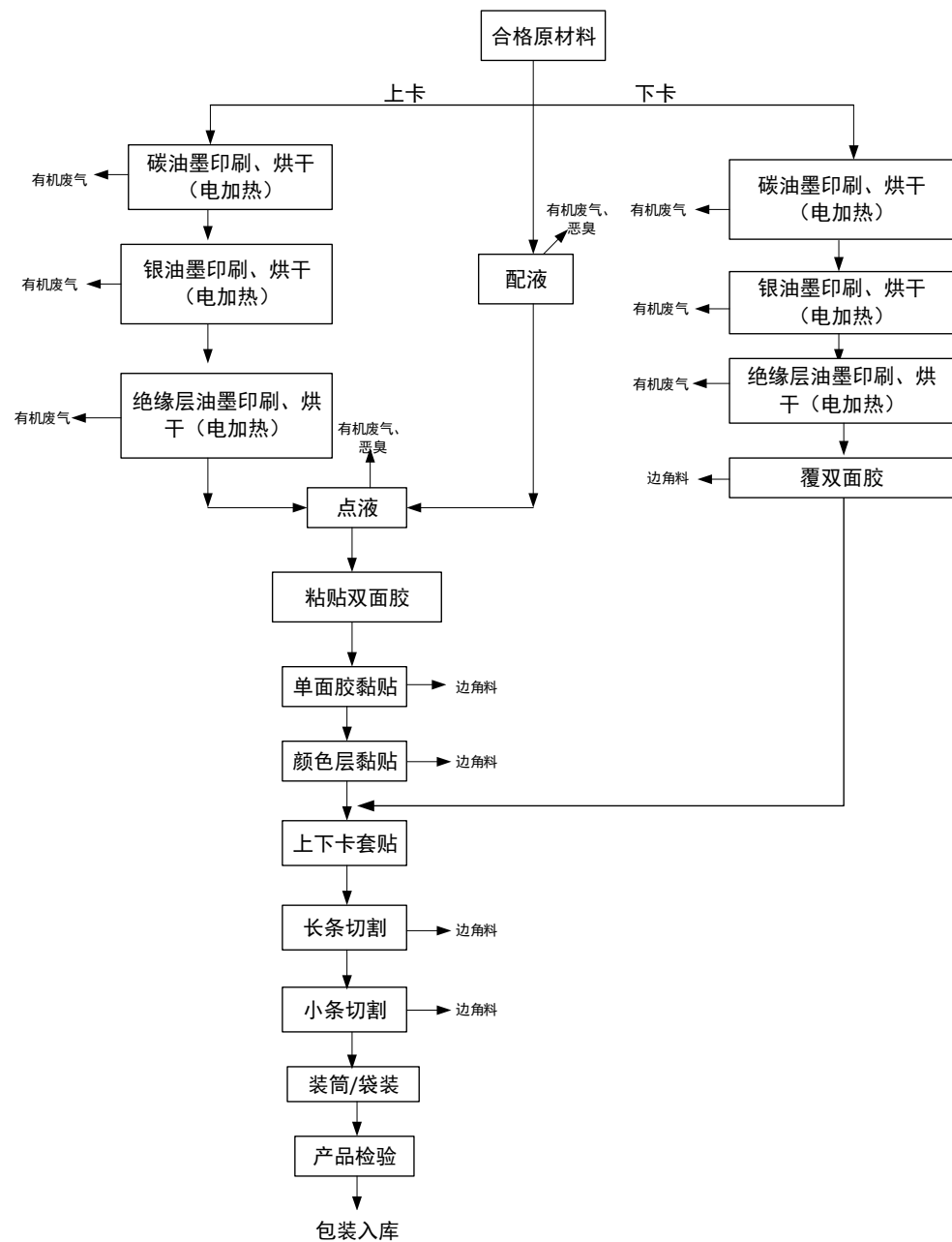
图 5-1 生产工艺及产污流程图
