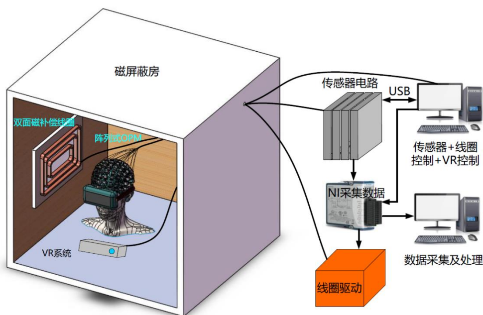
图 4.2-2 脑磁成像实验室布局
