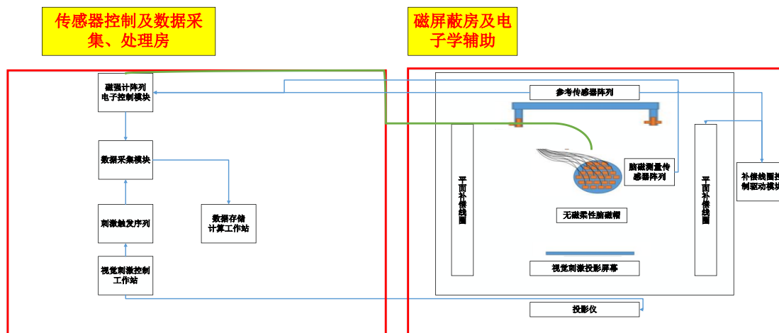
图 4.2-3 脑磁成像实验室主要功能区划分
