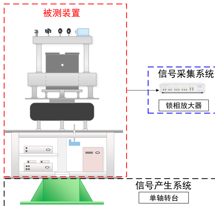
图 4.2-1 测试系统框图
