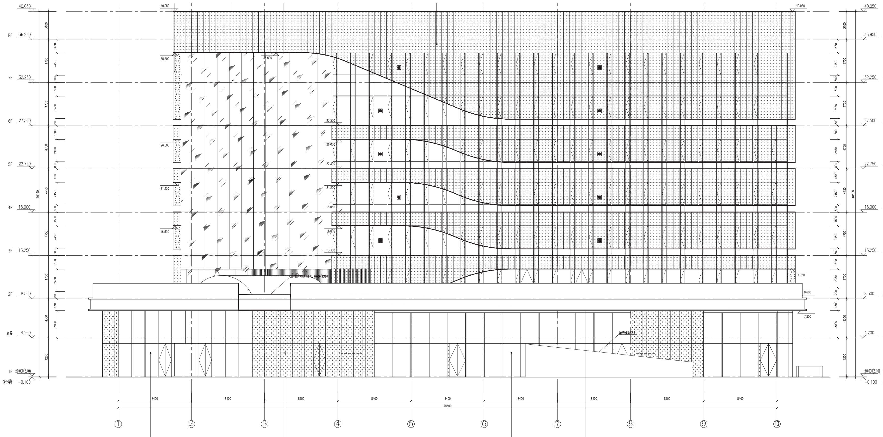
南立面图
