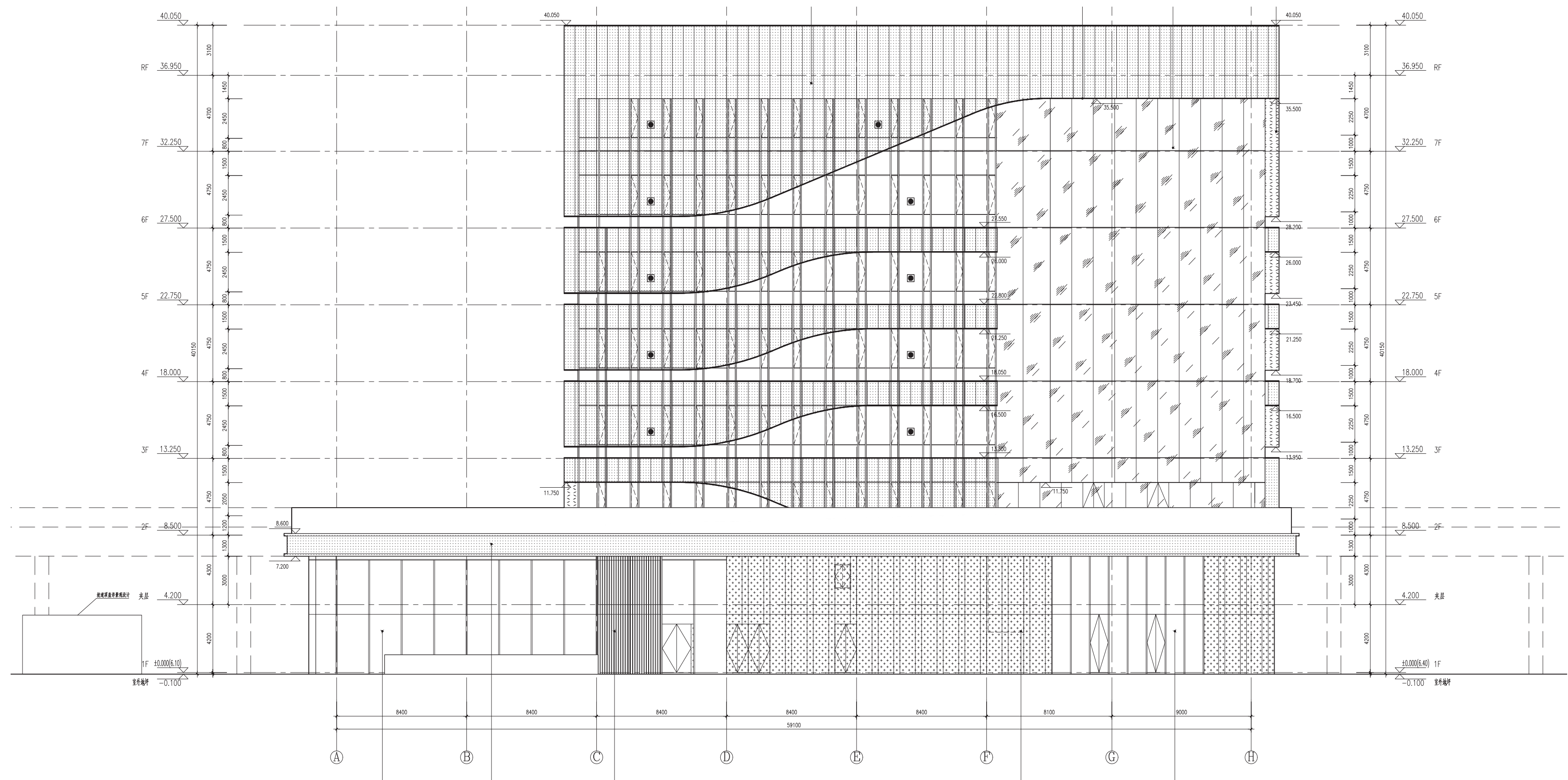
东立面图
