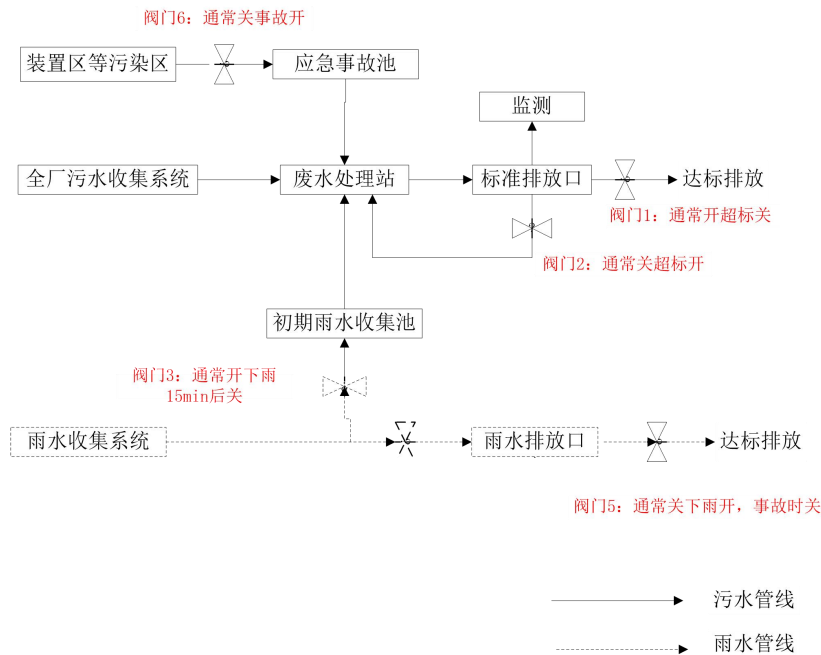
图 7.7-1 全厂排水示意图
