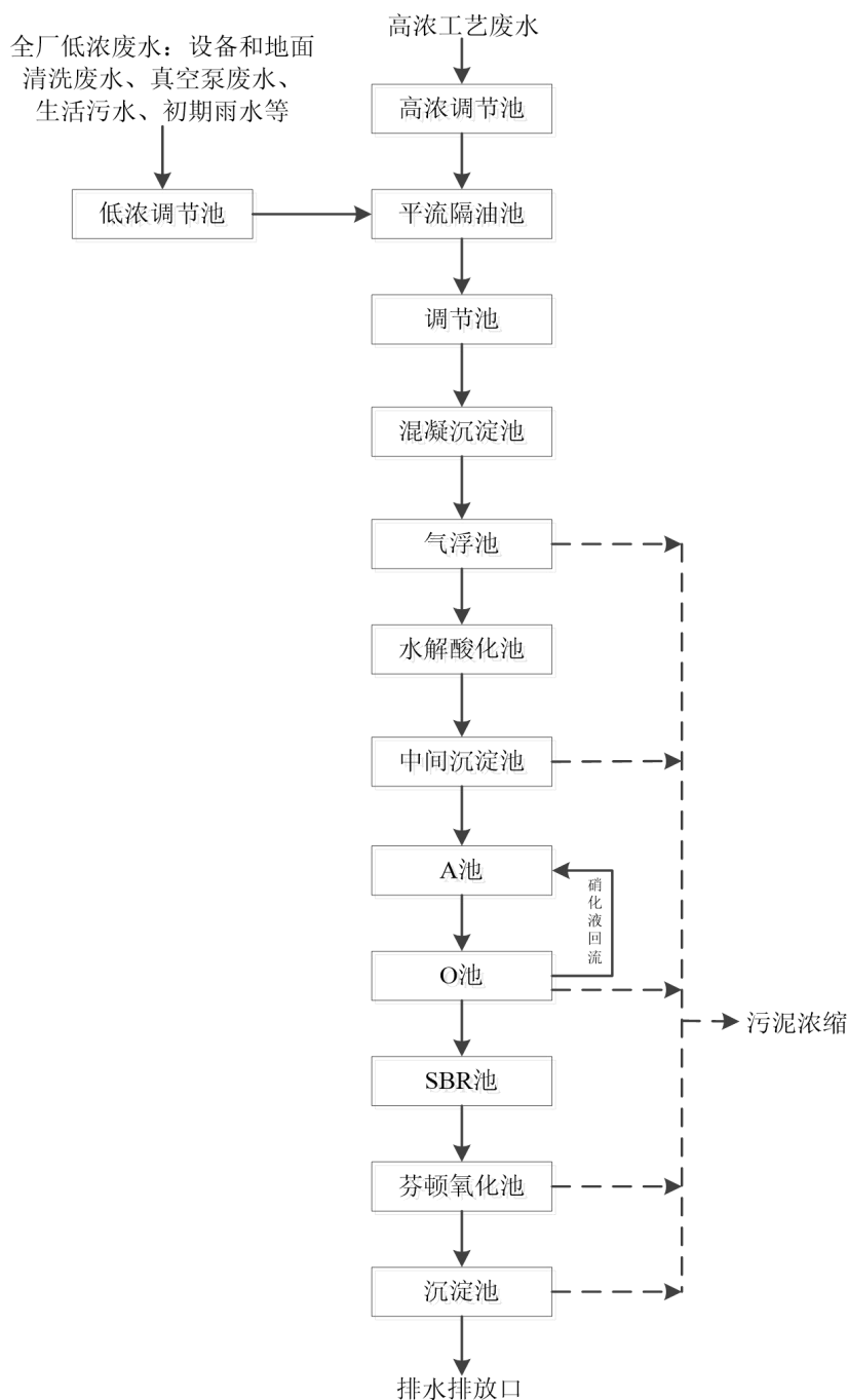
图 8.2-1 废水处理工艺流程
