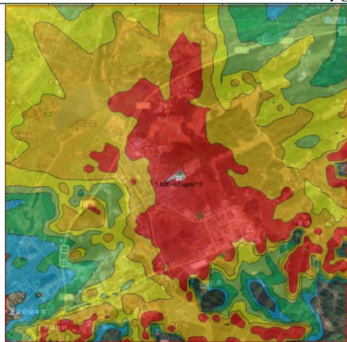
6.2-15NMHC 小时浓度预测结果 (单位: \mu\text{g}/\text{m}^3 )
