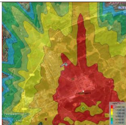
图 6.2-12 硫酸雾小时浓度预测结果 (单位: \mu\text{g}/\text{m}^3 )
