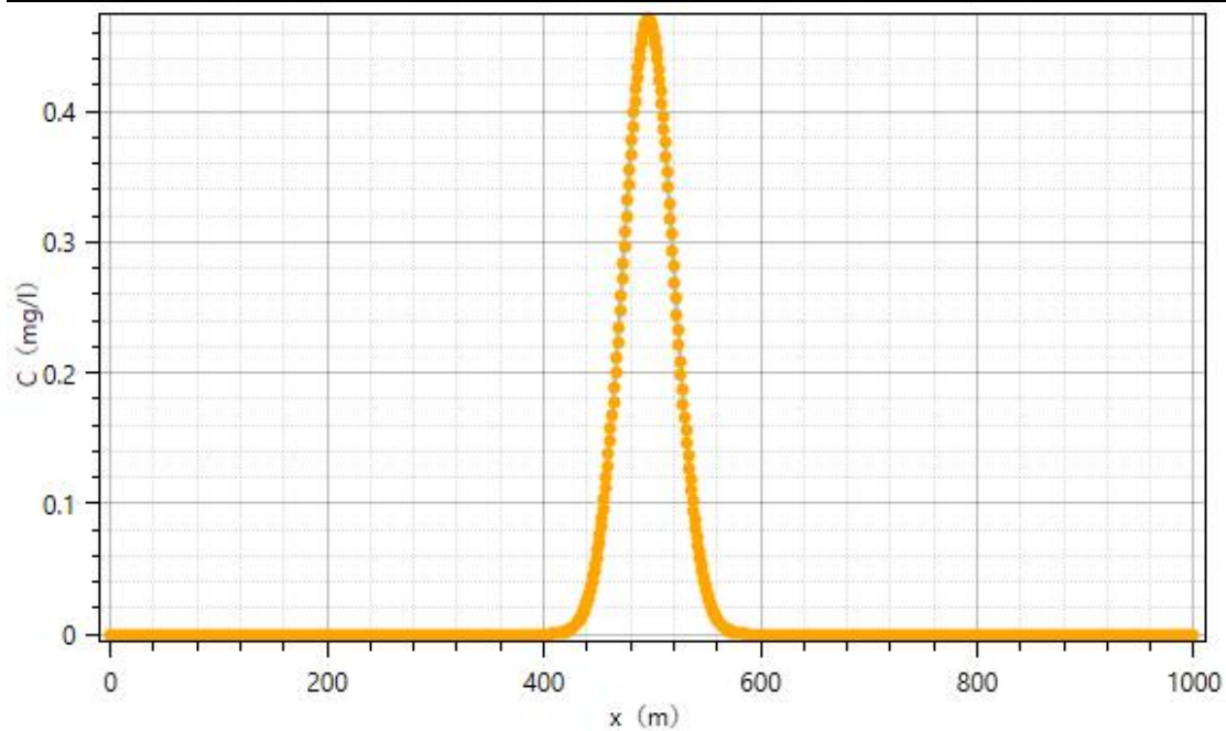
图 6.2-22 泄漏 20 年后耗氧量污染物运移范围图
