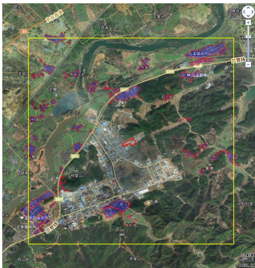
图 6.2.5 大气评价基本信息底图
