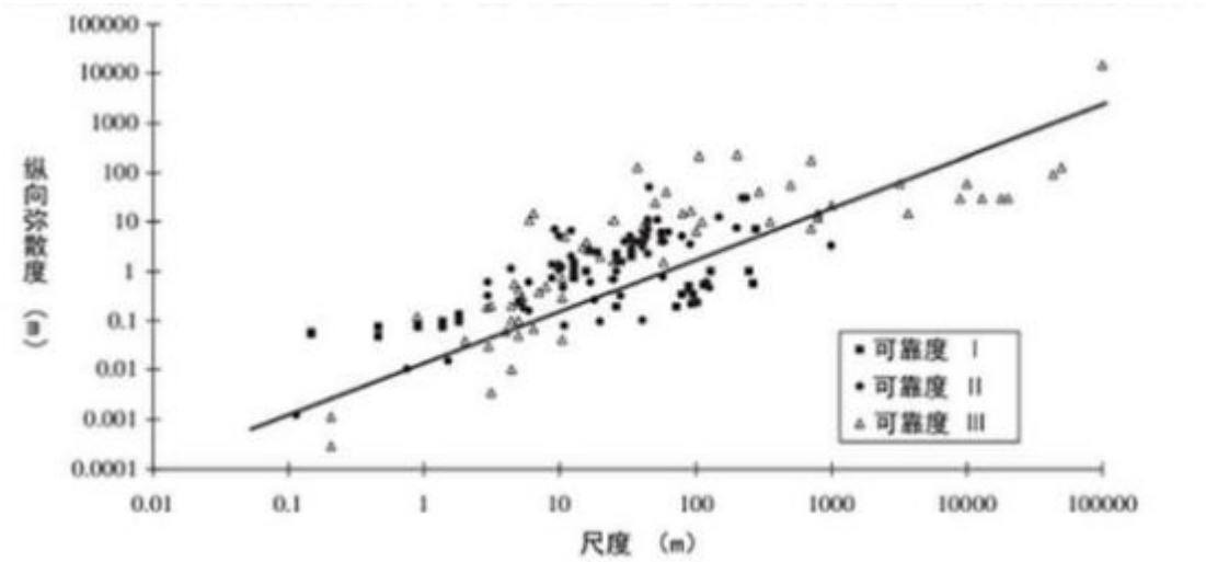
图 6.2-18 松散沉积物的纵向弥散度与研究区域尺度的关系 含水层弥散度类比取值见表 6.2-41。
