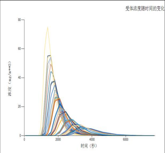
图7.6-2 最不利气象各受体浓度随时间的变化
