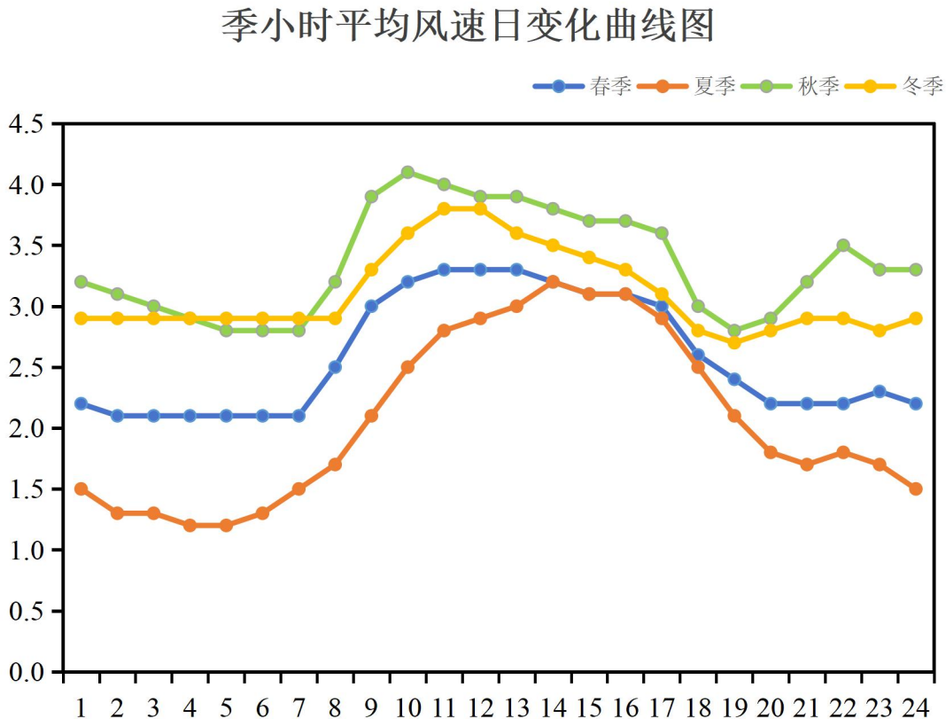
图 6.2-4 江山市季小时平均风速日变化图
