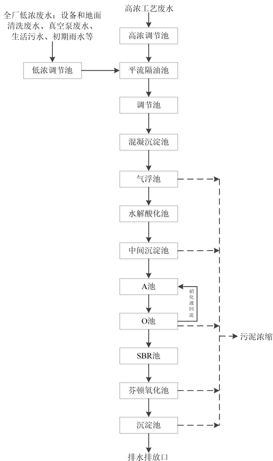
图 3.3-6 废水处理工艺流程图
