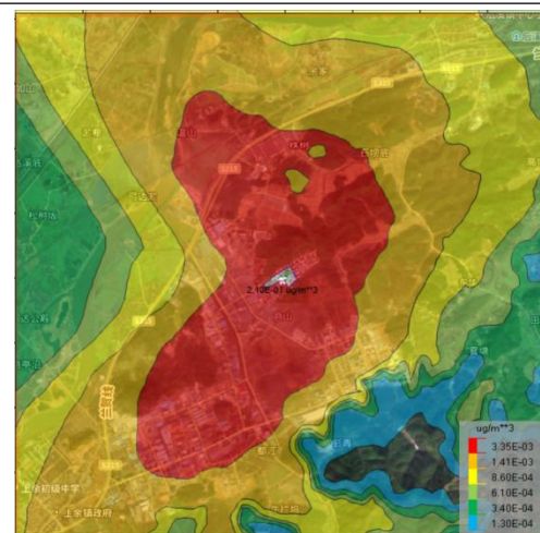
图 6.2-8 乙醛年均浓度预测结果 (单位: \mu\text{g}/\text{m}^3 )
