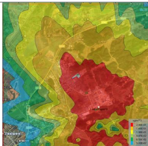
图 6.2-13 硫酸雾日均浓度预测结果 (单位: \mu\text{g}/\text{m}^3 )
