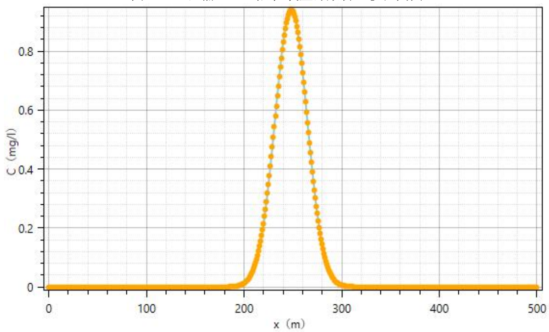
图 6.2-21 泄漏 10 年后耗氧量污染物运移范围图
