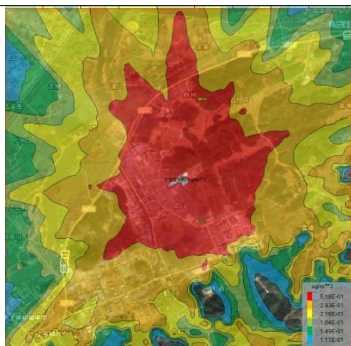
图 6.2-9 丁酮小时浓度预测结果 (单位: \mu\text{g}/\text{m}^3 )
