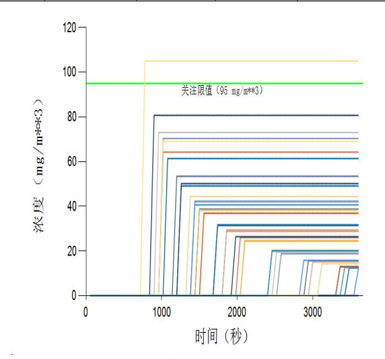
图 7.6-4 最不利气象各受体浓度随时间变化
