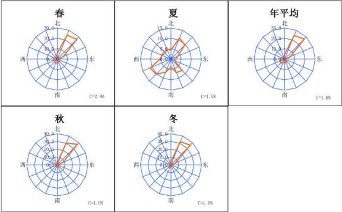
图 6.2-2 江山市各季风向频率玫瑰图
