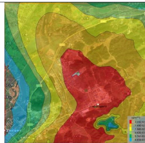
图 6.2-14 硫酸雾年均浓度预测结果 (单位: \mu\text{g}/\text{m}^3 )
