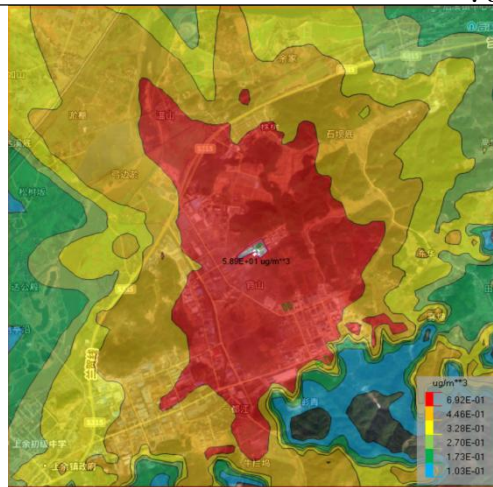
图 6.2-16NMHC 日均浓度预测结果 (单位: \mu\text{g}/\text{m}^3 )
