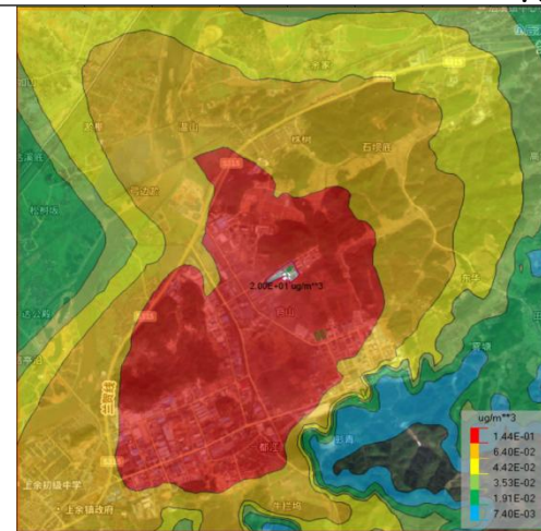
图 6.2-17NMHC 年均浓度预测结果 (单位: \mu\text{g}/\text{m}^3 )
