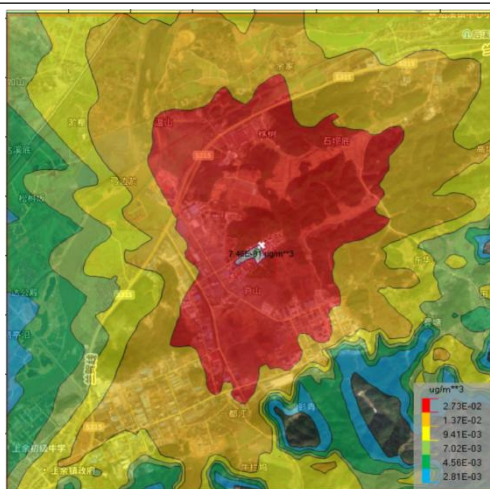
图 6.2-7 乙醛日均浓度预测结果 (单位: \mu\text{g}/\text{m}^3 )
