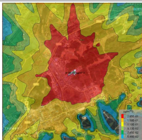
图 6.2-6 乙醛小时浓度预测结果 (单位: \mu\text{g}/\text{m}^3 )
