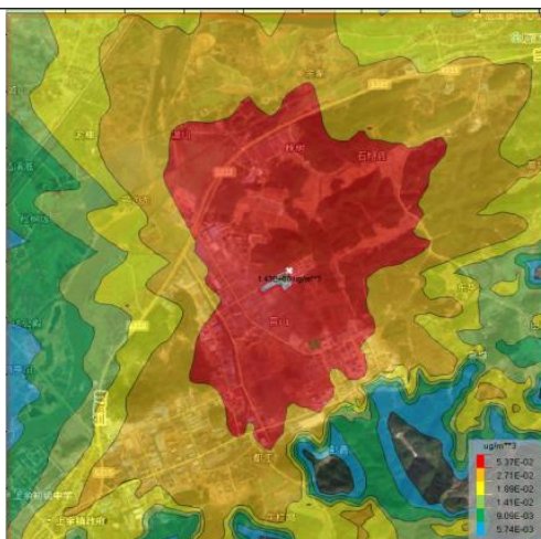
图 6.2-10 丁酮日均浓度预测结果 (单位: \mu\text{g}/\text{m}^3 )
