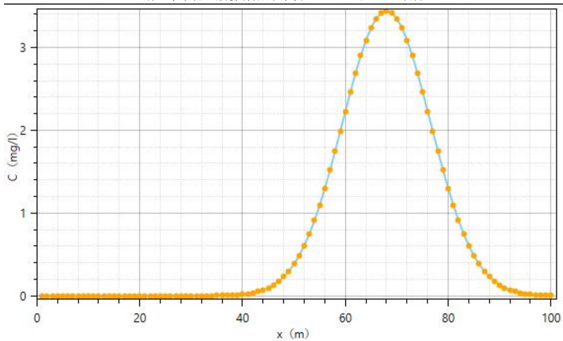
图 6.2-20 泄漏 1000d 后耗氧量污染物运移范围图
