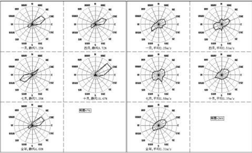
图 5.1-1 衢州市风向频率玫瑰图 图 5.1-2 衢州市风速频率玫瑰图
