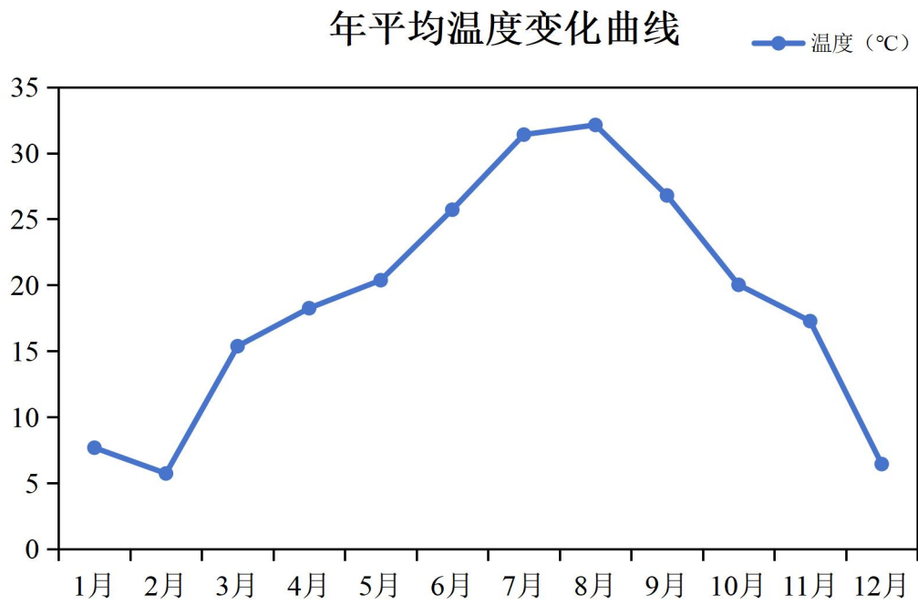
图 6.2-1 江山市年平均温度变化图
