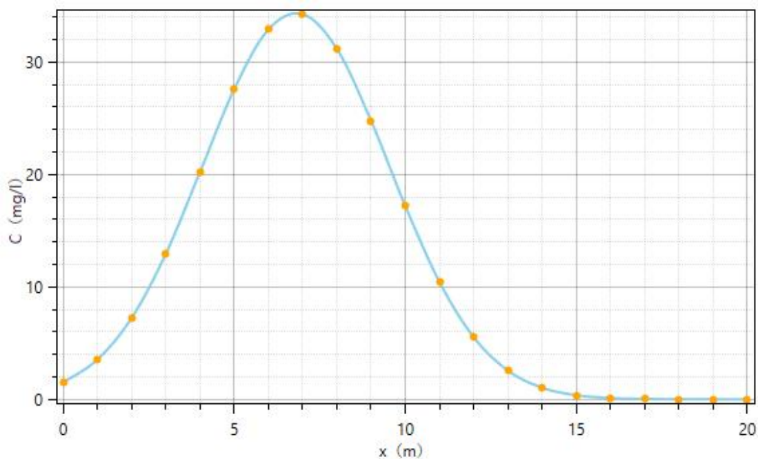
图 6.2-19 泄漏 100d 后耗氧量污染物运移范围图
