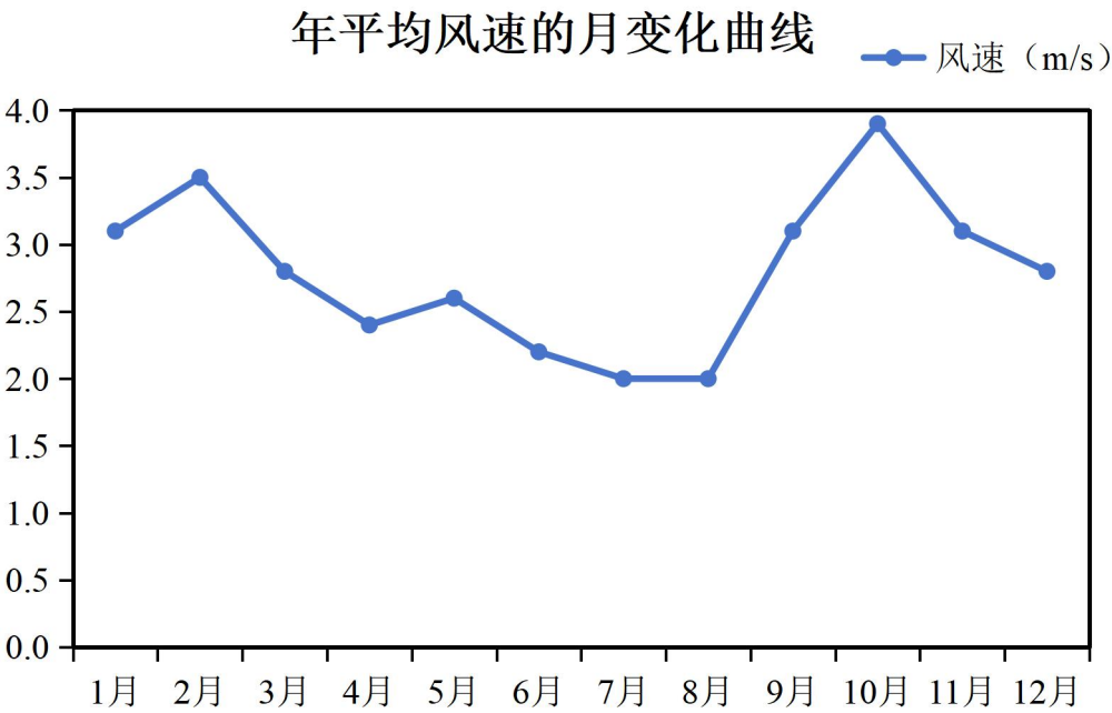
图 6.2-3 江山市年平均风速变化图
