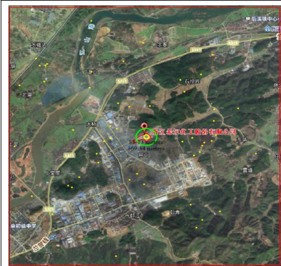
图7.6-1 乙醛在最不利气象条件下预测结果图
