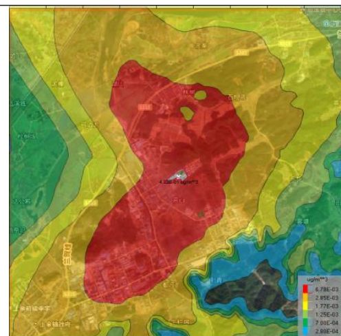
图 6.2-11 丁酮年均浓度预测结果 (单位: \mu\text{g}/\text{m}^3 )
