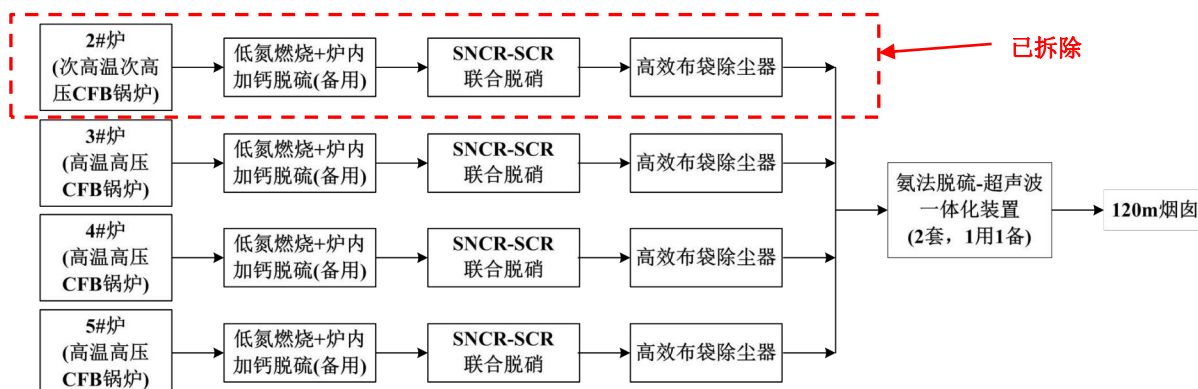
图 3.3-1 现有锅炉烟气治理流程图
