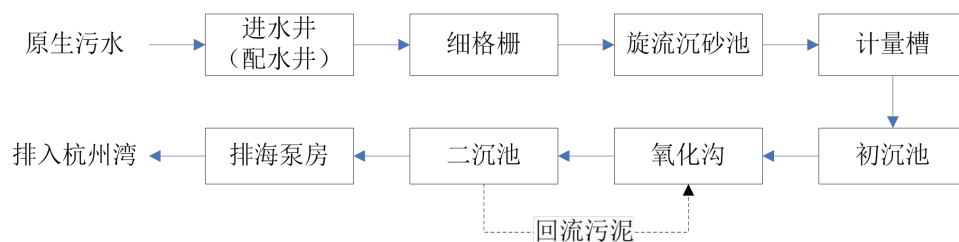
图 5.3-1 嘉兴污水处理一期工程污水处理工艺流程图
