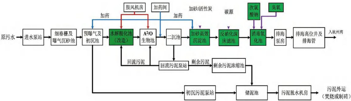
图 5.3-4 嘉兴污水处理二期工程提标改造后工艺流程图
