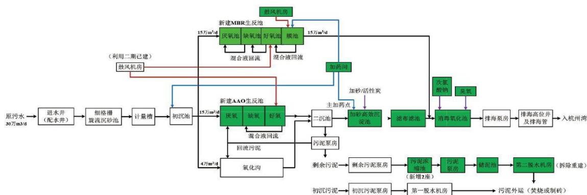
图 5.3-3 嘉兴污水处理一期工程提标改造后工艺流程图
