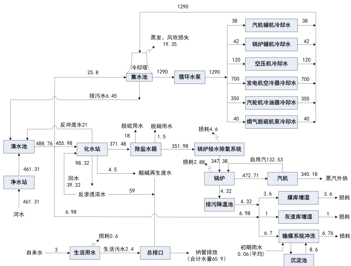
图 4.2-1 技改项目水平衡图 (t/h)
