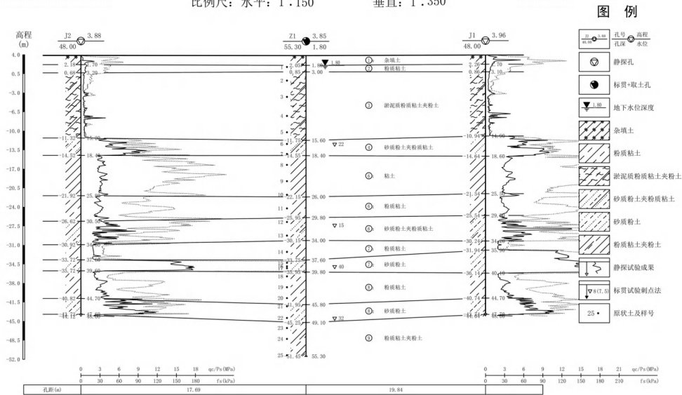
图 6.3-1 典型工程地质剖面图
