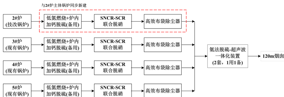
图 7.1-1 锅炉烟气治理工艺流程
