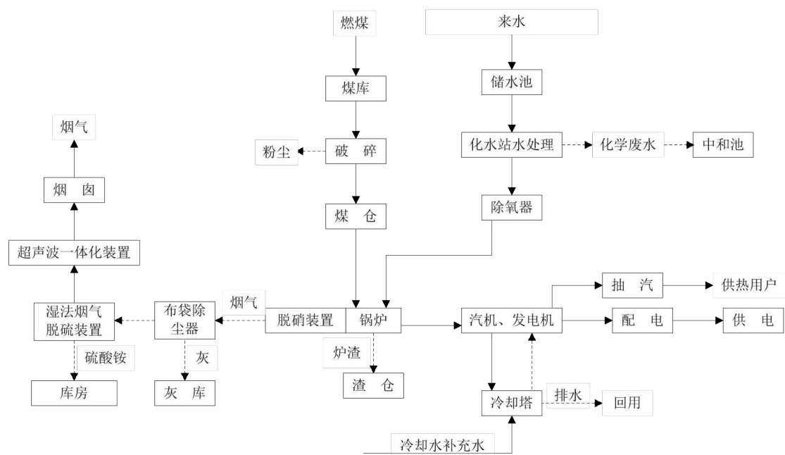
图 3.2-1 现有工艺流程图
