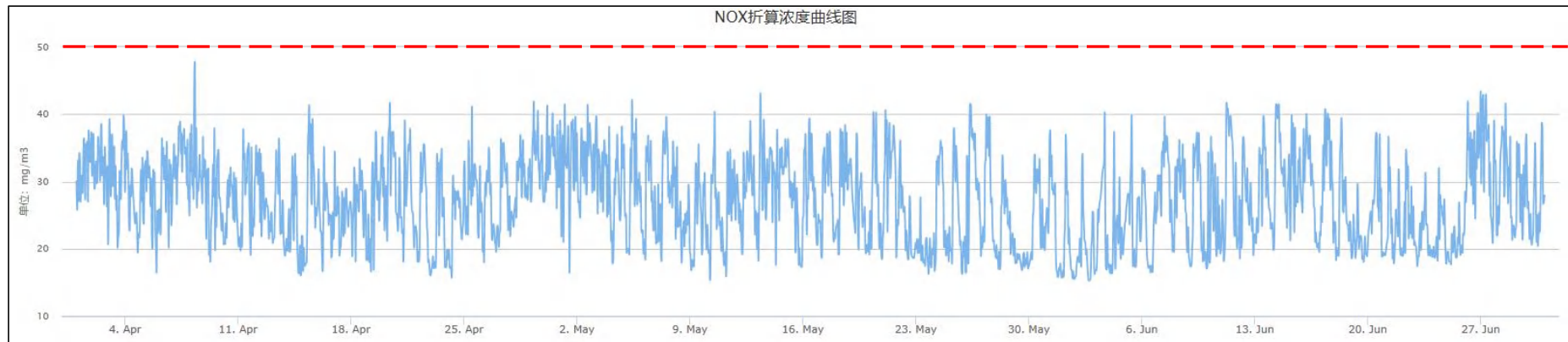
图 7.1-9 现有工程 NO x 折算浓度曲线图(2022.4.1~6.30)
