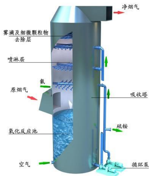
图 7.1-3 氨法脱硫塔示意图
