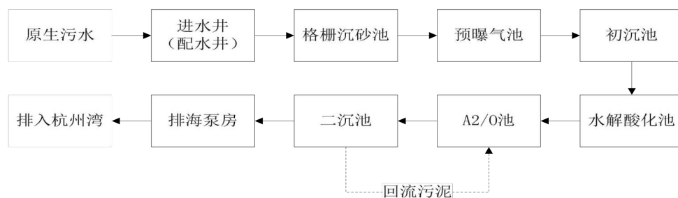
图 5.3-2 嘉兴污水处理二期工程污水处理工艺流程图
