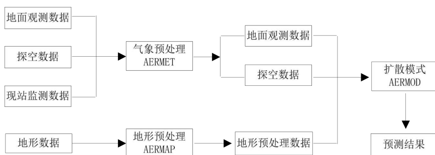
图 6.1-5 AERMOD 模式系统流程
