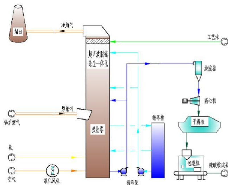
图 7.1-2 氨法脱硫+超声波一体化技术工艺流程示意图
