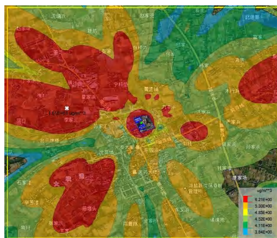
图 6.1-7 NO 2 小时平均浓度分布图
