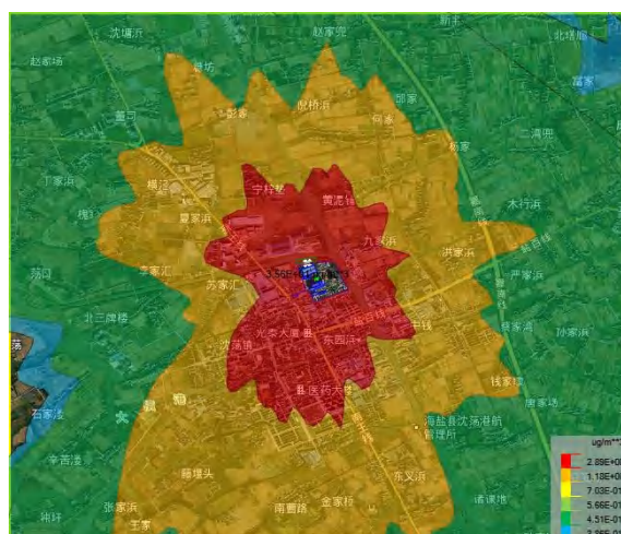
图 6.1-13 \text{PM}_{10} 日平均浓度分布图
