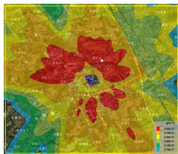
图 6.1-11 SO 2 日平均浓度分布图
