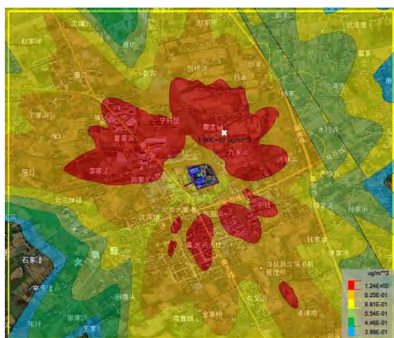
图 6.1-12 \text{NO}_2 日平均浓度分布图
