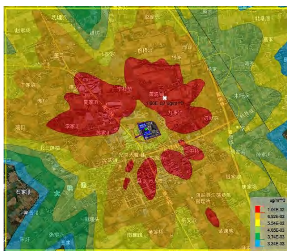
图 6.1-15 氟化物日平均浓度分布图
