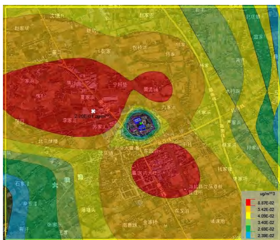
图 6.1-18 SO 2 年均浓度分布图
