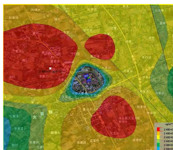
图 6.1-29 NO 2 年均浓度等值线图
