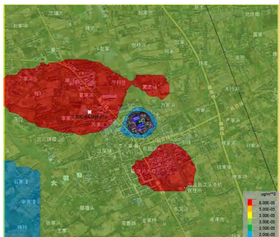
图 6.1-22 Hg 年均浓度分布图
