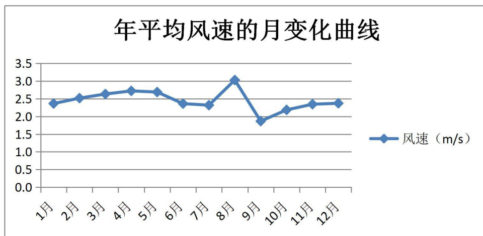
图 6.1-2 年平均风速月变化曲线图
