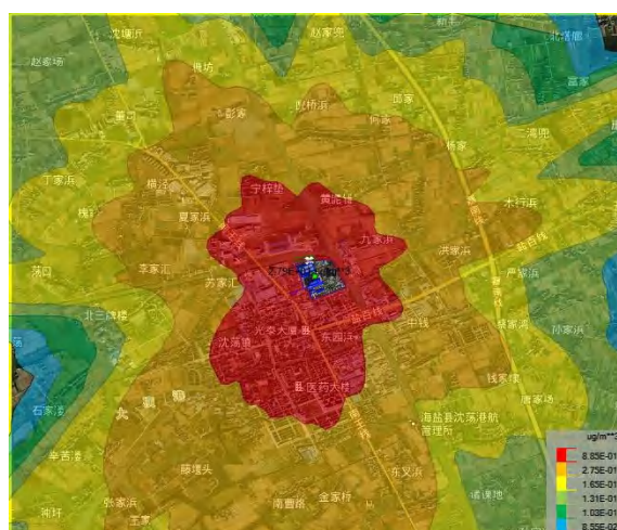
图 6.1-17 TSP 日平均浓度分布图
