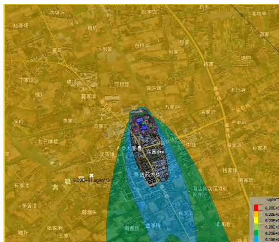
图 6.1-27 PM 2.5 保证率日均浓度分布图
