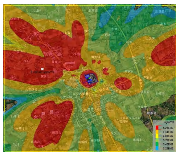
图 6.1-9 氟化物小时平均浓度分布图
