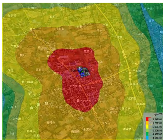
图 6.1-20 PM 10 年均浓度分布图
