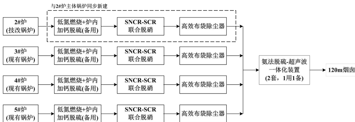
图 4.3-1 锅炉烟气治理工艺流程简图
