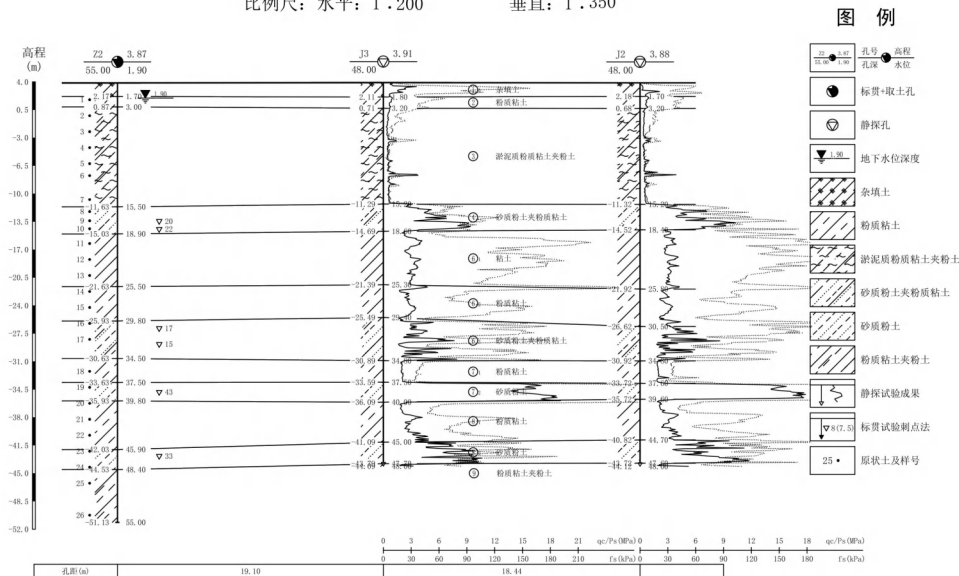
工程地质剖面图 1--1'
