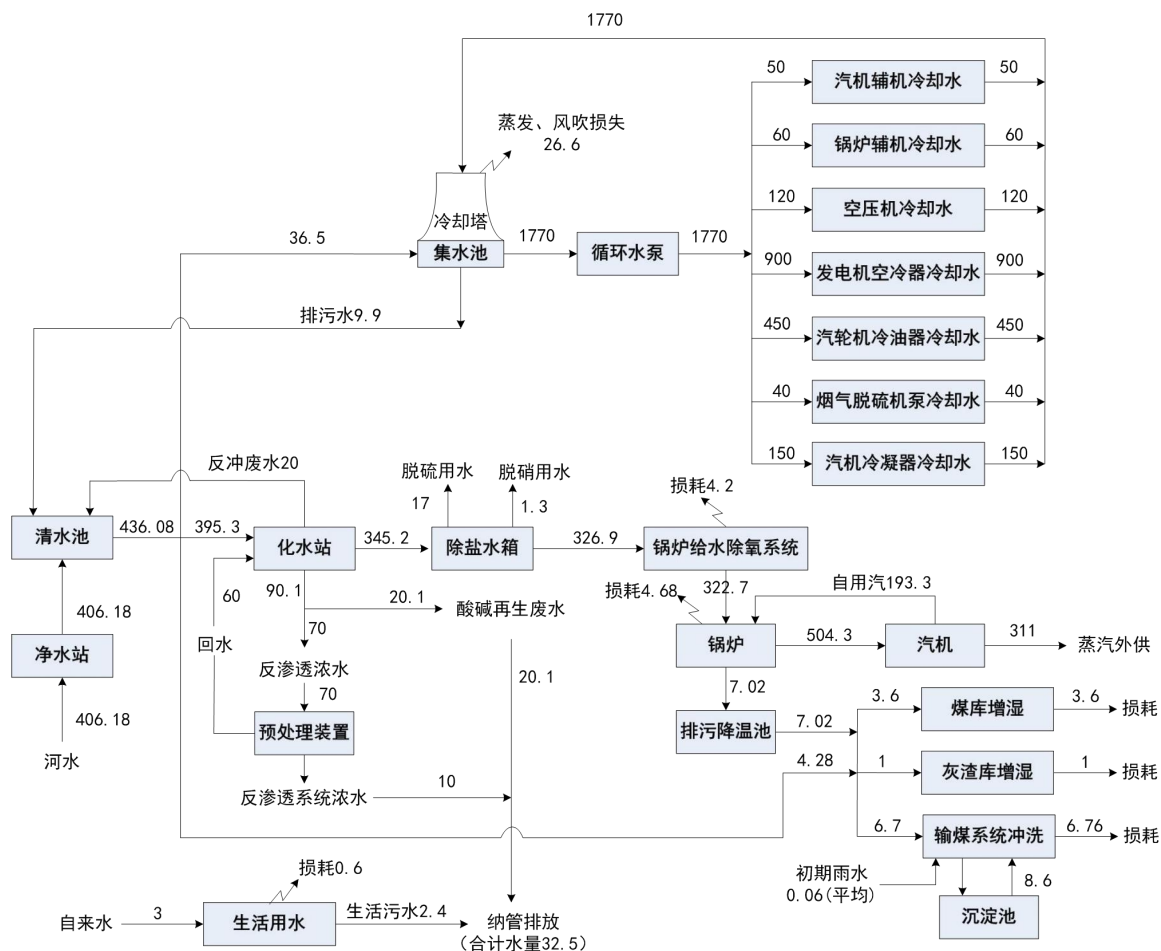
图 3.2-2 现有工程水平衡图 (t/h)
