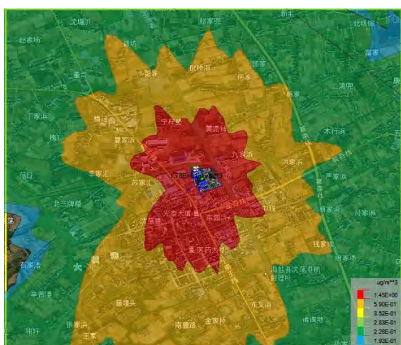
图 6.1-14 \text{PM}_{2.5} 日平均浓度分布图
