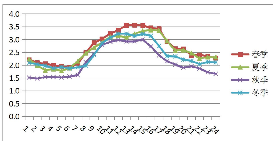
图 6.1-3 年平均风速月变化曲线图
