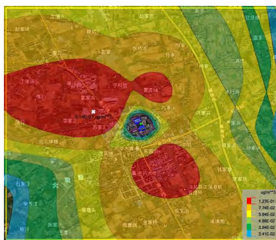
图 6.1-19 NO 2 年均浓度分布图
