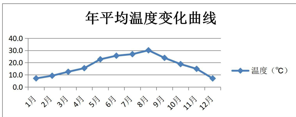
图 6.1-1 年平均温度月变化曲线图
