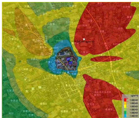
图 6.1-24 SO 2 保证率日均浓度分布图
