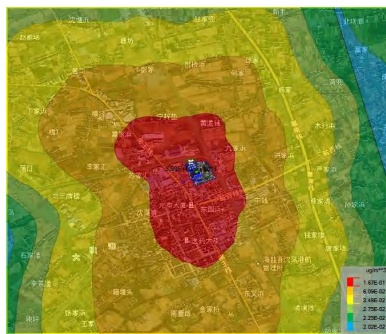
图 6.1-21 PM 2.5 年均浓度分布图
