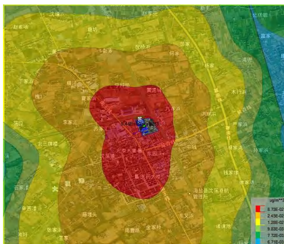
图 6.1-23 TSP 年均浓度分布图
