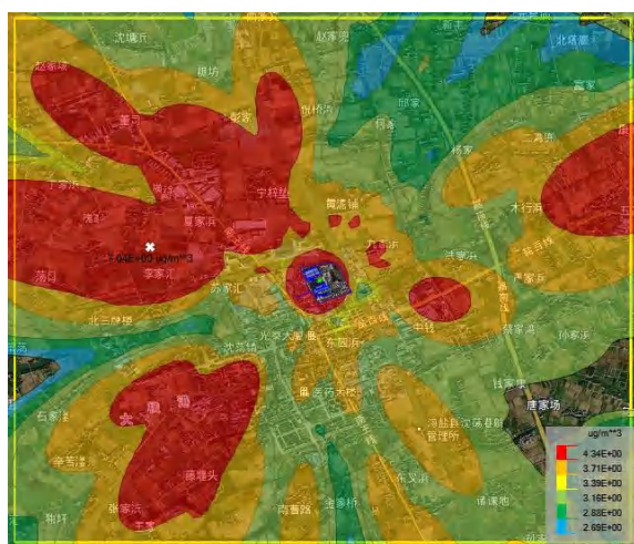
图 6.1-6 SO 2 小时平均浓度分布图
