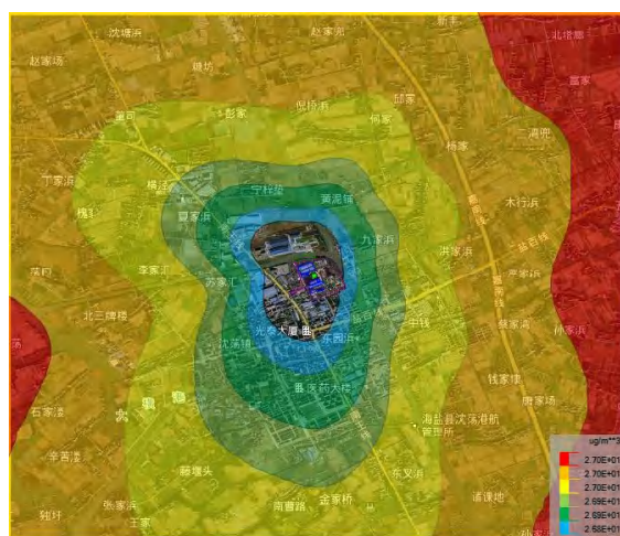
图 6.1-31 PM 2.5 年均浓度等值线图
