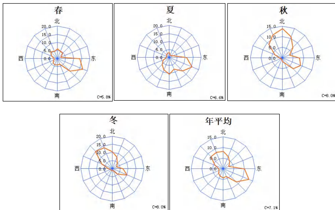
图 6.1-4 各季及全年风频玫瑰图
