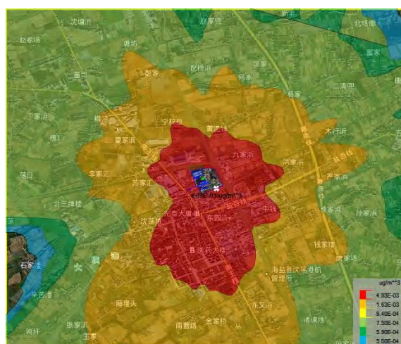
图 6.1-16 \text{HCl} 日平均浓度分布图
