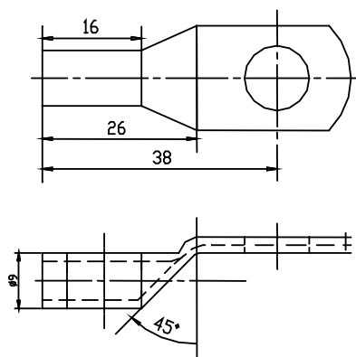
连接线夹
