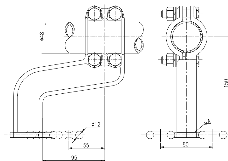
长定位双环
