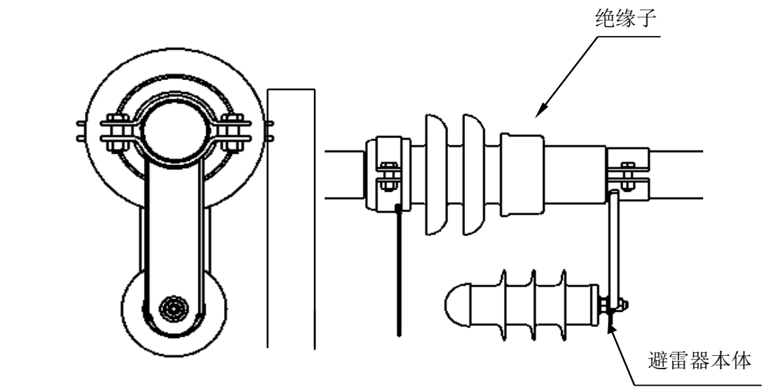
带串联间隙金属氧化物避雷器安装示意图
