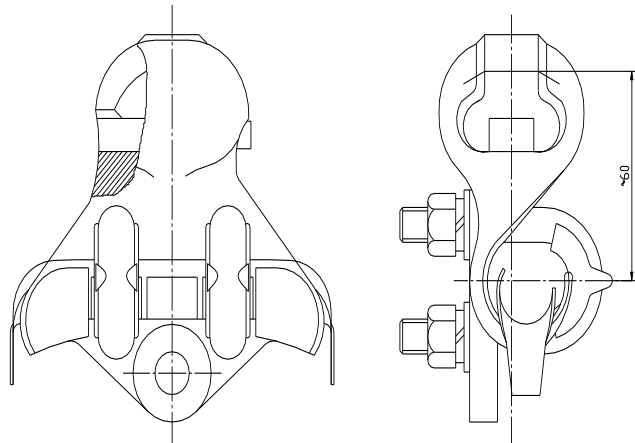
杵座鞍子
