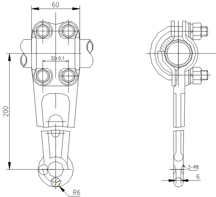
长定位环
