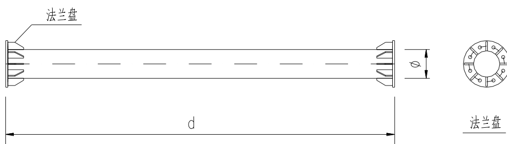
横梁直段外形示意图
