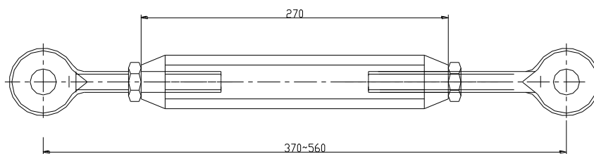
调整螺栓
