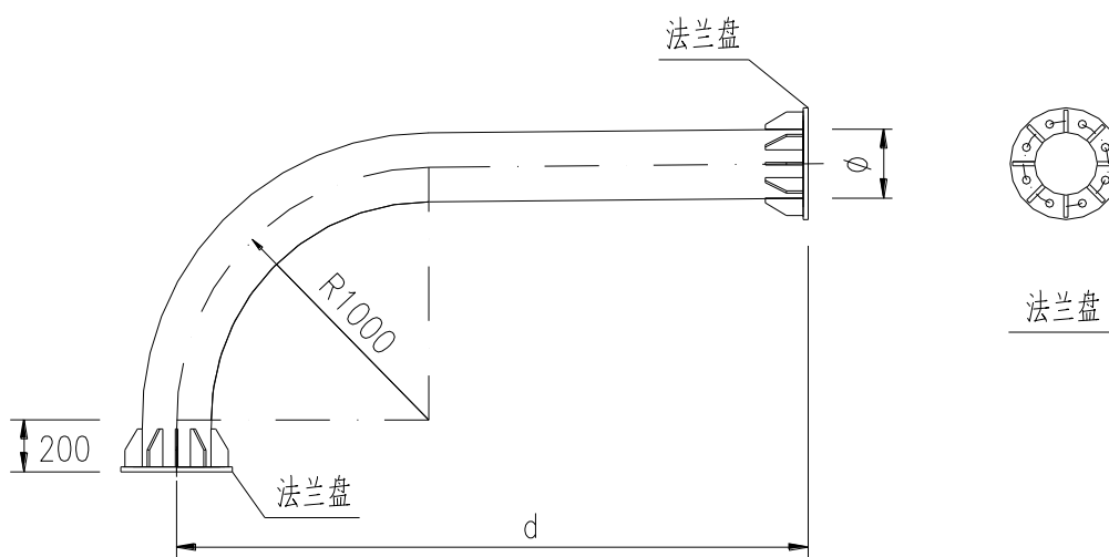
横梁弯段外形示意图
