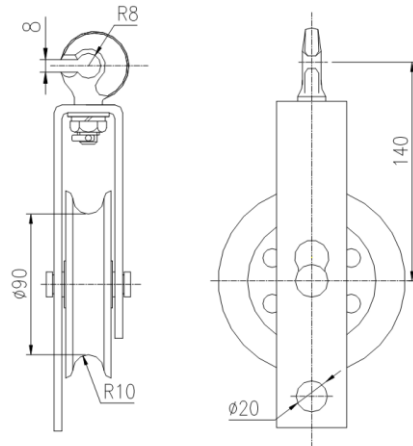
悬吊滑轮
