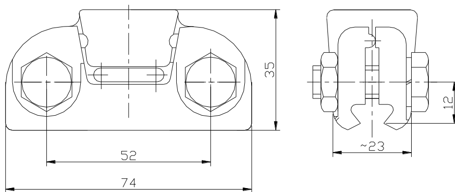
定位线夹
