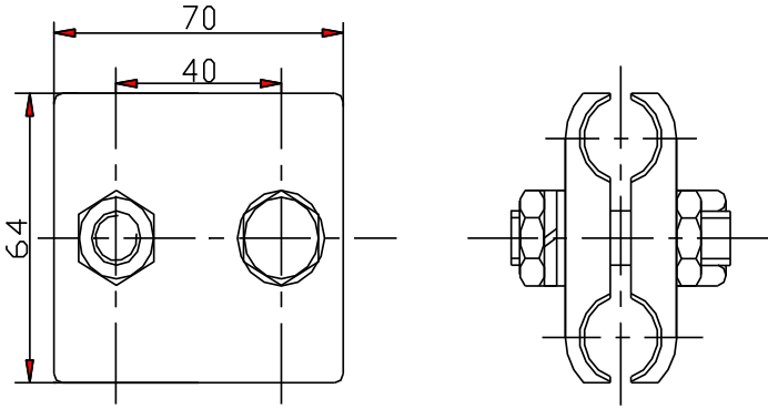
电连接线夹
