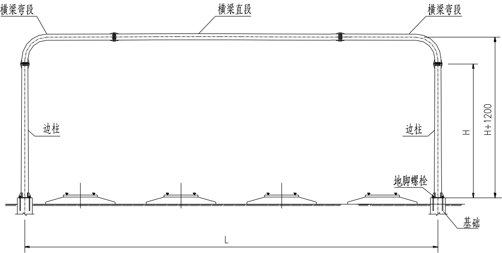
门形支架结构示意图
