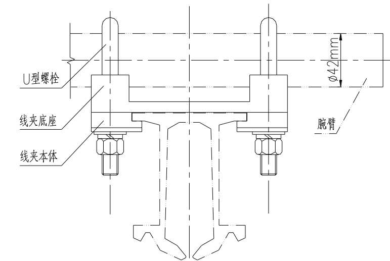
C 型汇流排定位线夹（仅为示意）
