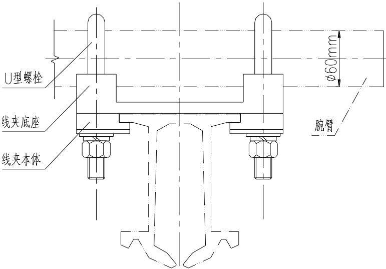
D 型汇流排定位线夹（仅为示意）
