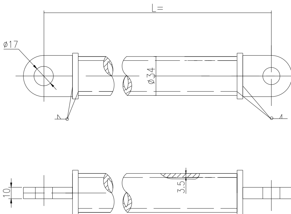
定位管支撑
