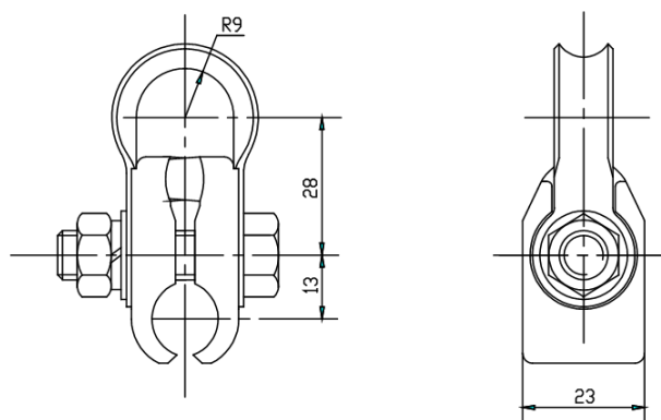
承力索吊弦线夹
