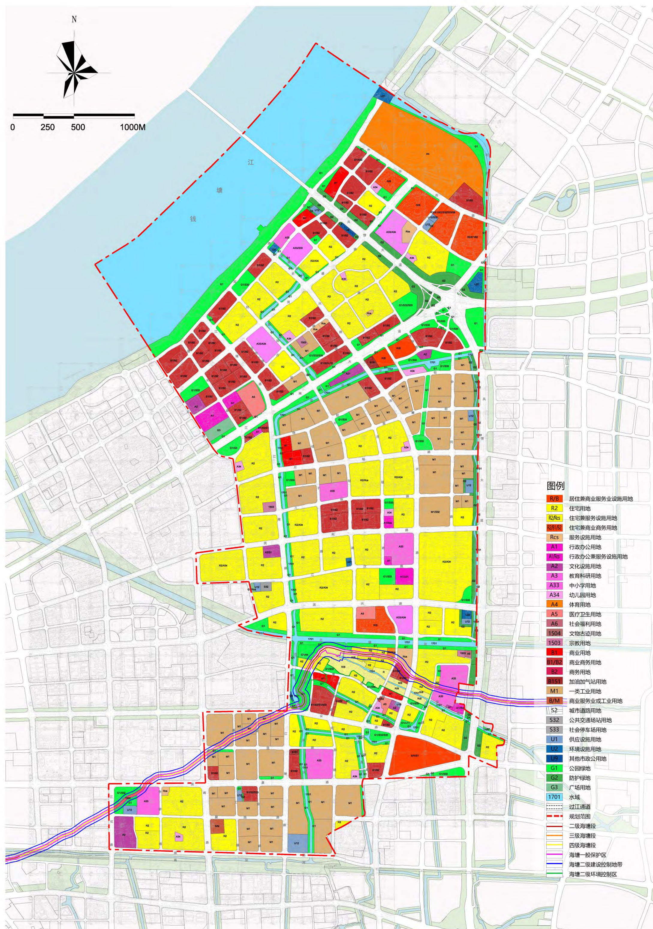
用地功能规划图
