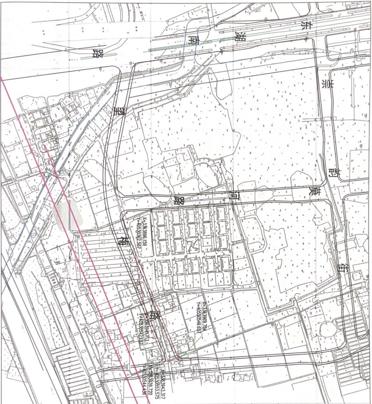
建设用地规划红线图
