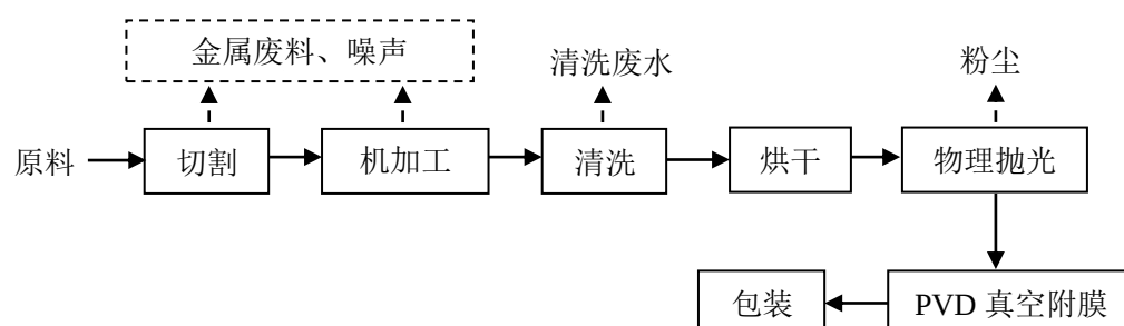
图 1-1 工艺流程示意图
