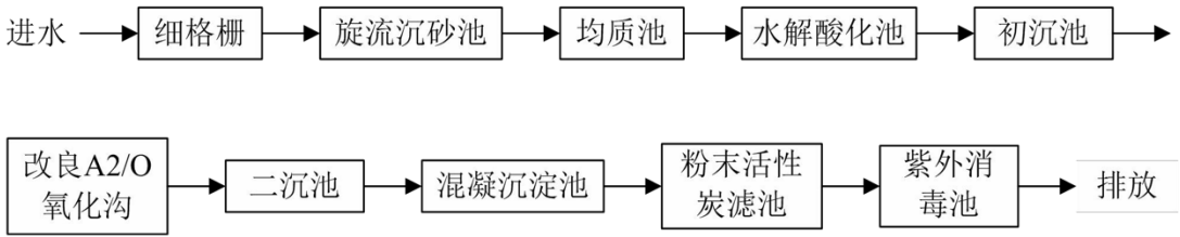
图 7-1 嵊新污水处理厂二期工程工艺流程图
