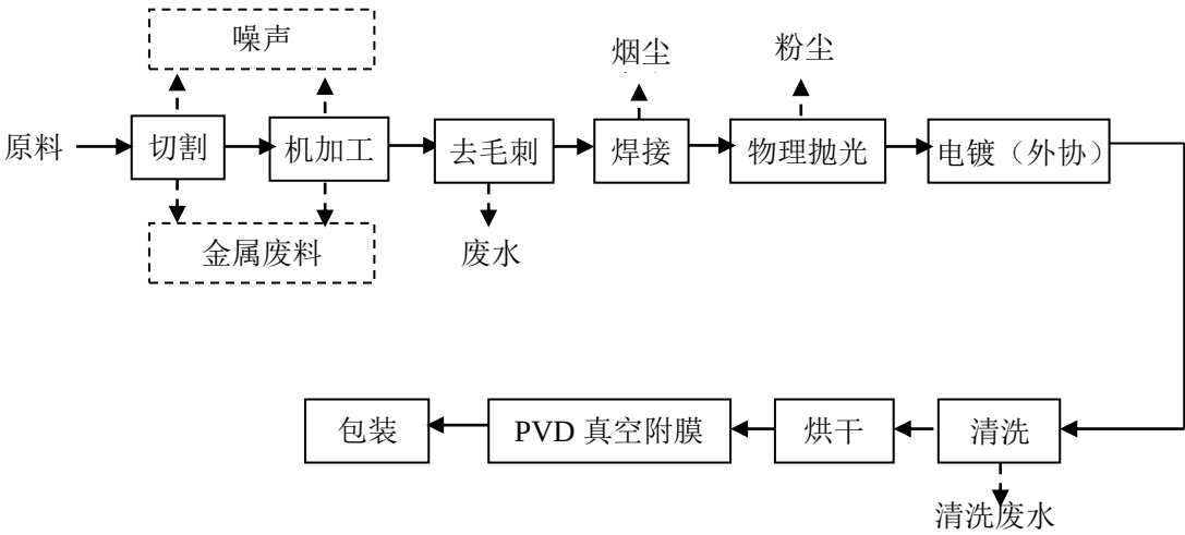
图 5-1 项目生产工艺流程图
