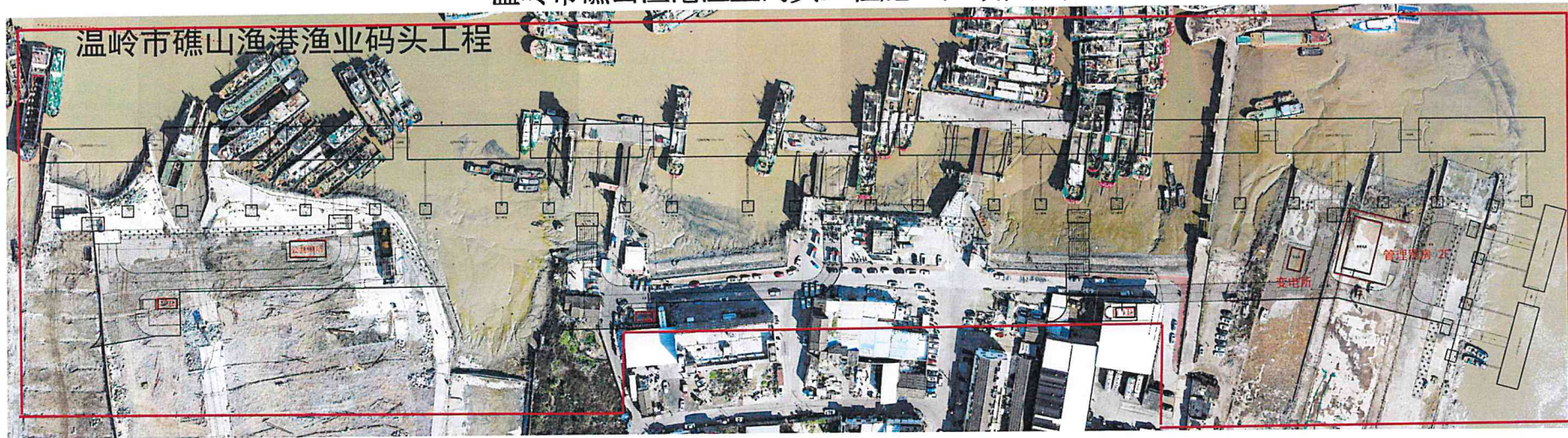
温岭市礁山渔港渔业码头工程施工区域位置图
