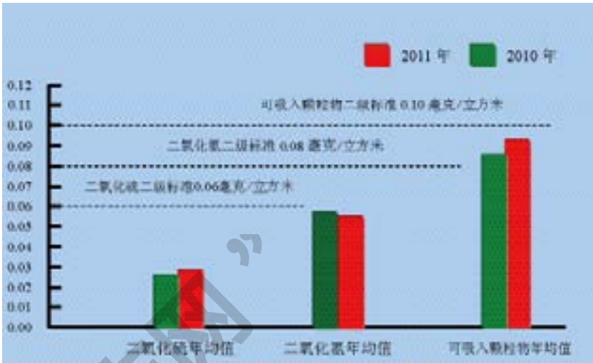
2011年鹿城区环境空气污染物年均值图
