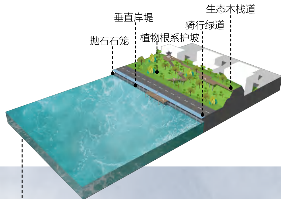
直立式岸带
