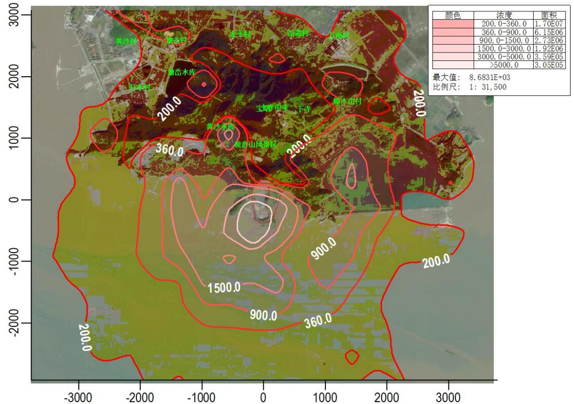
图4-5 非正常工况下粉尘小时最大落地浓度预测图
