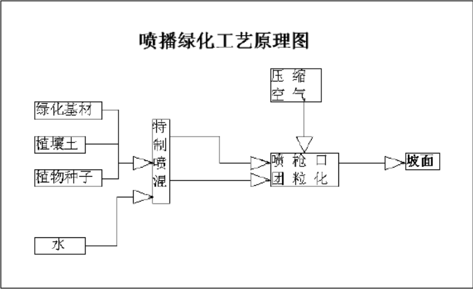
专项图1-4 厚层基材喷播绿化工艺原理
