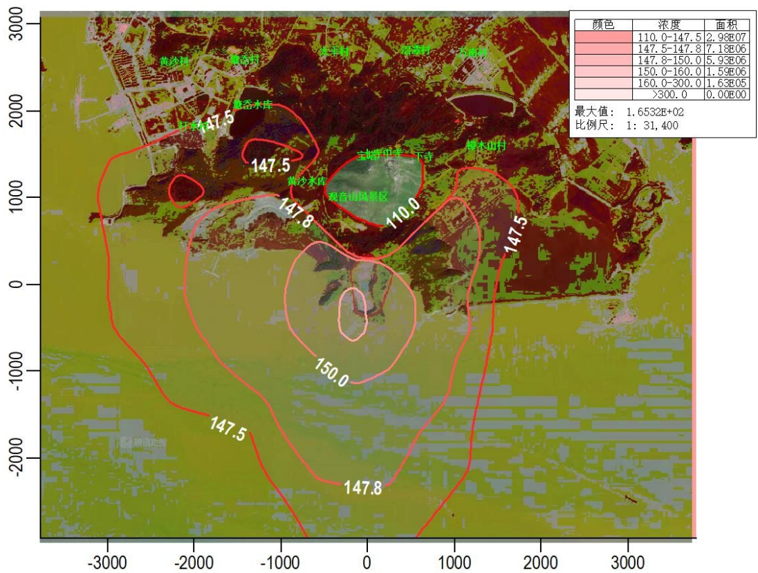
图4-4 正常工况下叠加背景值后保证率日平均浓度预测图
