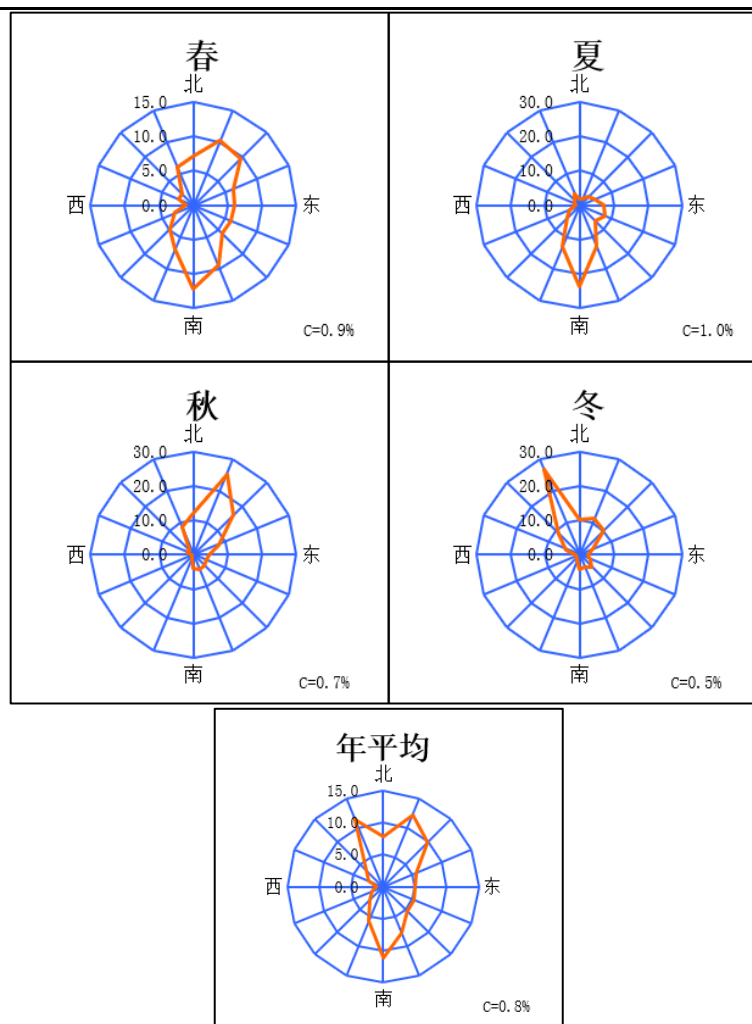
图4-4 风频玫瑰图
