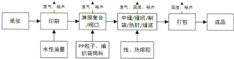
图 1-1 生产工艺流程和产污环节图
