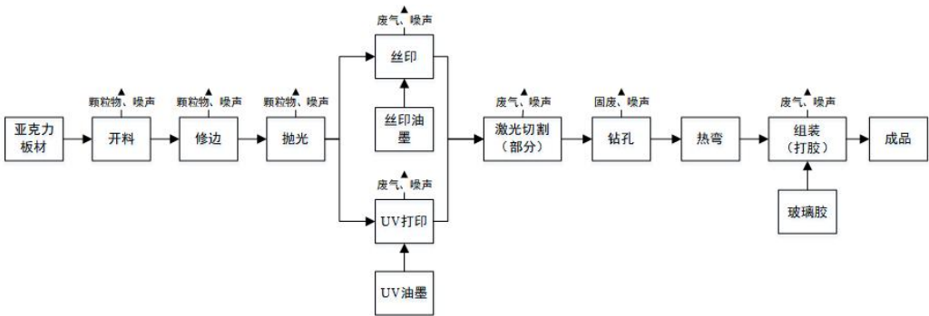
图 2-1 生产工艺流程和产污环节图
