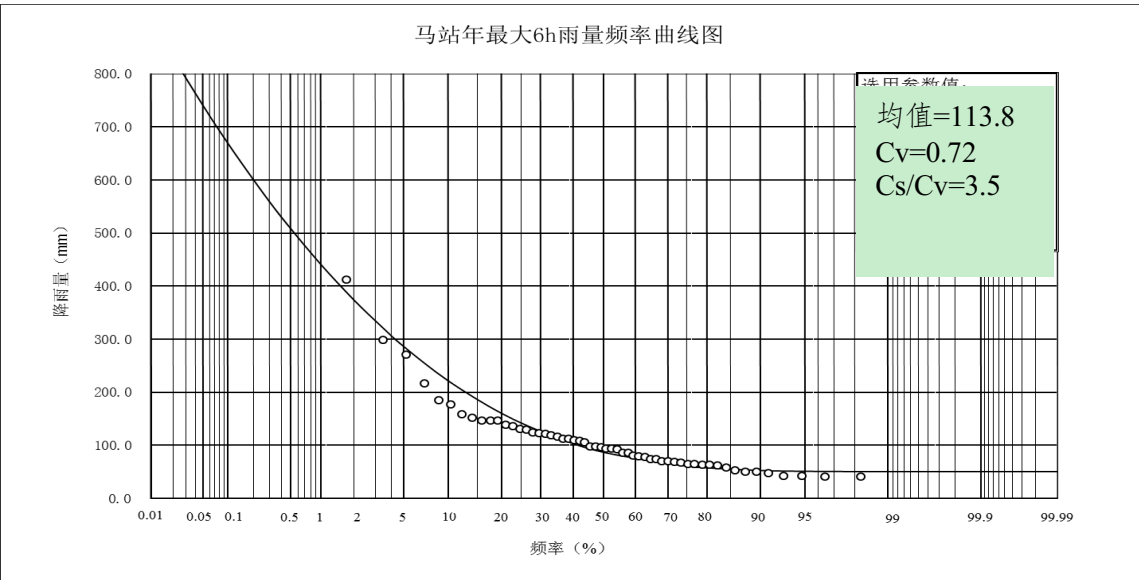
图 4.5-2 马站年最大 6h 降雨频率曲线图
