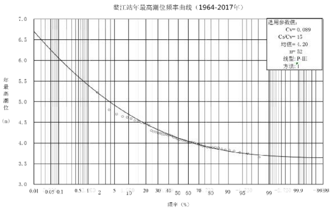
图 4.6-1 鳌江站年最高潮位频率曲线
