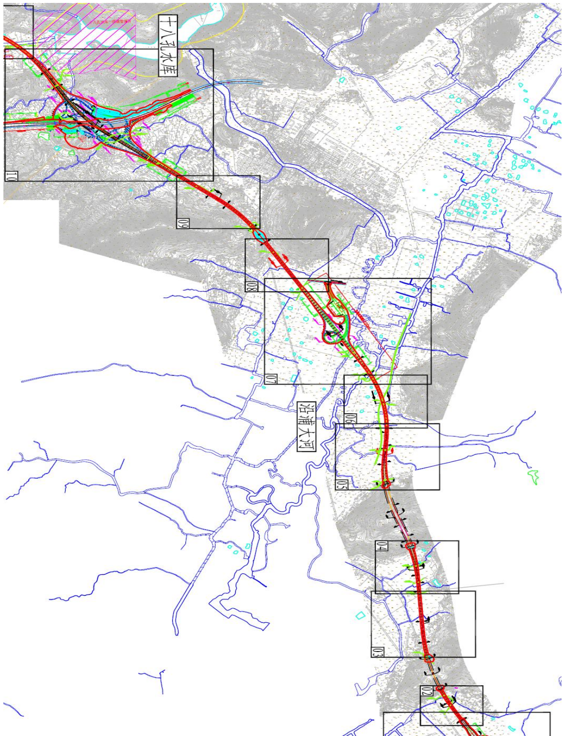
图 2.3-4 马站平原段工程平面布置图
