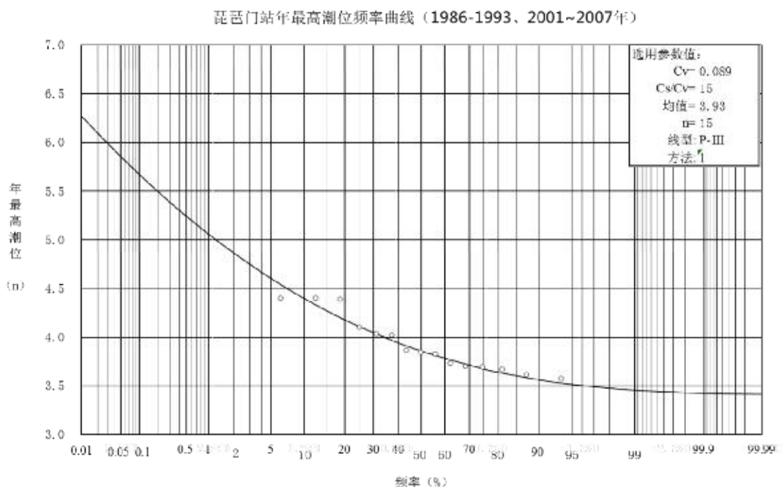
图 4.6-2 琵琶门站年最高潮位频率曲线图
