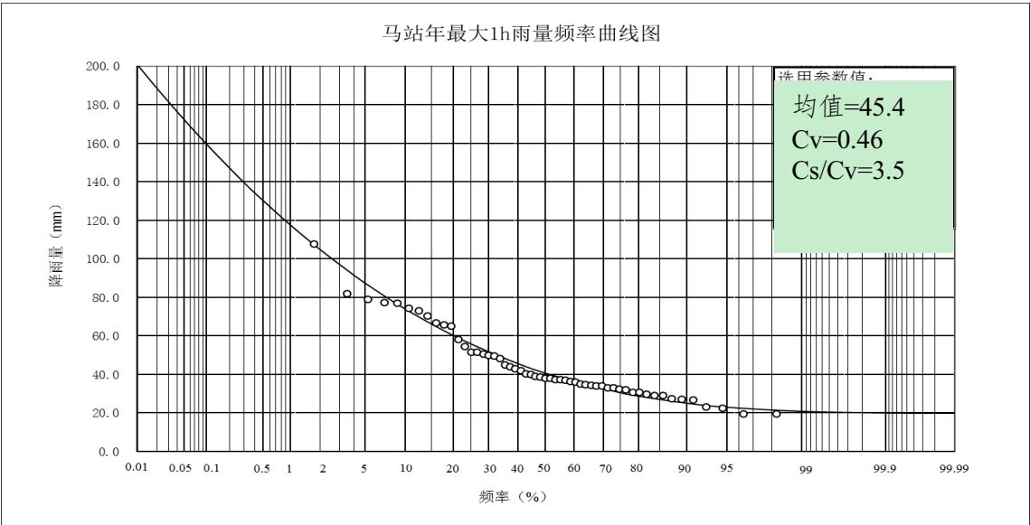
图 4.5-1 马站年最大 1h 降雨频率曲线图
