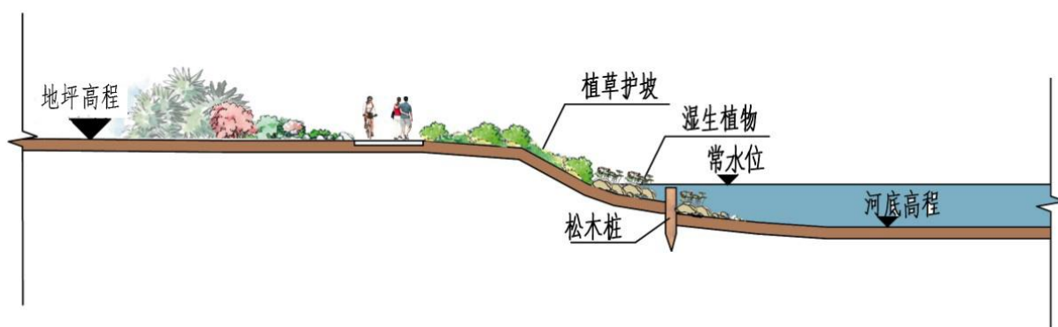
图 6.2-1 典型复式断面示意图
