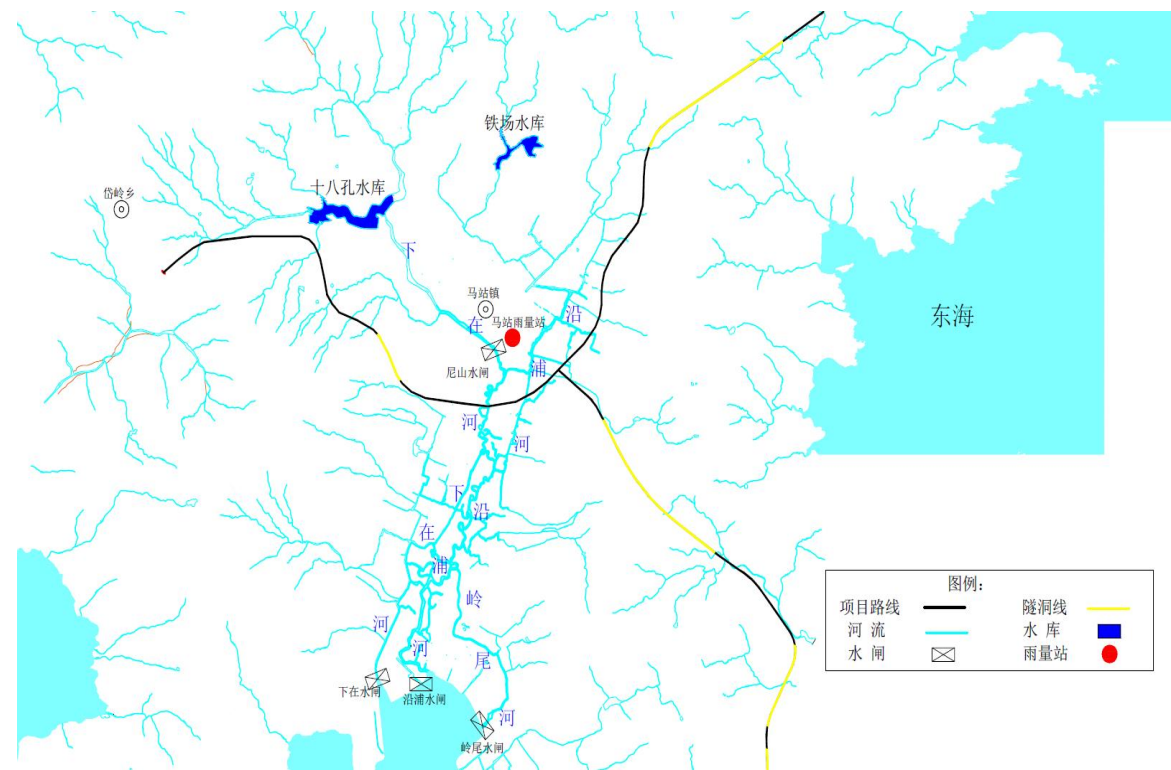
图 2.3-1 工程线位与马站平原位置图
