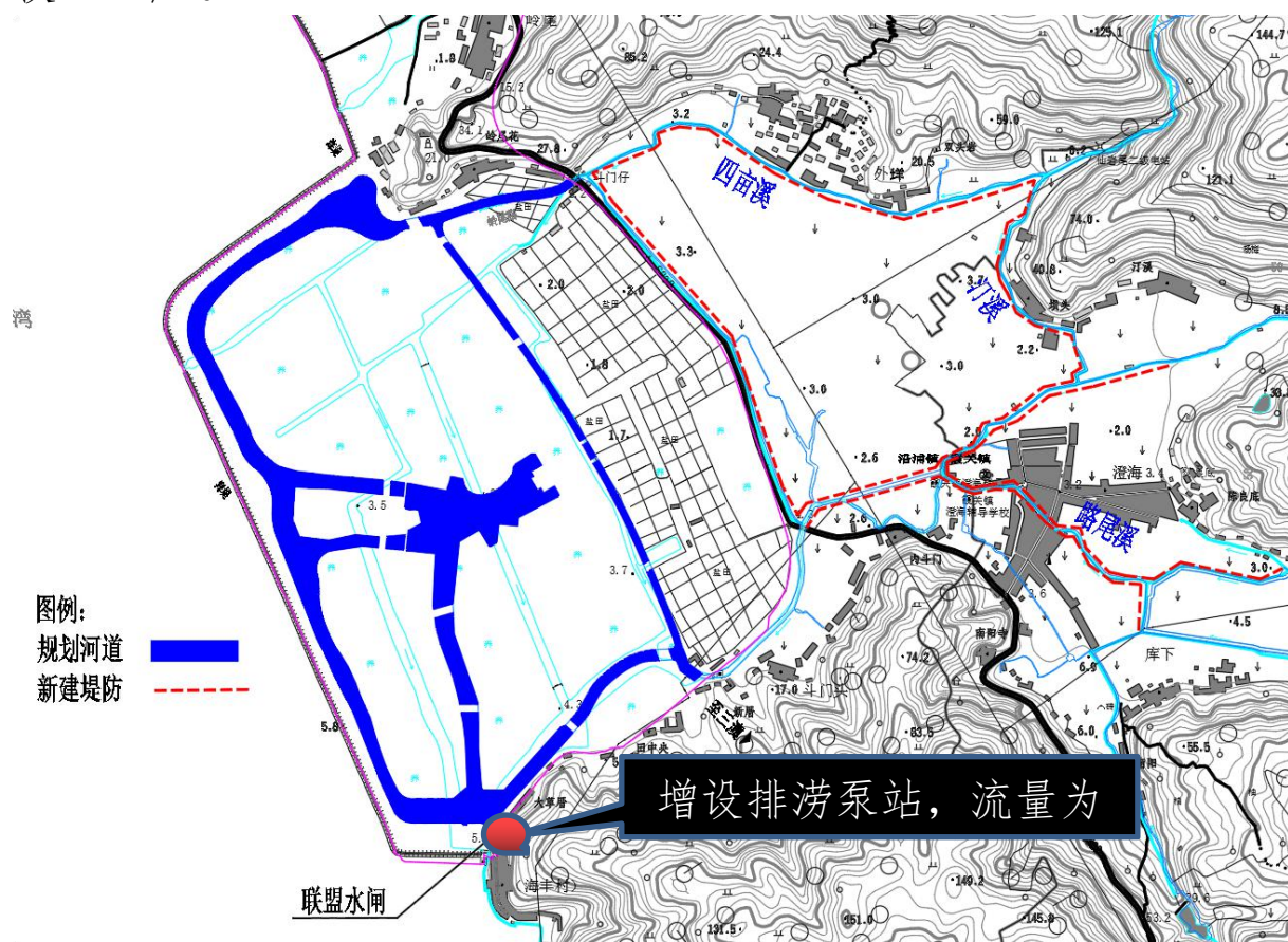
图 5.3-5 澄海小流域泵站位置示意图
