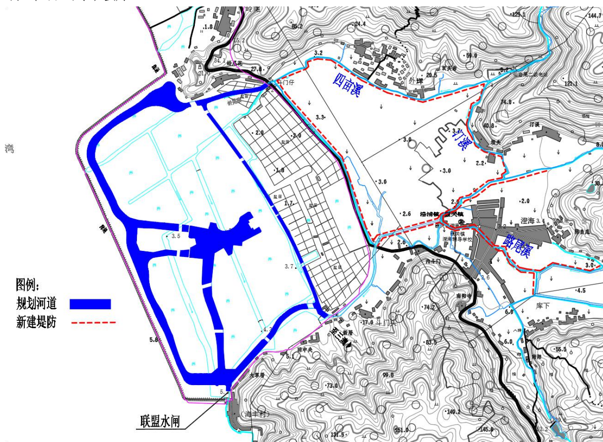
图 5.3-4 澄海小流域堤防建设方案示意图
