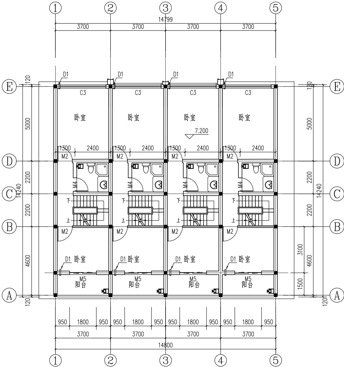
三层平面图 1:100
