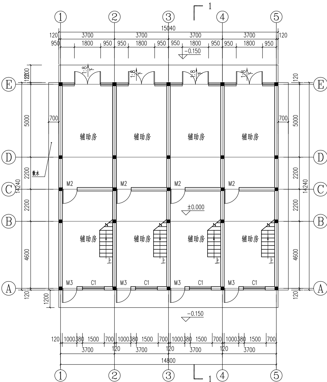
一层平面图 1:100
