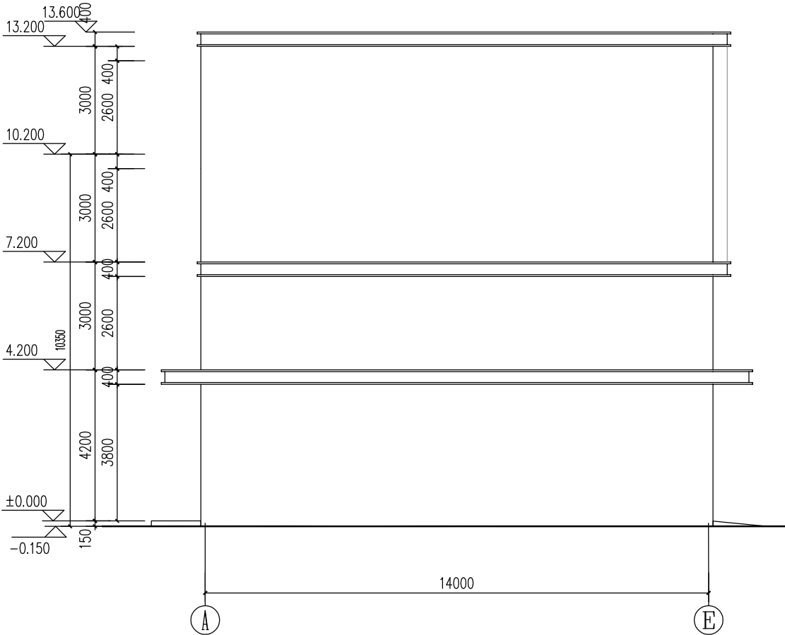
①—⑤轴立面图 1:100
