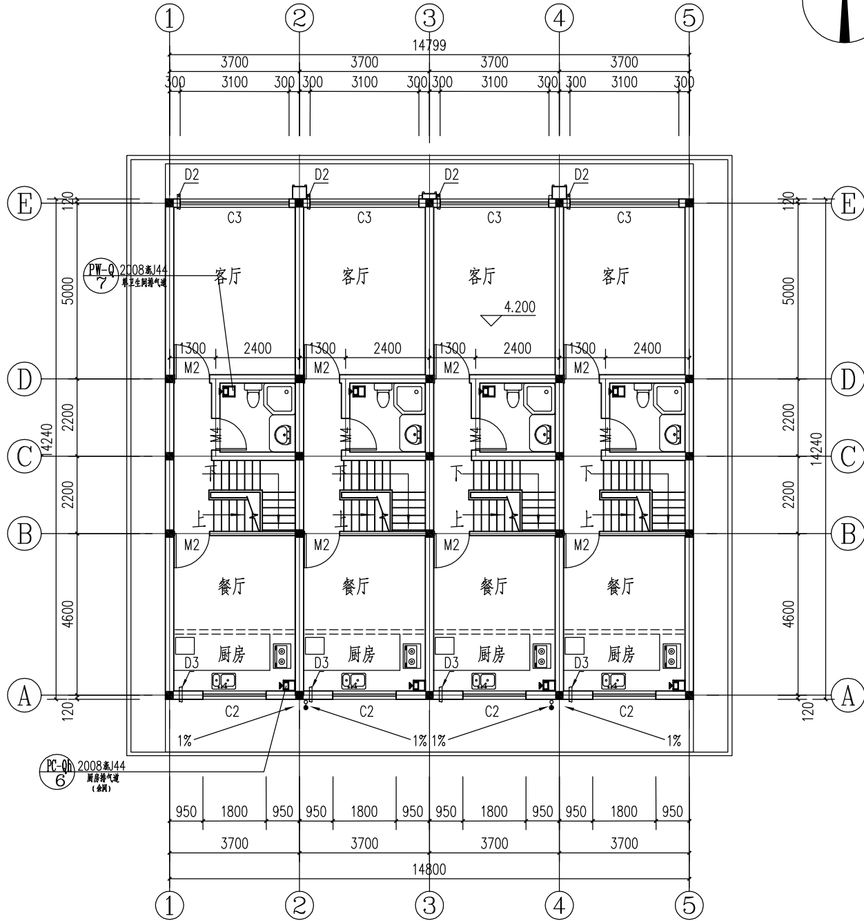
二层平面图 1:100
