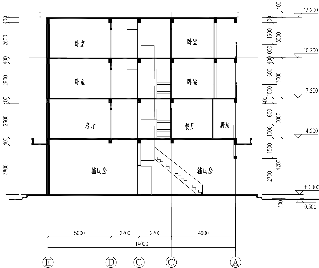
1-1剖面图 1:100
