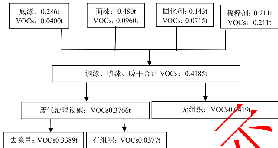
图 2-2 项目油漆有机溶剂平衡图
