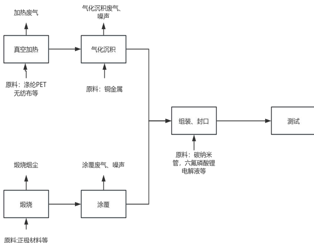
图 2-4 柔性电池研发流程示意图
