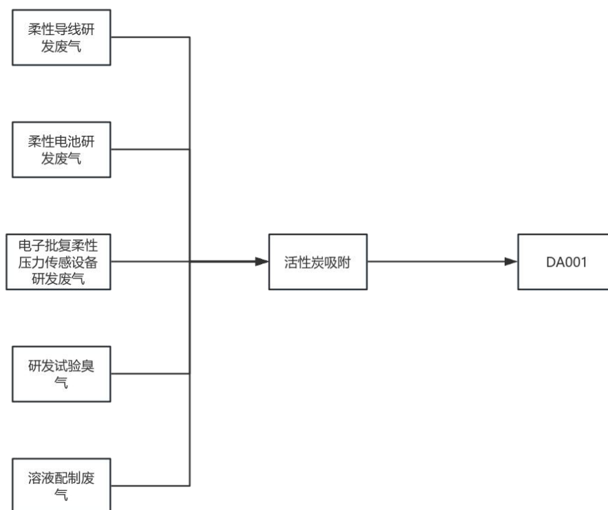
图 2-2 废气处理流程图
