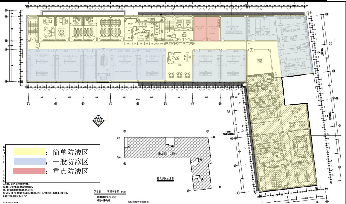
图 4-1 分区防渗图
