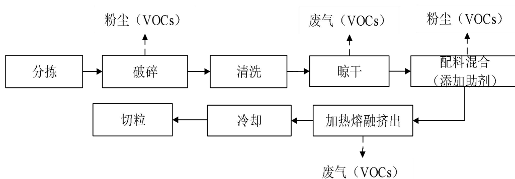
图 A.2 回料造粒工艺流程及产排污节点
