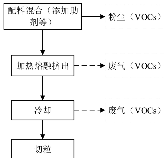
图 A.1 新料造粒工艺流程及产排污节点
