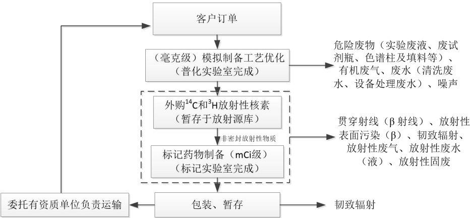
图 9.2-2 项目总体工艺流程及产污环节图
