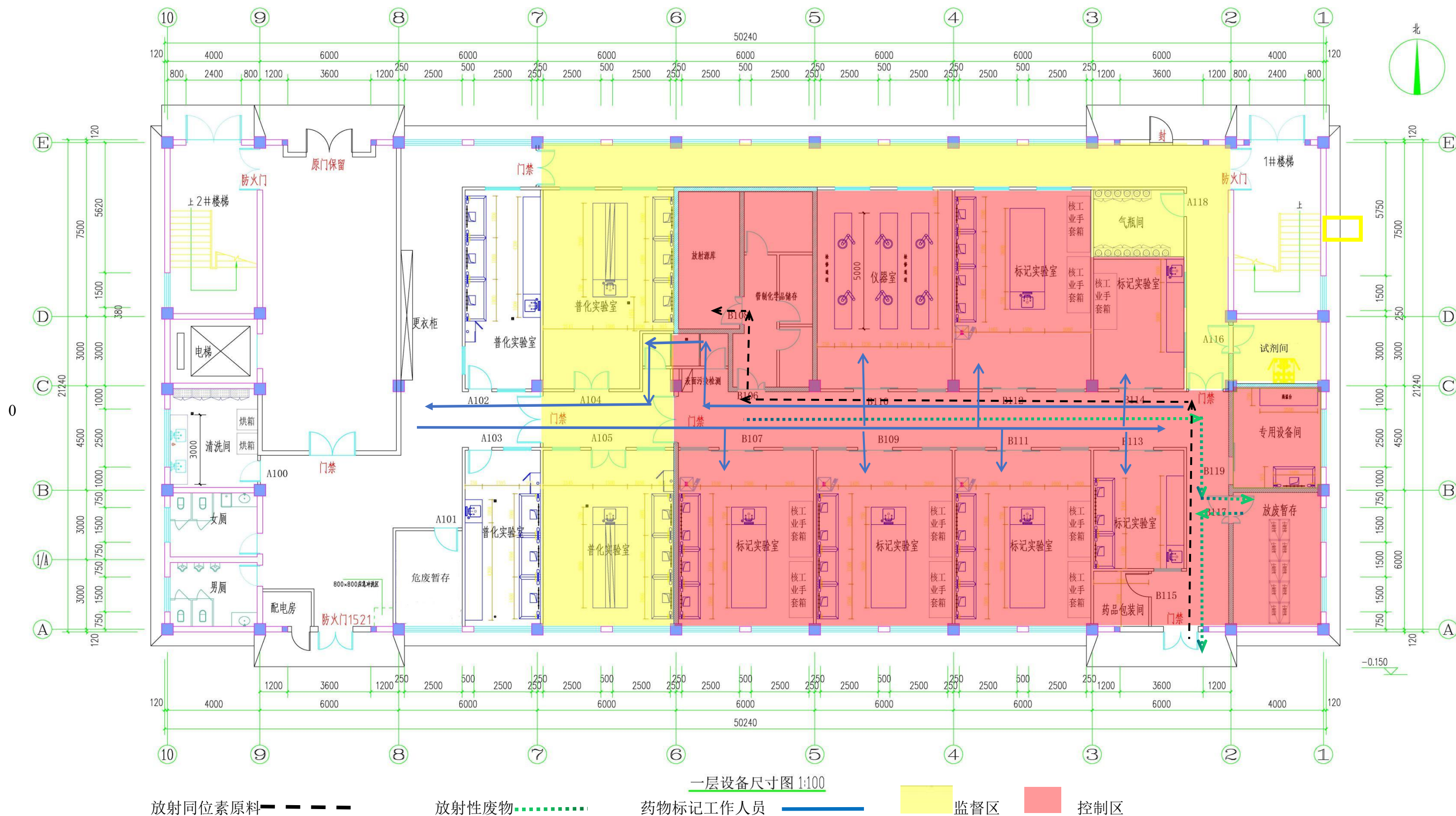
附图 4 项目平面布局及两区划分图（单位：mm）
