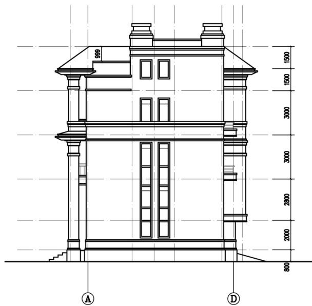
①—⑮轴立面图 1:100
