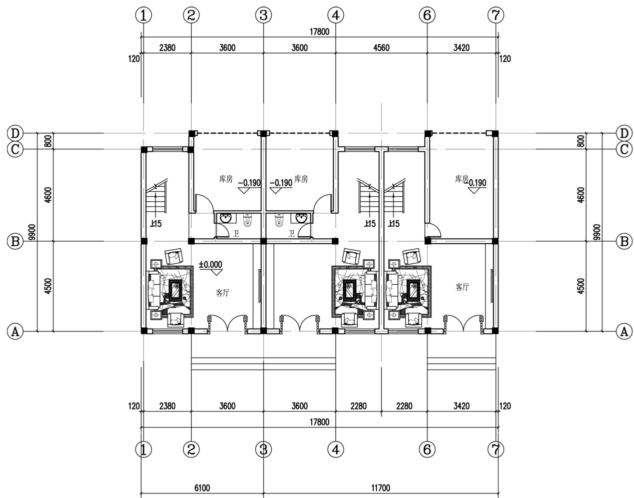
一层平面图 1:100
