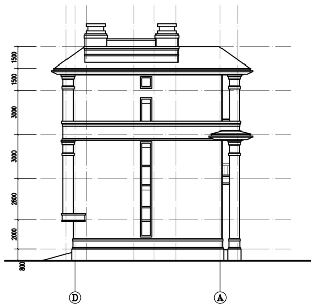
⑮—①轴立面图 1:100
