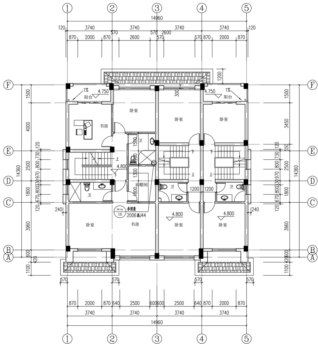
二层平面 1:100
