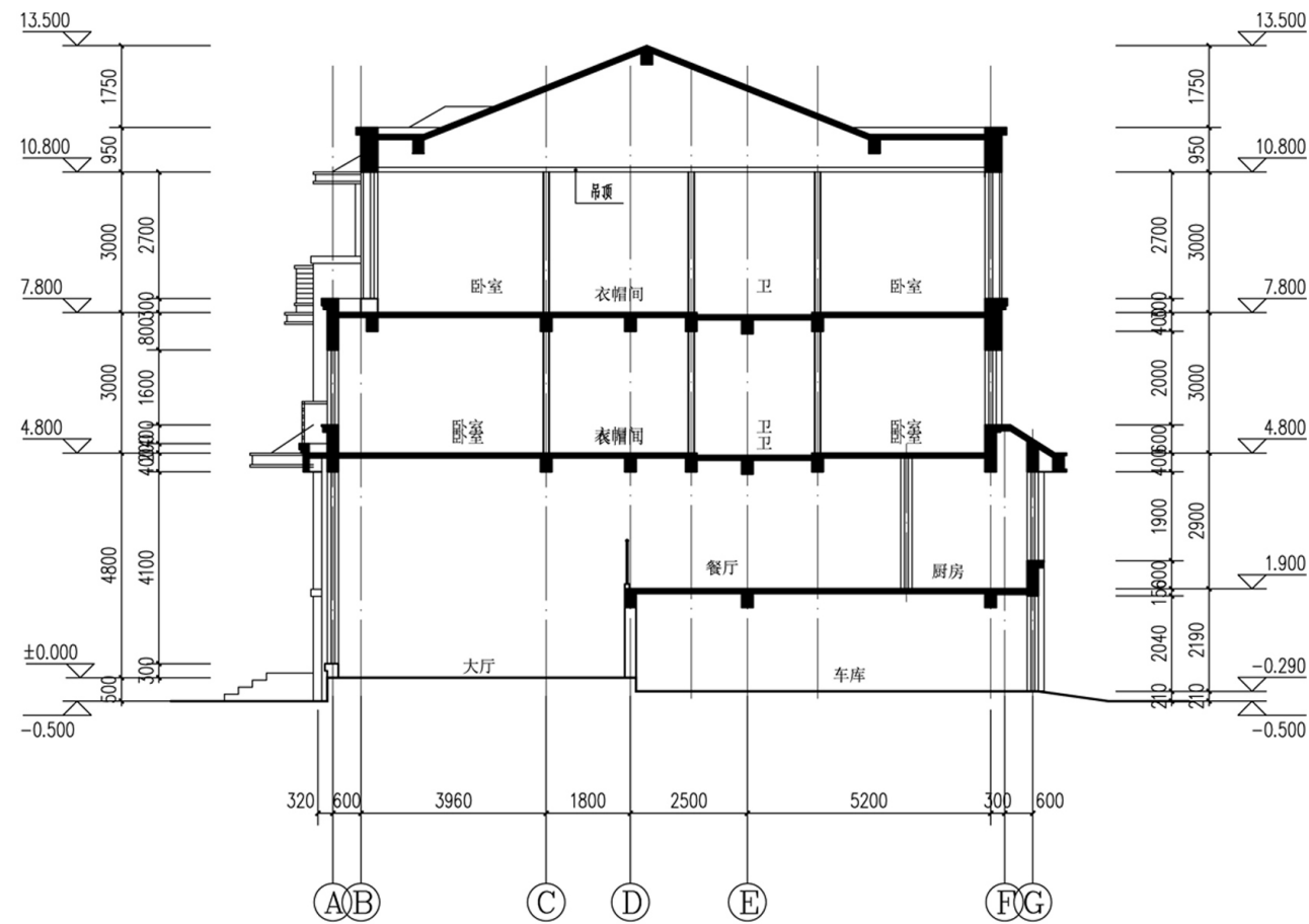
1-1剖面 1:100
