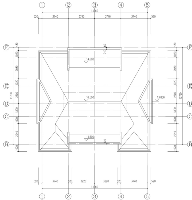
屋顶平面 1:100
