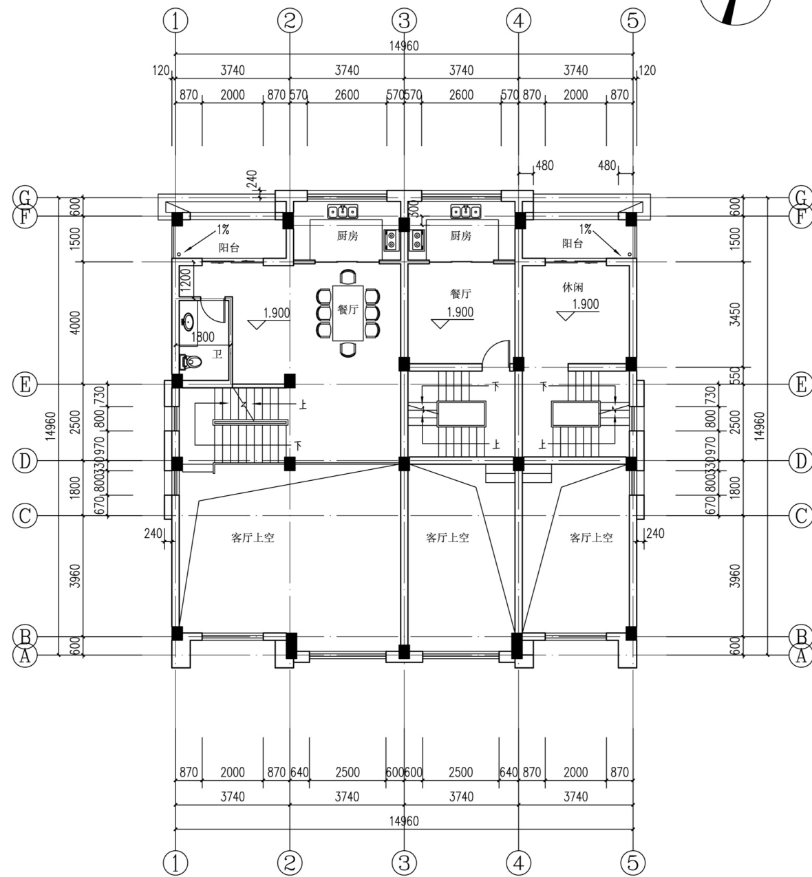
夹层平面 1:100
