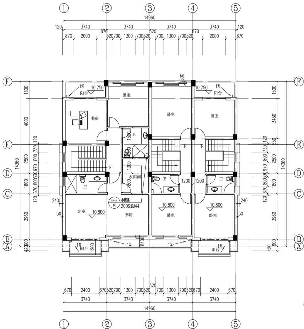
三层平面 1:100
