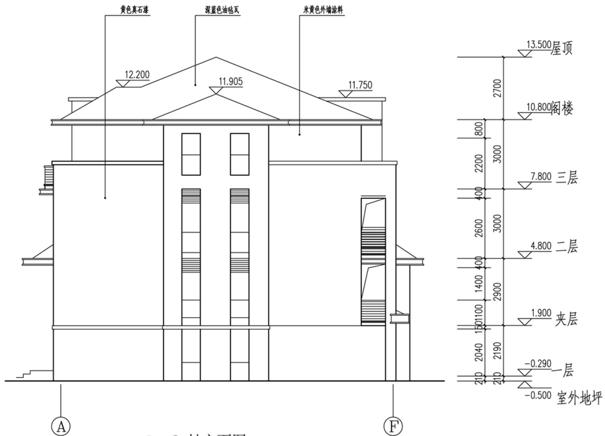
①-⑥ 轴立面图 1:100
