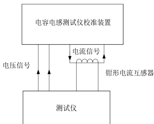
图 2 电容量、电感量校准接线图
