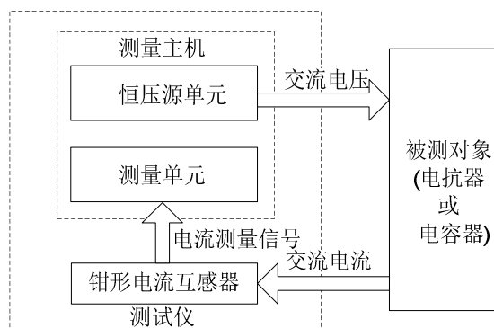
图 1 测试仪工作原理图
