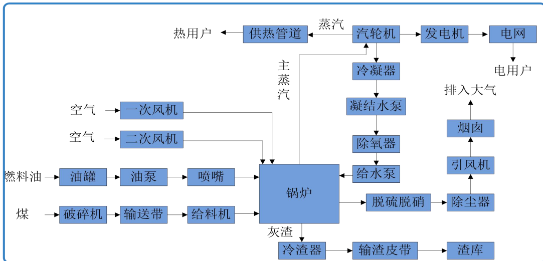
图 2 抽凝发电机组工艺路线图
