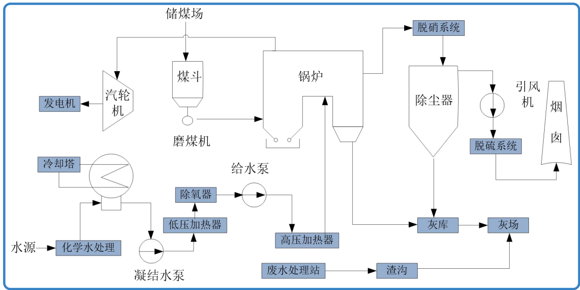
图 1 常规燃煤发电机组工艺路线图
