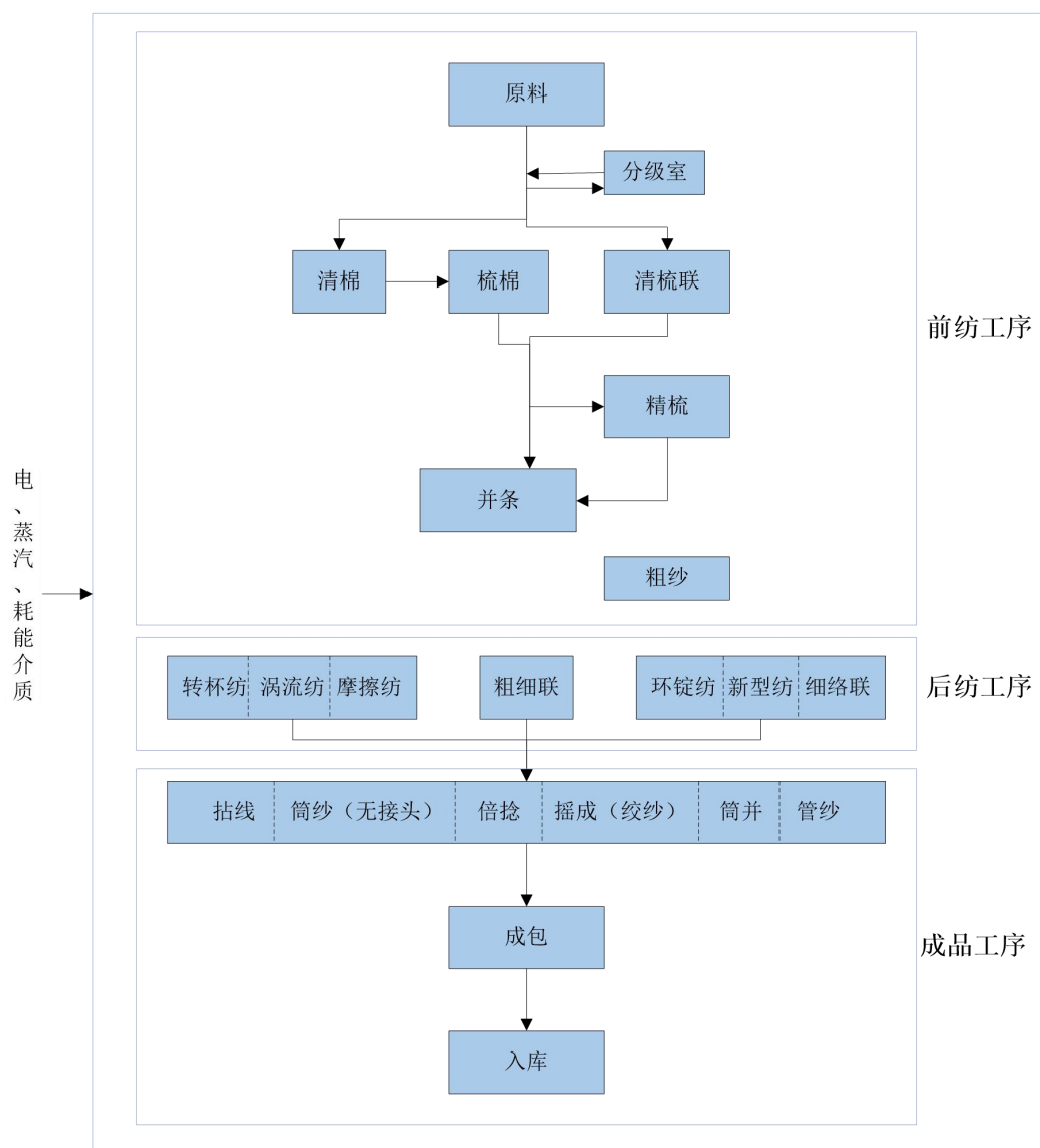
图 1 纺纱（棉、化纤及混纺）生产工艺流程图
