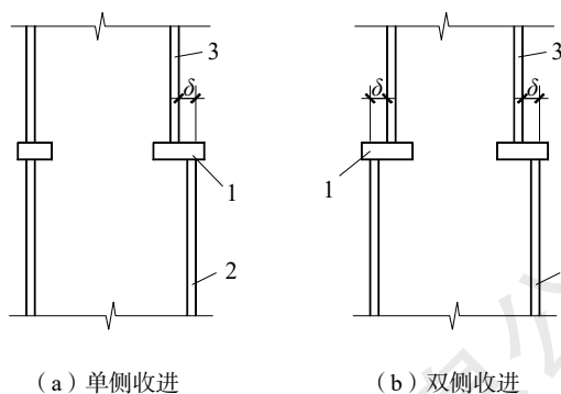
图 7.2.2-1 桁架加劲多腔体变厚度连接节点示意图
