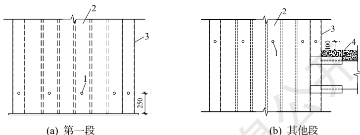
图 9.2.4 桁架加劲多腔体排气孔位置示意图
