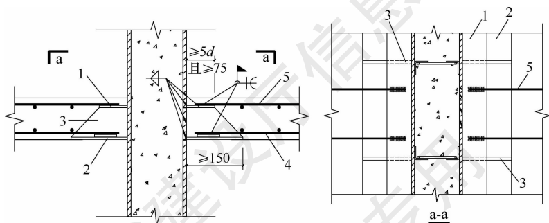
图 7.6.4 组合剪力墙与楼板预留钢板连接节点示意图
