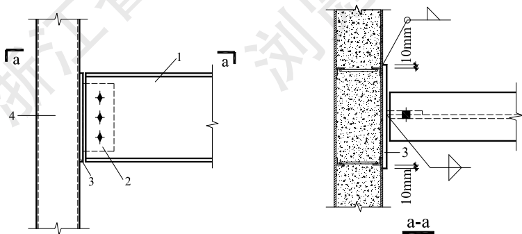
图 7.4.6 铰接连接节点示意图
