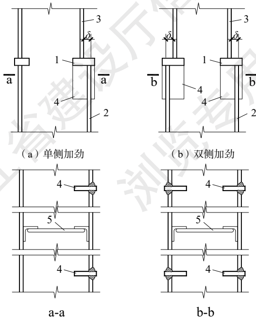
图 7.2.2-2 桁架加劲多腔体变厚度加劲连接节点示意图
