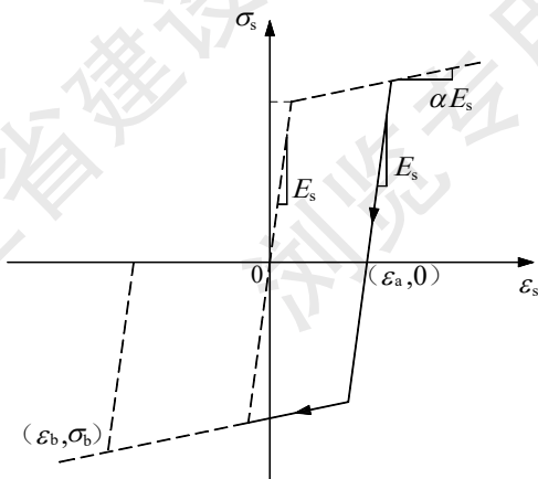
图 B.1.2 钢材反复加载应力—应变曲线
