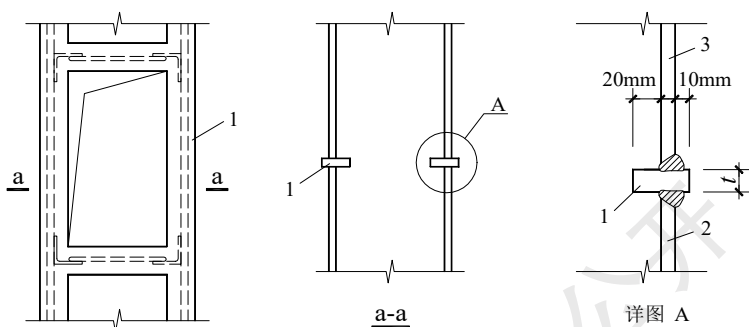
图 7.2.1 桁架加劲多腔体连接节点示意图
