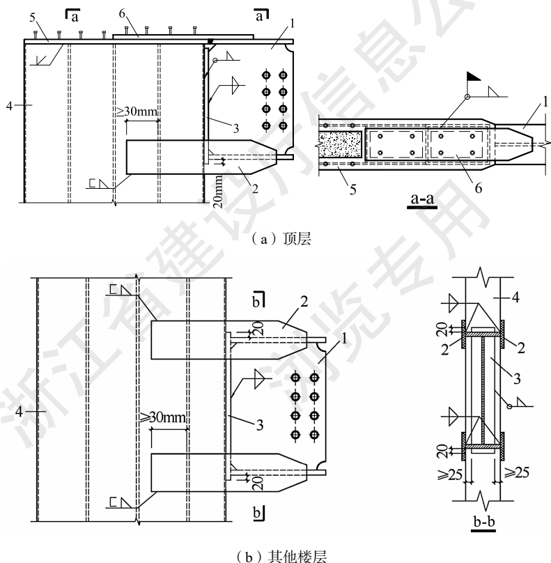
图 7.4.2 刚性连接节点示意图
