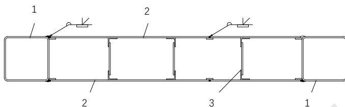
图 6.3.5 桁架加劲多腔体焊缝示意图
