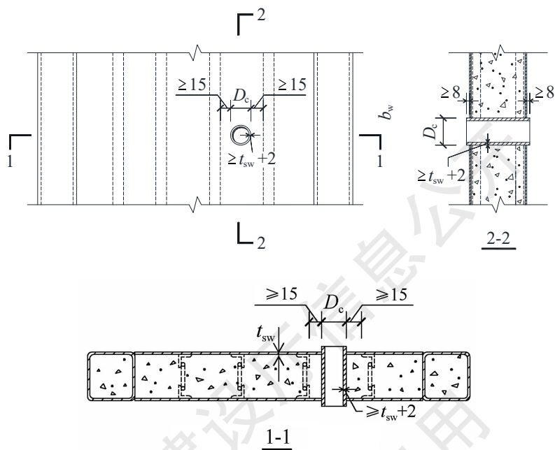
图 7.6.5 墙体开孔套管补强方式示意图
