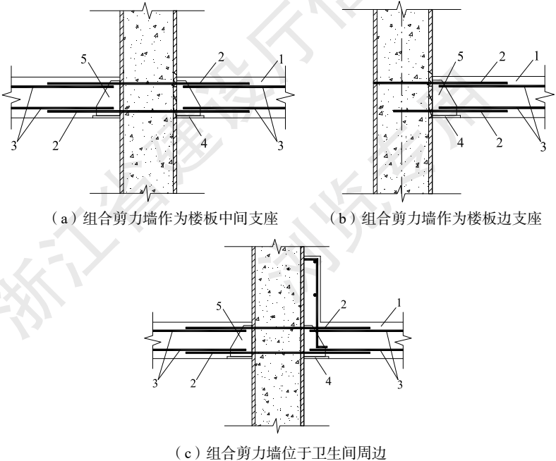
图 7.5.3 组合剪力墙与楼板预留钢筋连接节点示意图
