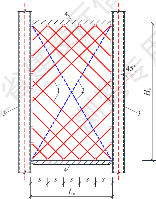
图 A.0.1 组合剪力墙等效杆系模型示意图
