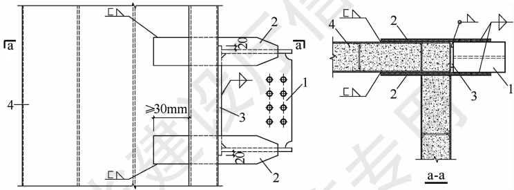
图 7.4.7 L形或Z形组合剪力墙转角处一侧与钢梁刚性连接节点示意图
