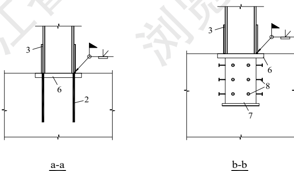
图 7.3.1 桁架加劲多腔体钢板组合剪力墙墙脚节点示意图
