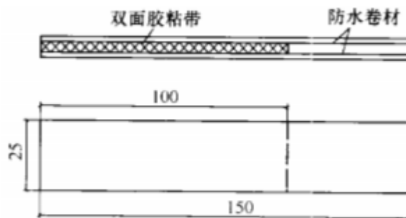
图 D.3.1 双面胶粘带剥离强度试样
