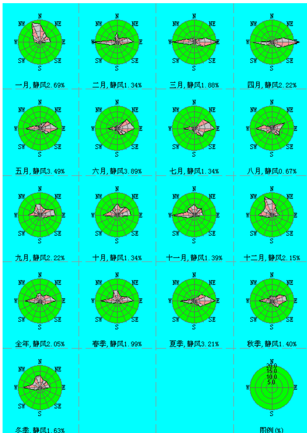
图 6.2-4 气象统计风玫瑰图
