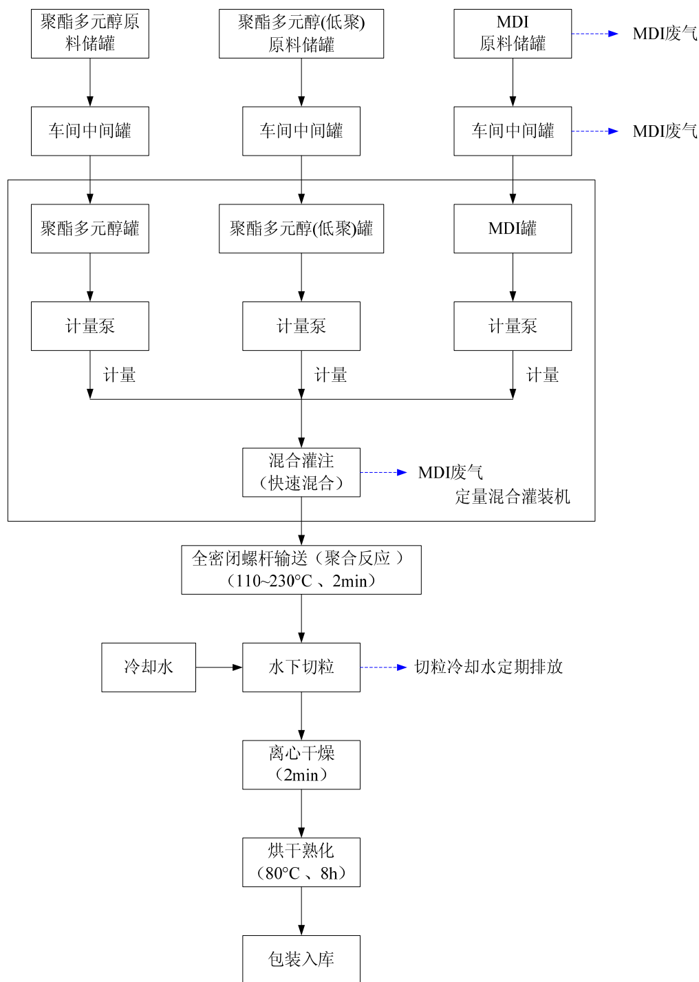
图 3.2-1 现有 TPU 生产工艺流程图
