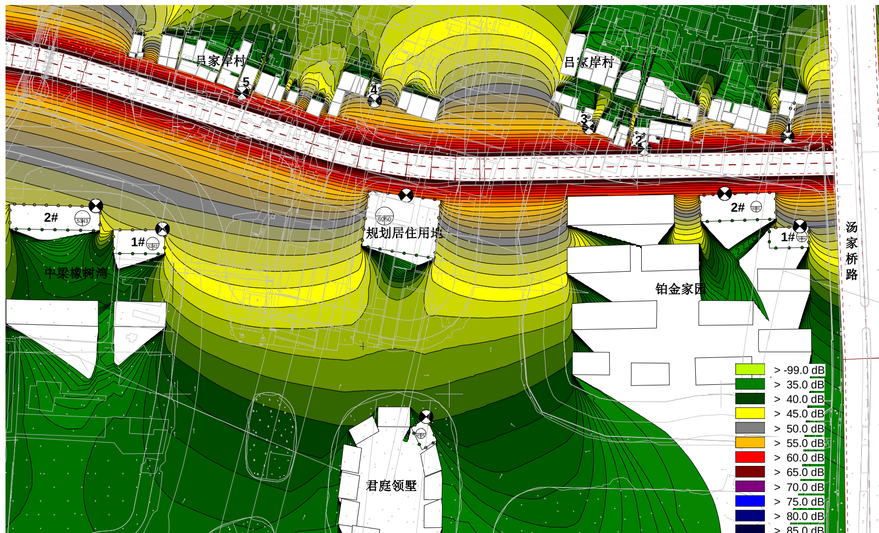
图 6.3-1 营运远期昼间等声级线图（2030 年）
