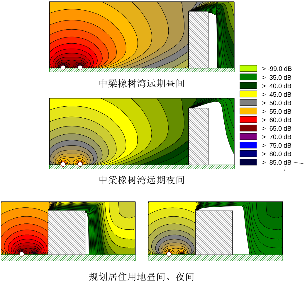
图 6.3-8 营运远期剖面等声级线图
