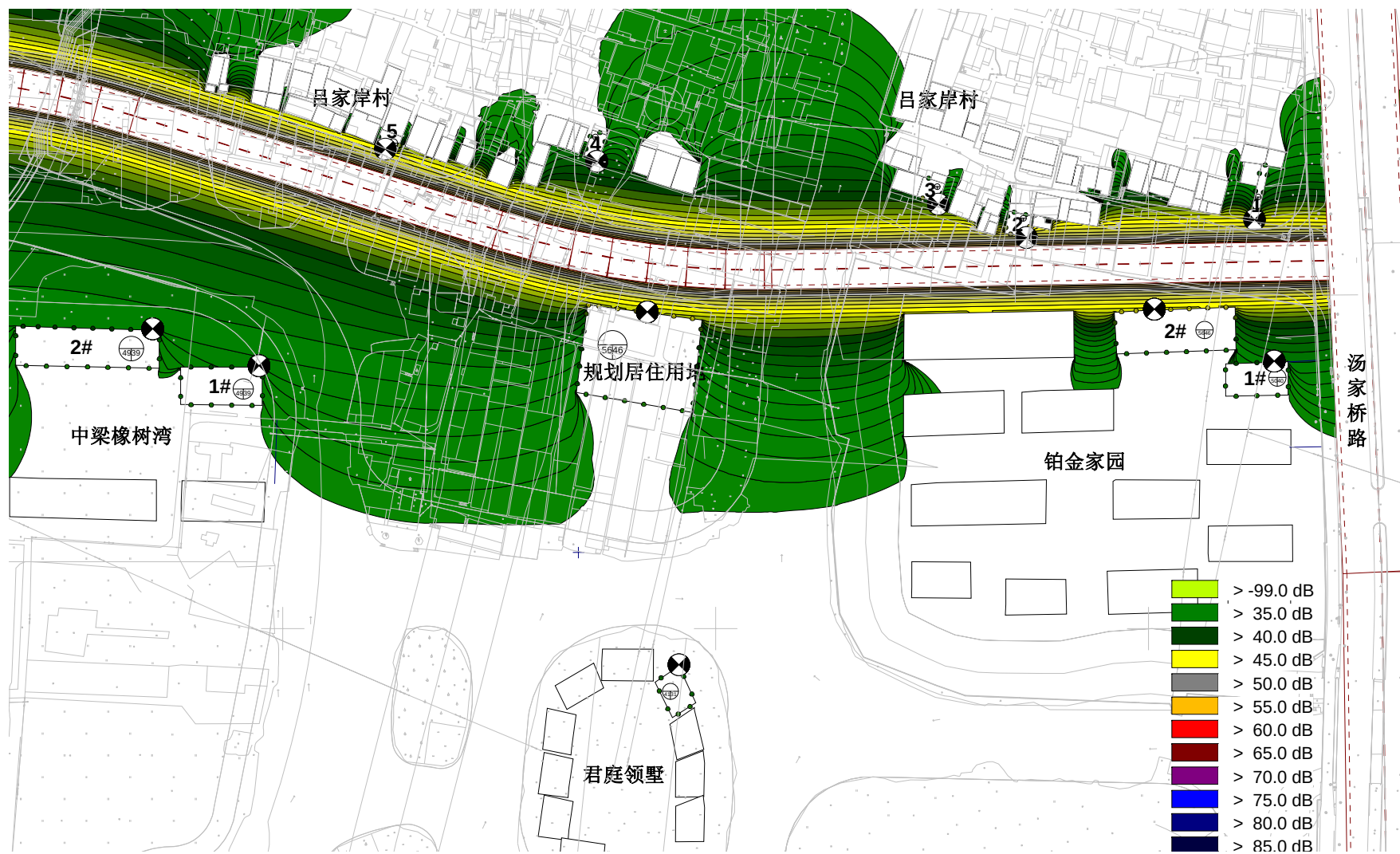
图 6.3-2 营运近期夜间等声级线图（2016 年）
