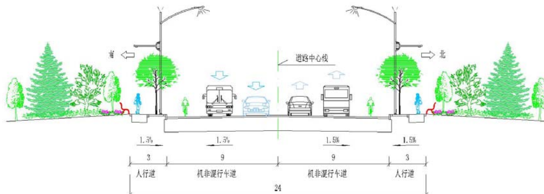
东垟路标准横断面
