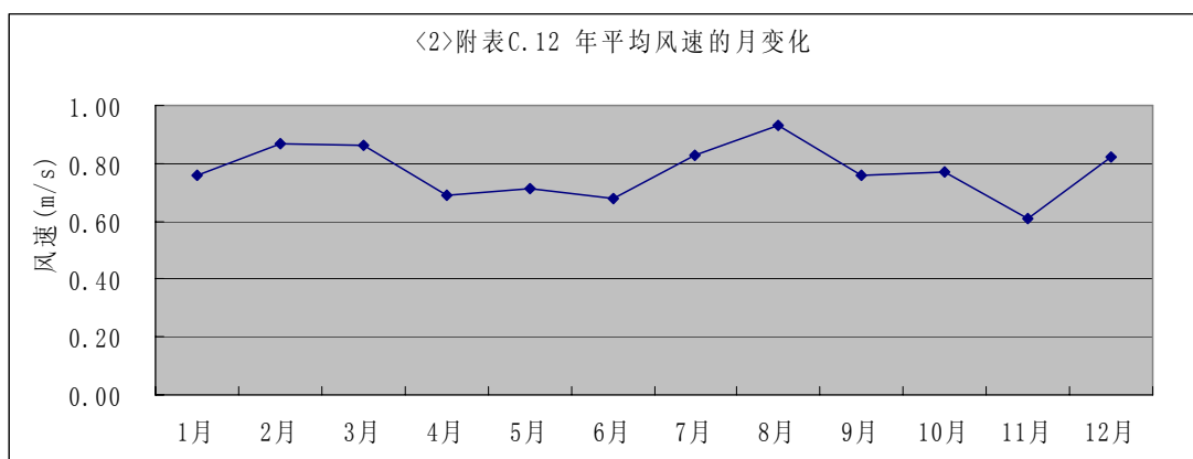
图 5.2-2 年平均风速的月变化曲线图
