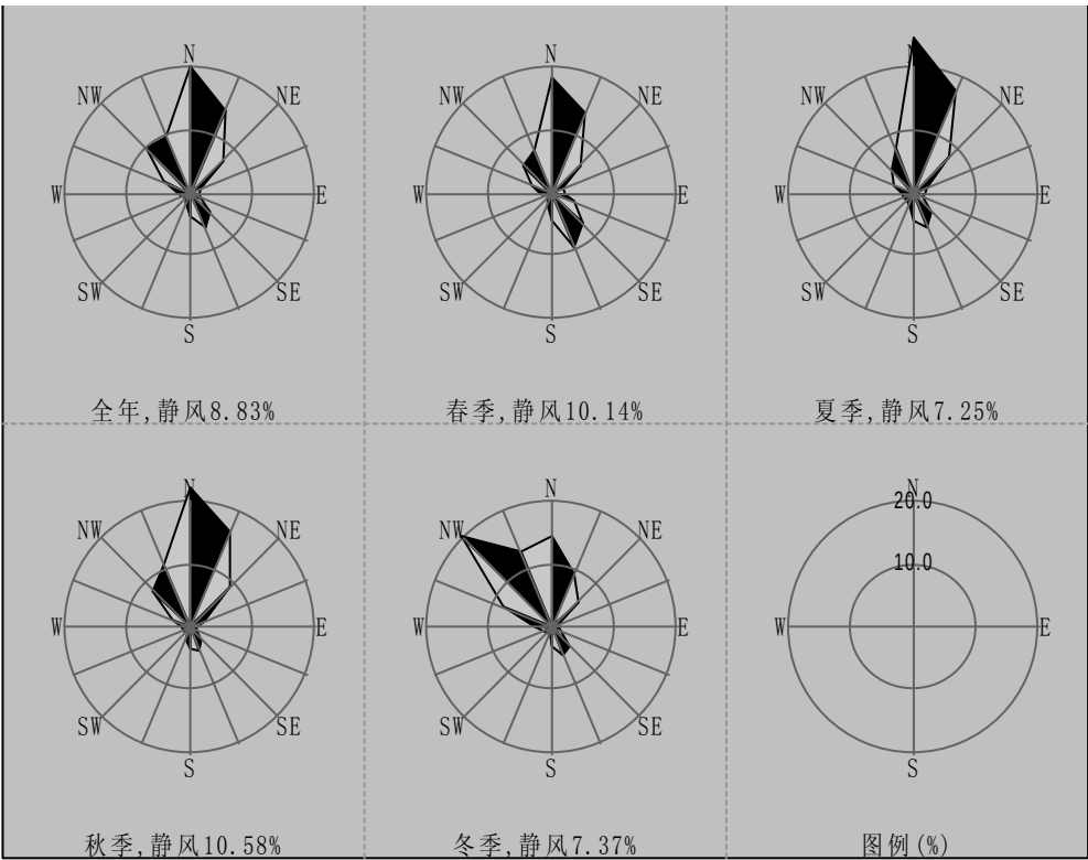
图 5.2-4 各季及年平均风向玫瑰图
