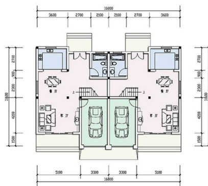
一层平面图 占地面积: 98.1M 2 /户 建筑面积: 250.3M 2 /户
