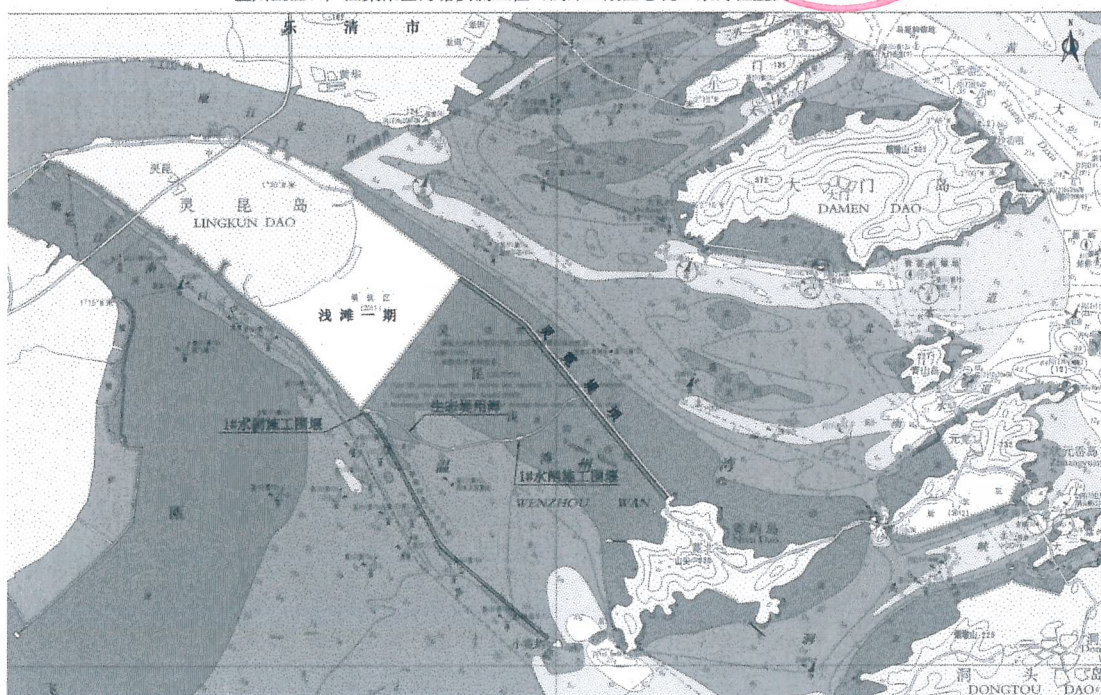
温州瓯江口产业集聚区海塘安澜工程（浅滩二期生态堤）宗海位置图
